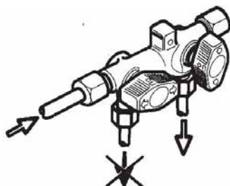
Fig. 79: Position marche/arrêt
