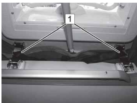
Fig. 197: Fermetures de toit (1)
