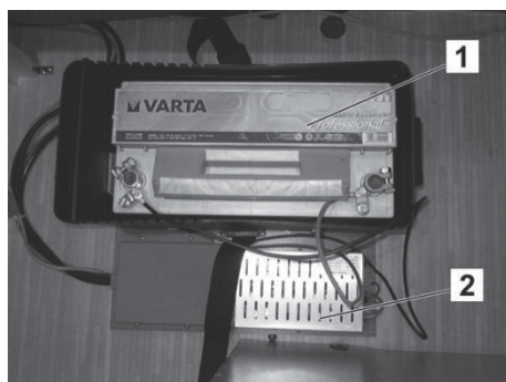
Fig. 64 : Pack Liberty
