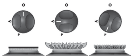
Fig. 209 : Positions des boutons : ARRÊT, grande flamme, petite flamme
