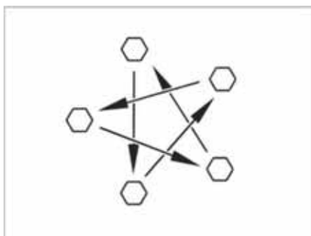
Fig. 220: Serrer en croix les écrous de roues ou vis de roues
