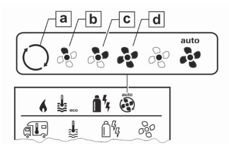
Fig. 147 : Symbole du niveau de ventilateur
