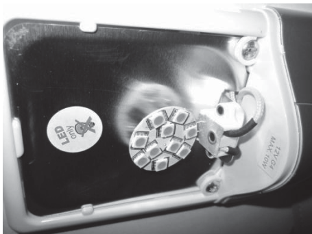
Fig. 225: Remplacement de l'ampoule LED
