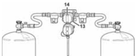
Fig. 120 : Kit détendeur
