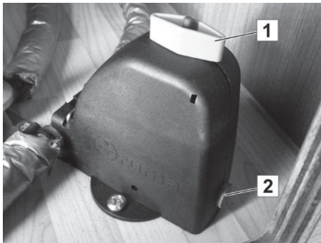
Fig. 109 : Vanne de vidange de sécurité ouverte
