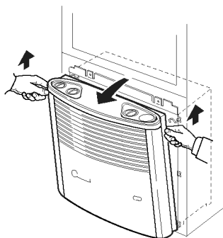
Fig. 125: Ouvrir l'habillage du chauffage
