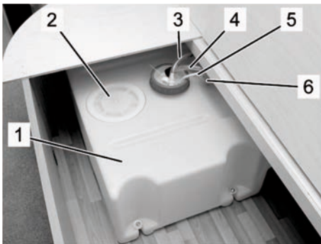
Fig. 88: Exemple de réservoir d'eau fraîche
