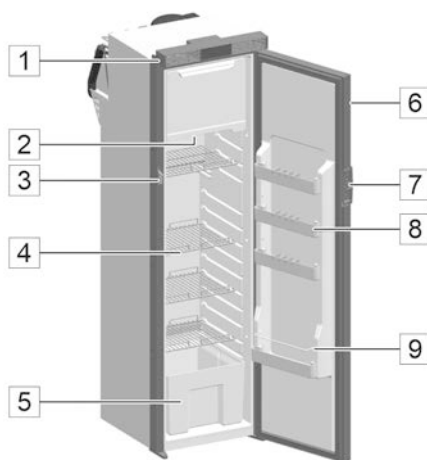
Fig. 154 : Réfrigérateur à compression 12 V
