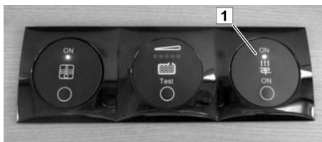
Fig. 86 : Boutons Marche/Arrêt du chauffage au sol
