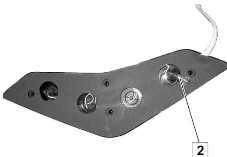
Fig. 168 : Remplacement de l'ampoule
