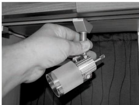
Fig. 140 : déplacer les spots LED
