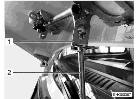
Afb. 36 Steun motorkap
