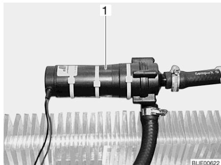
Afb. 128 Extra circulatiepomp
