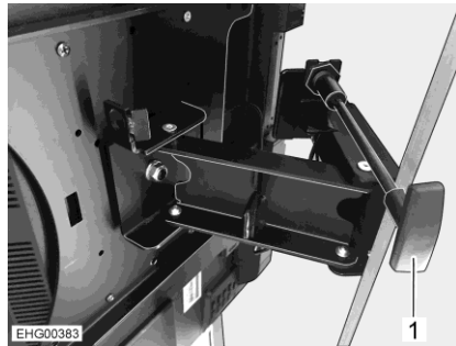
Afb. 76 Houder (eendelige scharnierarm)
