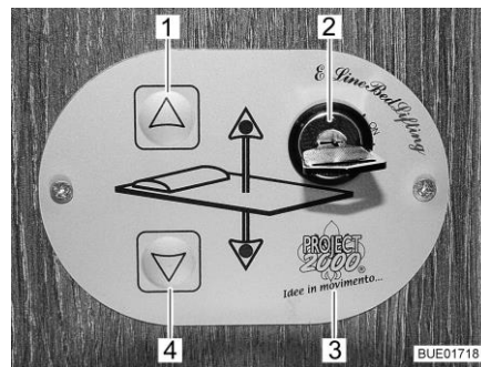
Afb. 96 Bedieningsgedeelte
