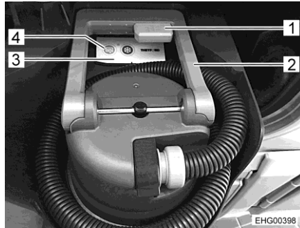
Afb. 150 Legingsmodule
