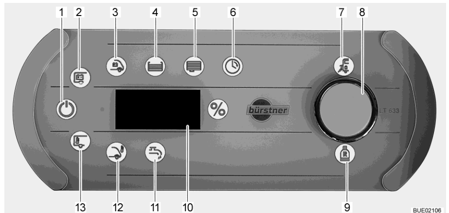
Afb. 109 Paneel LT 633
