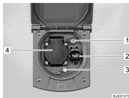
Afb. 116 Buitencontactdoos
