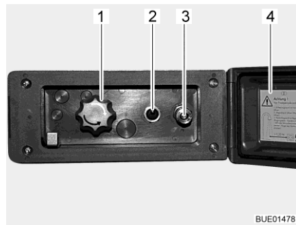
Afb. 98 Doucheaansluiting buiten
