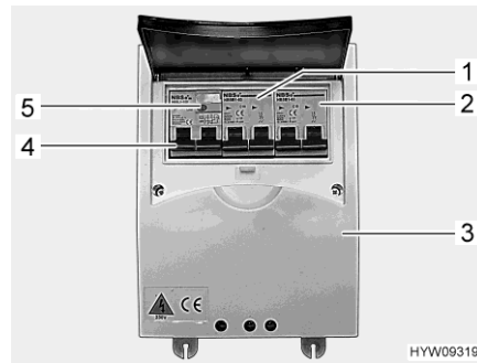
Afb. 110 Beveiligingsautomaat en FI-schakelaar (230-V-zekeringenkast)
