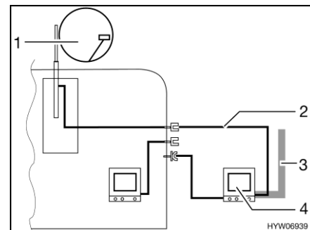
Afb. 118 TV in de voortent
