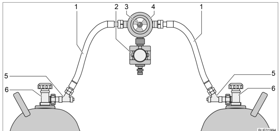
Afb. 11 Gasdrukregelaar met CPU en slangbreukbeveiliging
