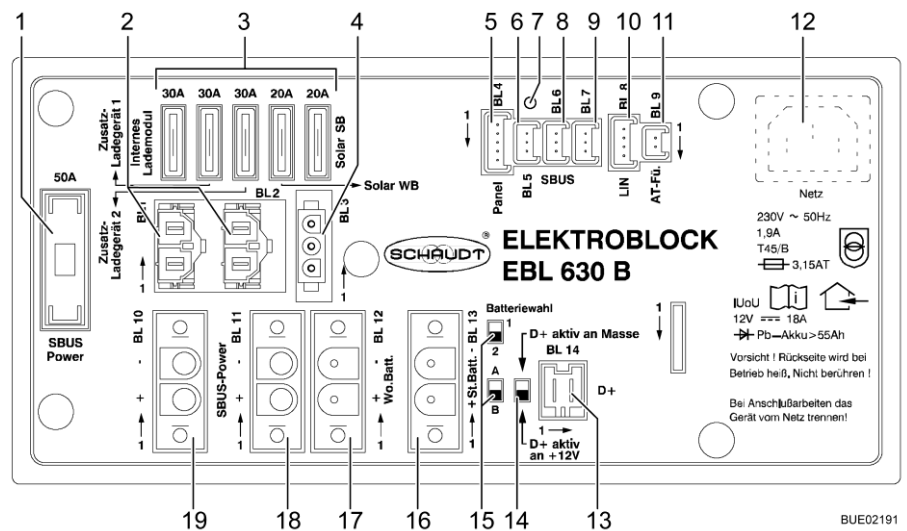
Afb. 108 Elektroblok (EBL 630)
