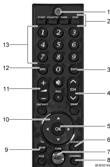
Afb. 45 Afstandsbediening
