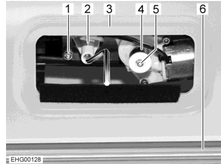
Afb. 34 Toegang tot de motor
