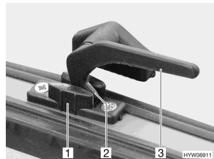
Afb. 83 Vergrendelingshendel in stand "vast afgesloten"
