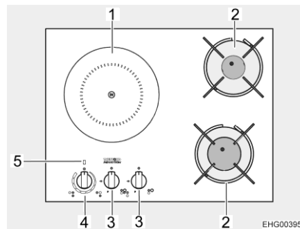
Afb. 139 Hybride kookveld
