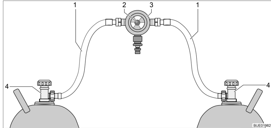
Afb. 102 Omschakelinstallatie voor gasflessen
