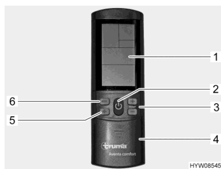
Afb. 134 Afstandsbediening (klimaatregeling)
