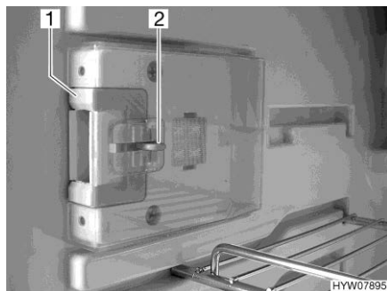
Billede 163 Låseanordning (normal- stilling)
