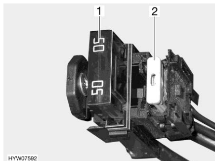
Billede 126 Sikringer på opholdsrummets batteri
