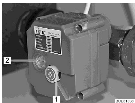
Billede 172 Elektrisk aftapningshane
