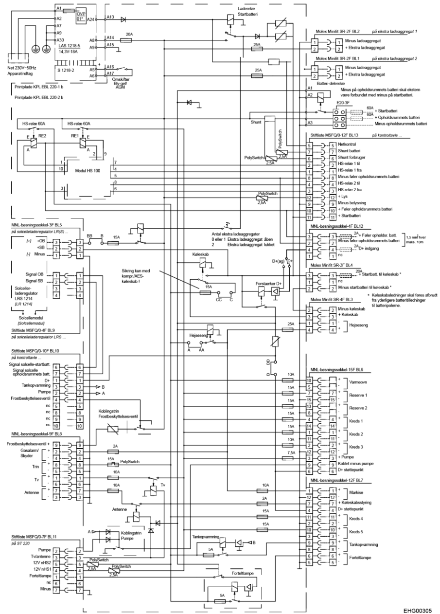
Billede 133 Strømdiagram indvendig (EBL 223)
