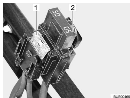
Billede 125 Sikringer på startbatteriet
