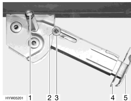
Billede 26 Hejsestøtte
