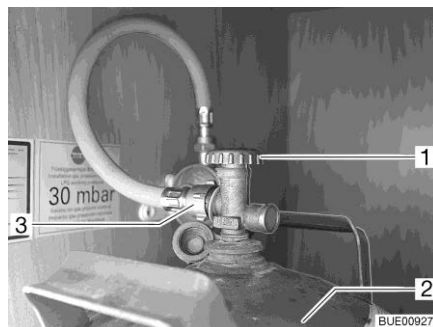
Billede 115 Gaskasse
