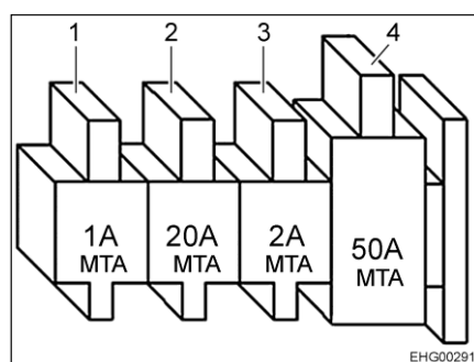
Billede 127 Sikringer (opholdsrummets batteri med ladebooster)
