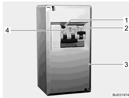
Billede 122 230 V-sikringskabinet med sikkerhedsafbryder og HFI-afbrydere
