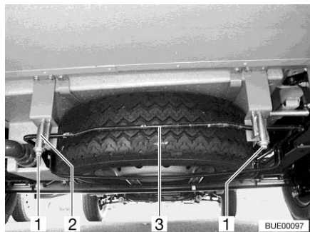
Billede 202 Reservehjulholder (ophæng)
