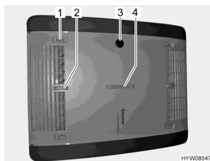
Billede 150 Funktionsdisplay og luftfordeling (klimaanlæg)
