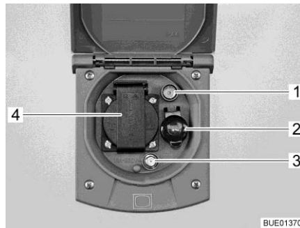
Billede 130 Udvendig stikdåse
