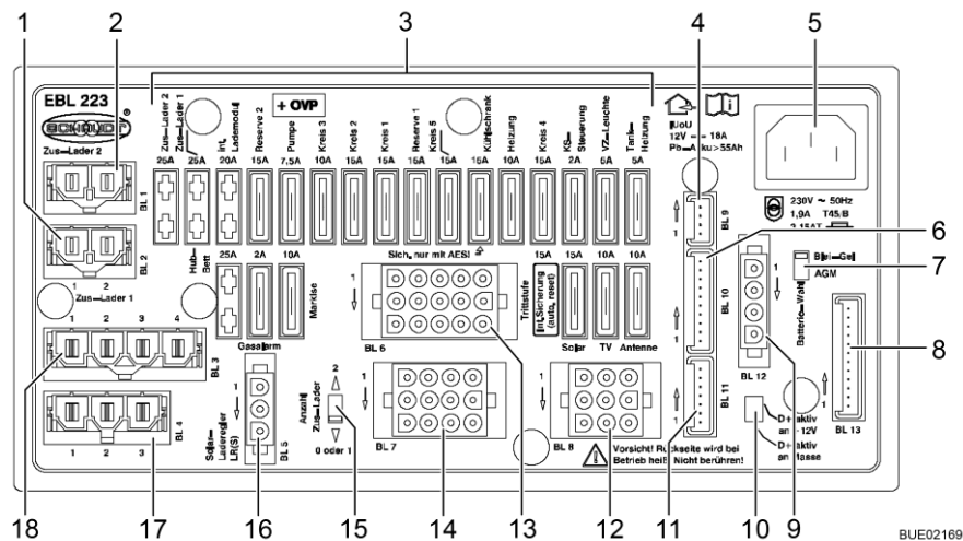
Billede 119 EL-blok (EBL 223)
