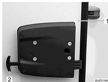
Billede 40 Nødåbning garageklap
