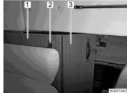
Billede 53 Skillevæg til førerkabinen
