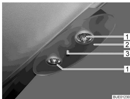
Billede 191 Halogenloftslampe
