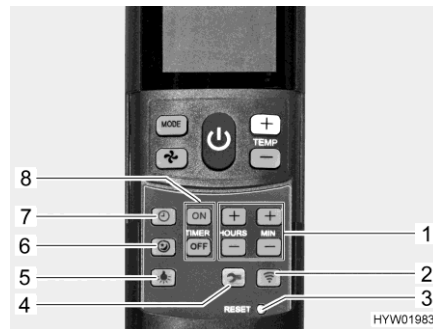
Billede 151 Fjernbetjening med indstillingsknapper (klimaanelæg)
