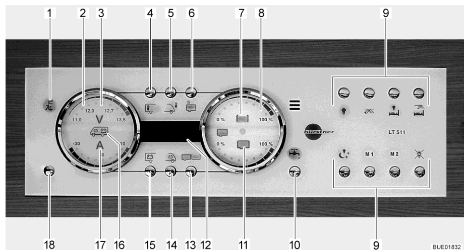
Billede 120 Panel LT 511
