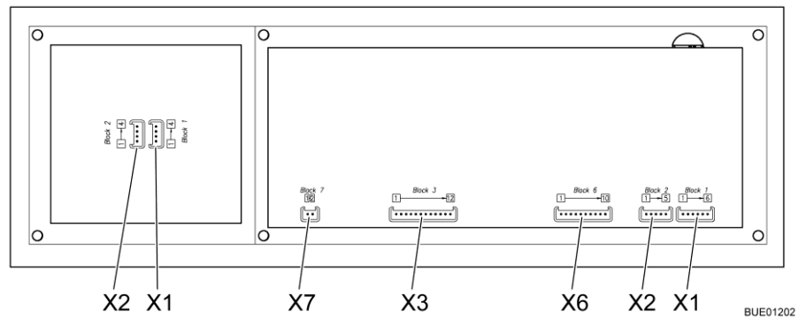
Billede 134 Blokstrømskema, panel (LT 511)
