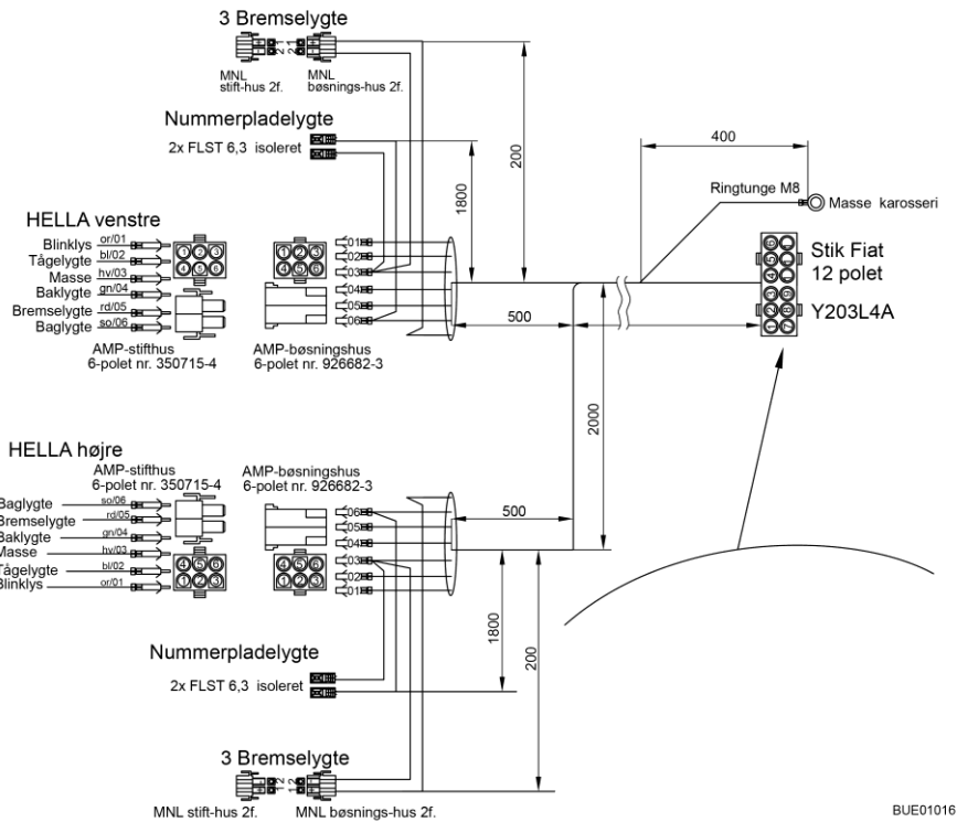
Billede 135 Strømdiagram udvendig
