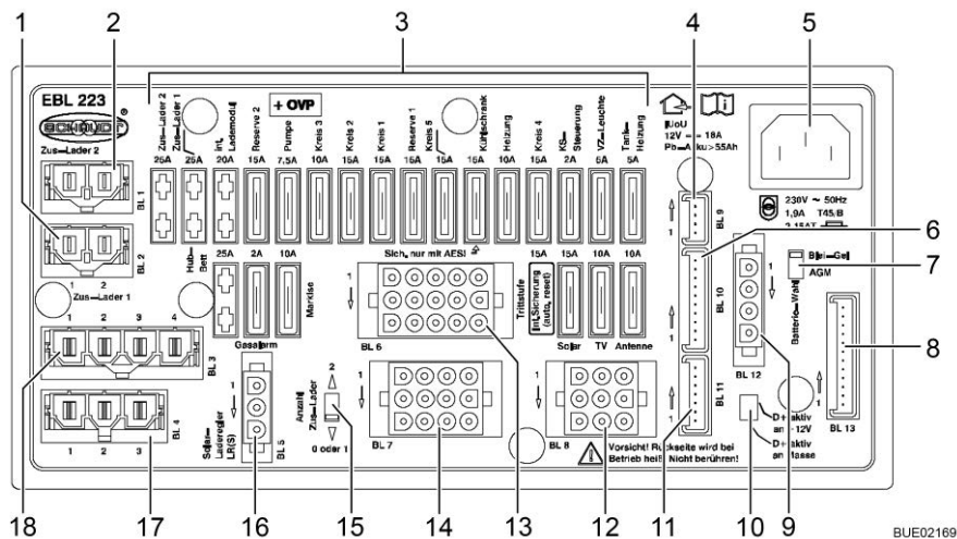
Afb. 139 Elektroblok (EBL 223)
