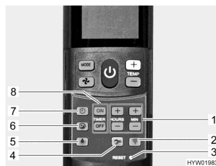
Afb. 172 Afstandsbediening met insteltoetsen (klimaatregeling)
