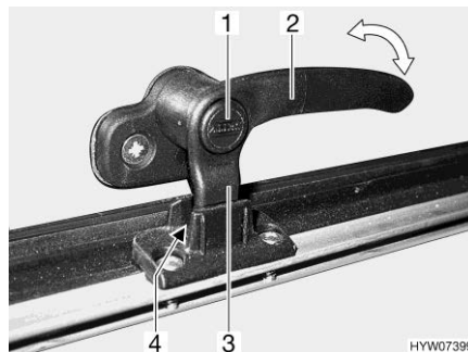
Afb. 98 Vergrendelingshendel met vergrendelingsknop in stand "continue ventilatie"
