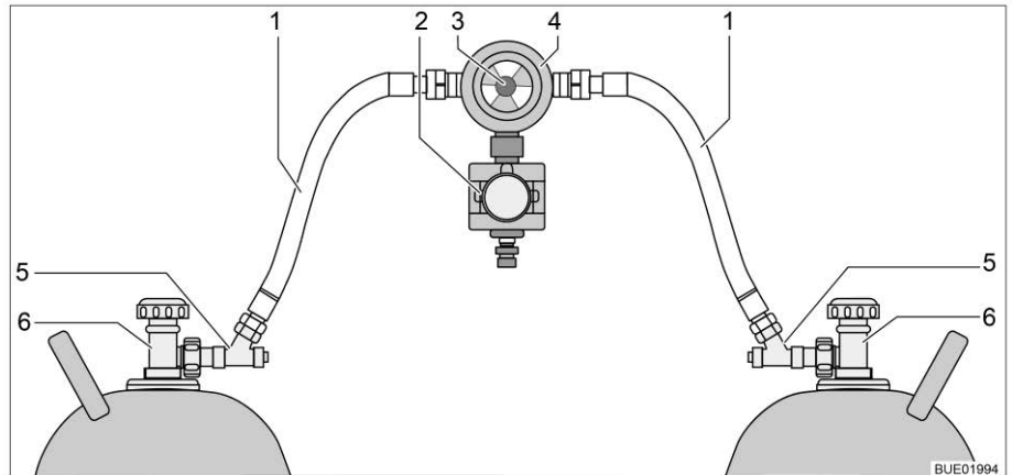
Afb. 22 Gasdrukregelaar met CPU en slangbreukbeveiliging
