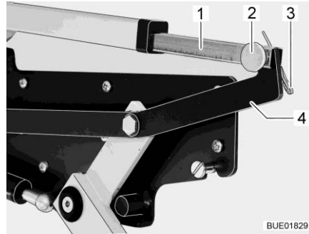
Afb. 124 Aandrijving voor hefbed
