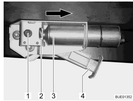
Afb. 52 Elektrische hefsteun aan het voertuig
