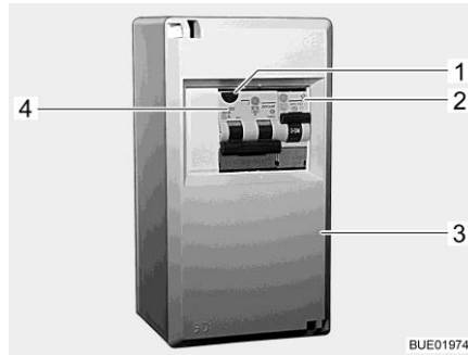
Afb. 149 230-V-zekeringenkast
