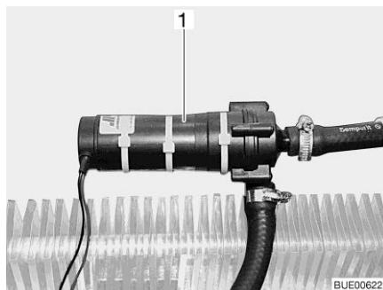
Afb. 163 Extra circulatiepomp
