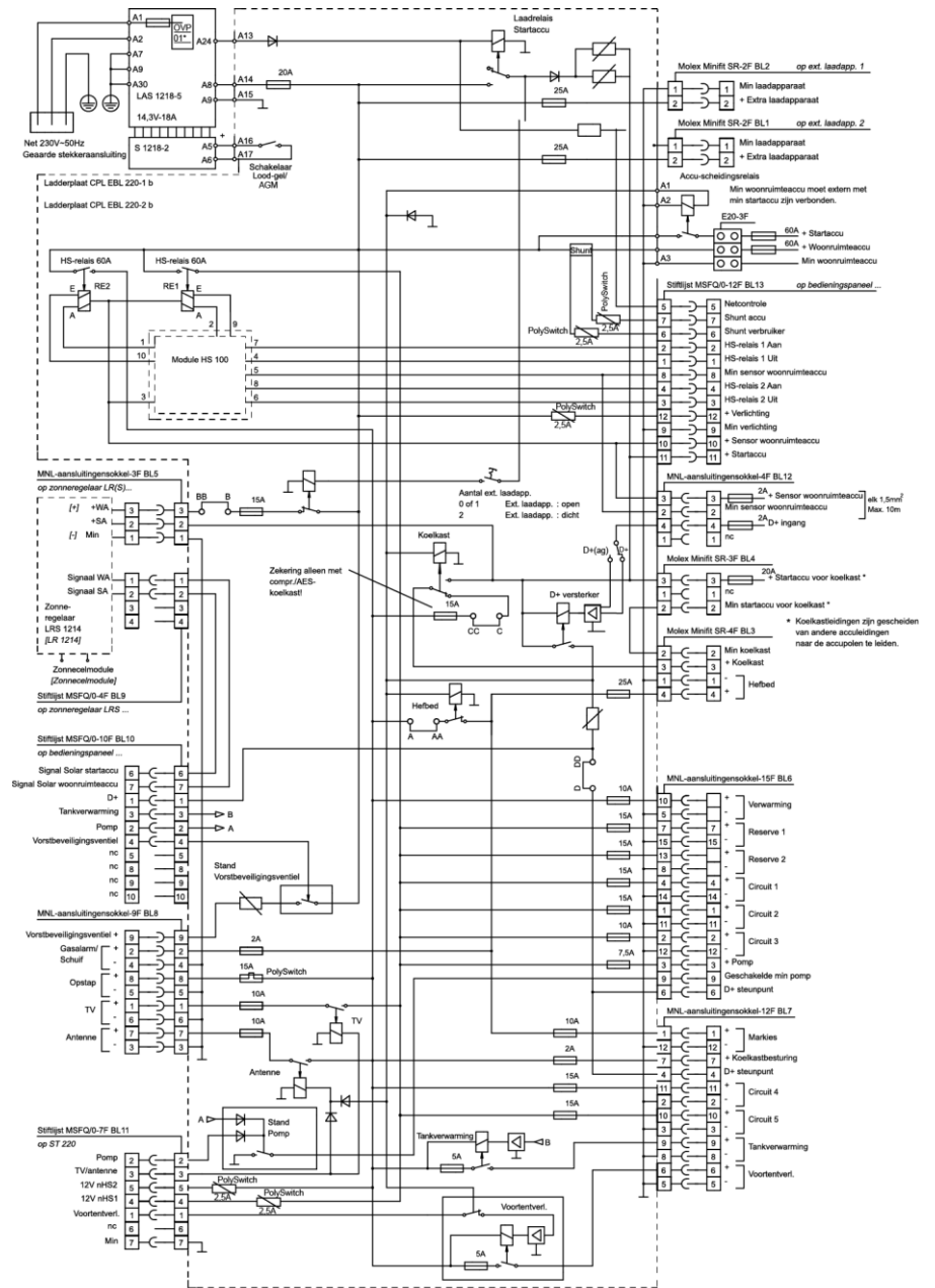
Afb. 153 Stroomschema binnen (EBL 223)
