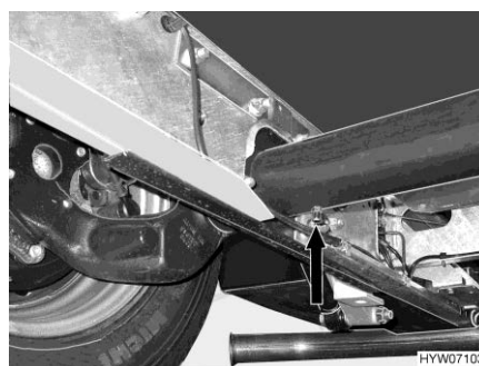
Afb. 224 AL-KO achteras (Fiat)
