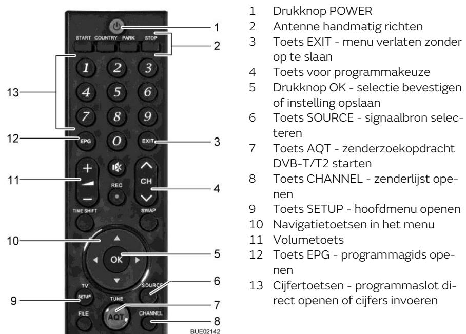
Afb. 57 Afstandsbediening
