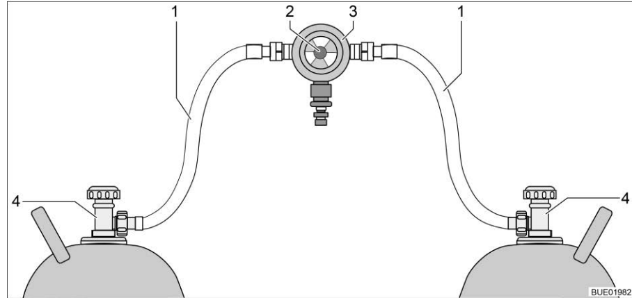
Afb. 132 Omschakelinstallatie voor gasflessen
