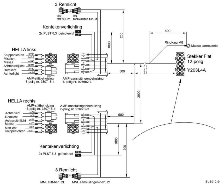
Afb. 155 Stroomschema buiten
