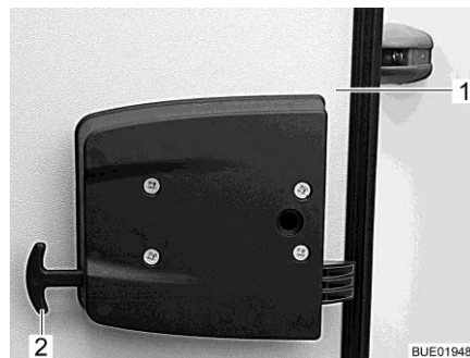
Afb. 68 Noodontgrendeling garageluik
