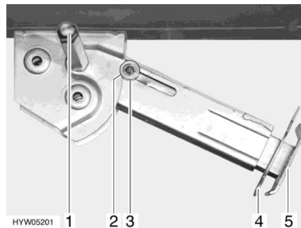
Afb. 49 Hefsteun
