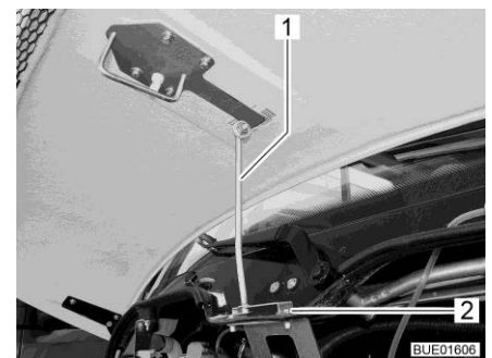
Afb. 40 Steun motorkap
