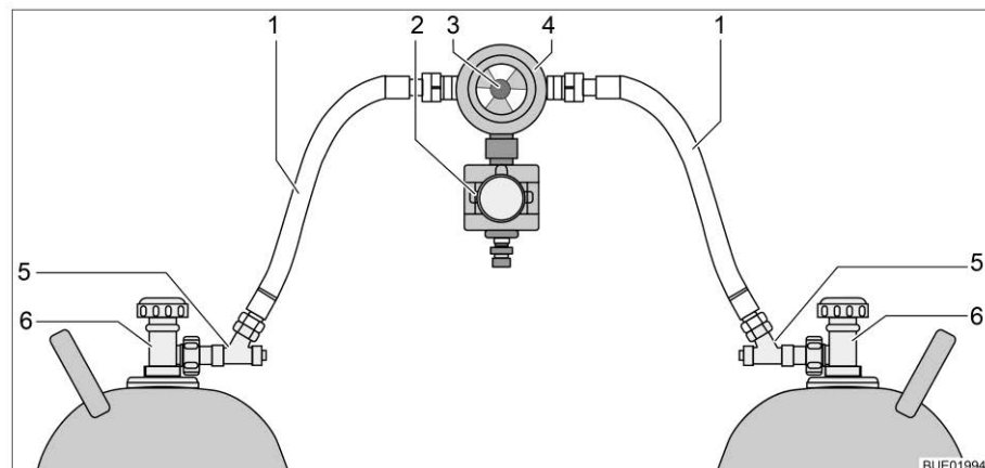
Afb. 133 Omschakelinstallatie voor gasflessen met CPU
