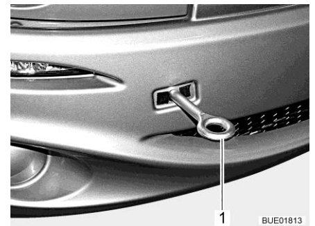
Afb. 48 Sleepoog, gemonteerd
