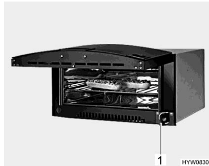
Fig. 245 Four à gaz (Dometic TecTower)
