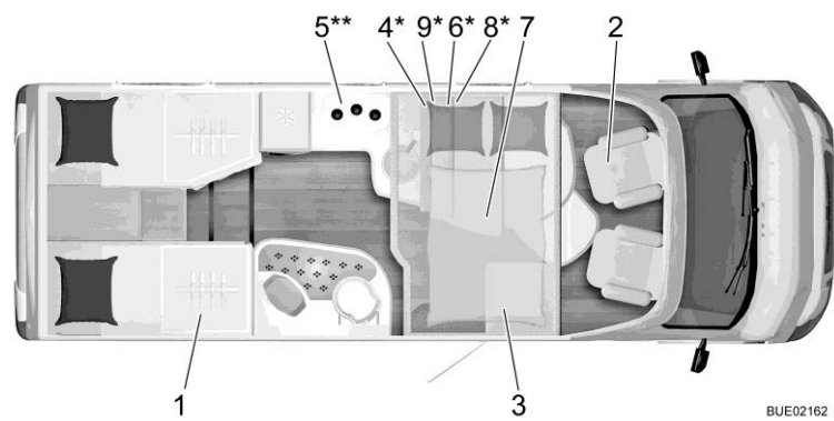
Fig. 342 Tracé Ixeo Time IT 726 G
