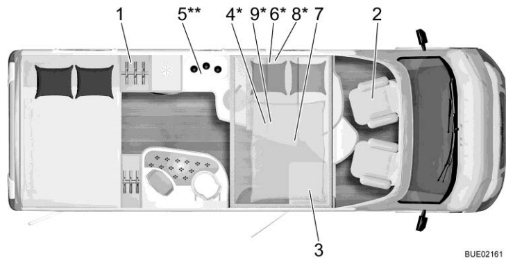
Fig. 341 Tracé Ixeo Time IT 710 G
