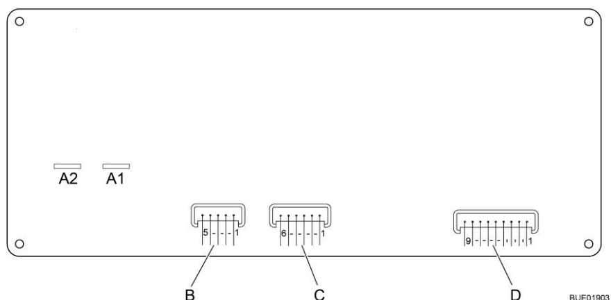
Fig. 213 Schéma de connexions, panneau de contrôle (LT 96)
