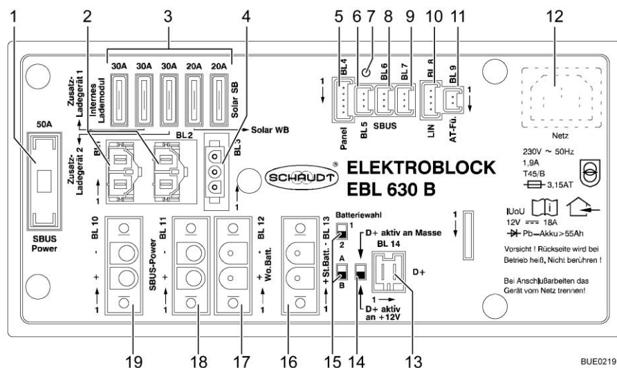
Fig. 187 Bloc électrique (EBL 630)
