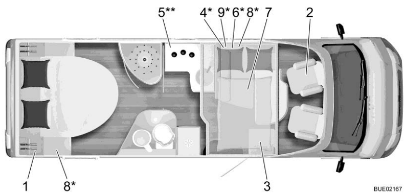
Fig. 343 Tracé Ixeo Time IT 734
