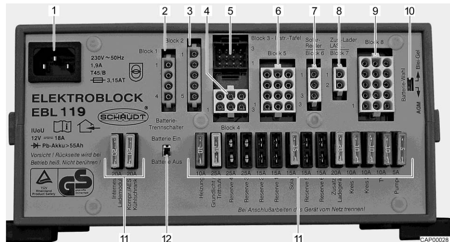
Fig. 186 Bloc électrique (EBL 119)
