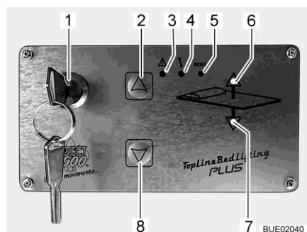
Fig. 324 Commande
