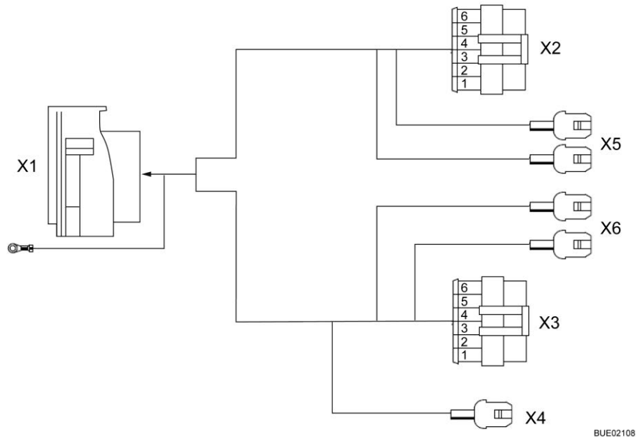
Fig. 215 Schéma électrique extérieur
