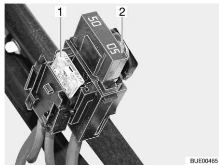
Fig. 196 Fusibles de la batterie de démarrage
