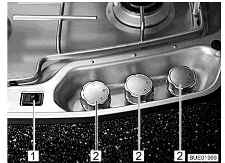
Fig. 242 Boutons de commande pour le réchaud à gaz (alternative)
