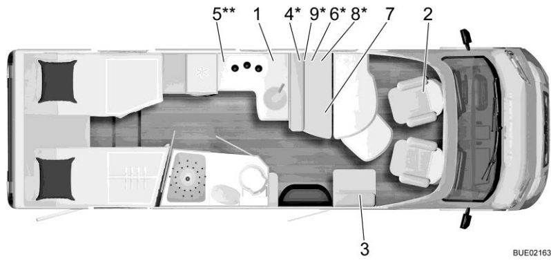
Fig. 333 Tracé Lyseo TD 728 G
