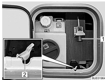
Fig. 193 Raccordement 230 V sur le véhicule (avec unité de service)
