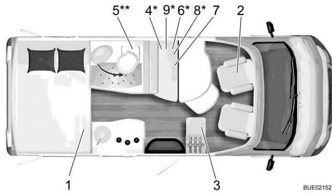
Fig. 339 Tracé Travel Van T 590 G
