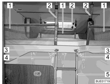
Fig. 142 Lit escamotable avec filet de sécurité tendu
