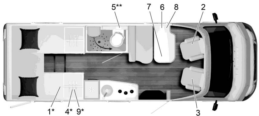
Fig. 325 Tracé Lyseo Time T 690 G
