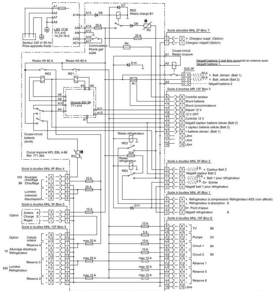
Fig. 211 Schéma électrique intérieur (EBL 119)
