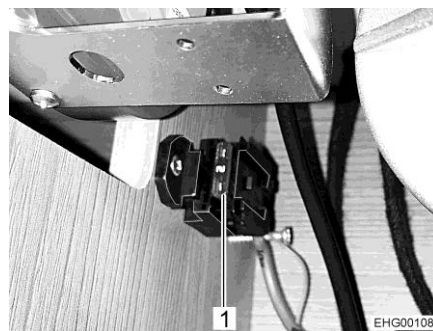
Fig. 205 Fusible du lit escamotable (Ixeo T)
