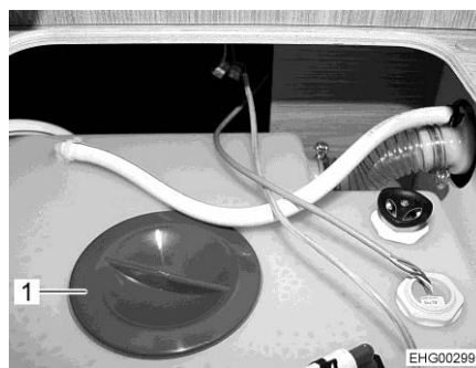
Fig. 302 Ouverture de nettoyage du réservoir d'eau
