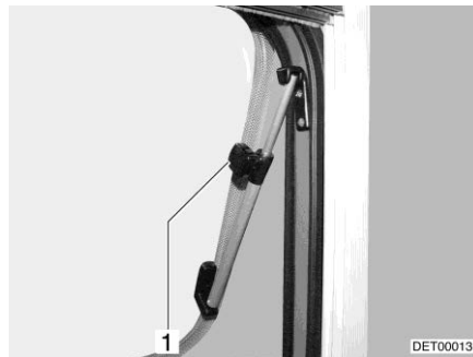
Fig. 95 Fenêtre projetante avec bras pivotant
