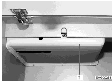
Fig. 204 Habillage dans le meuble haut
