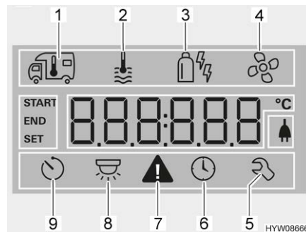
Fig. 220 Écran (unité de commande)
