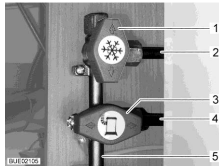
Fig. 175 Position des robinets d'arrêt de gaz (exemple)
