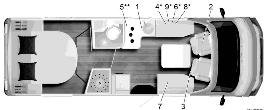
Fig. 349 Tracé Ixeo T 736
