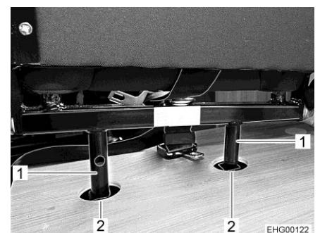
Fig. 31 Montants (insérés)
