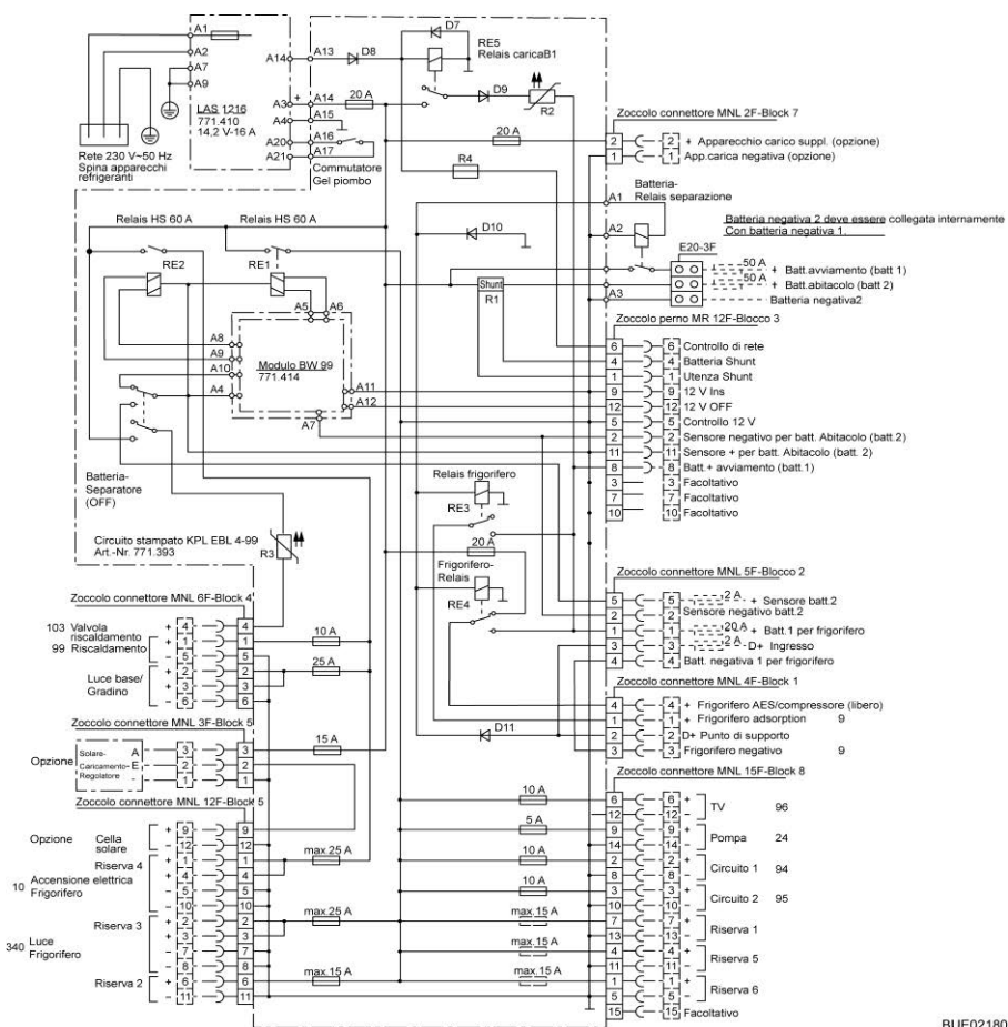
Fig. 201 Schema elettrico interno (EBL 119)
