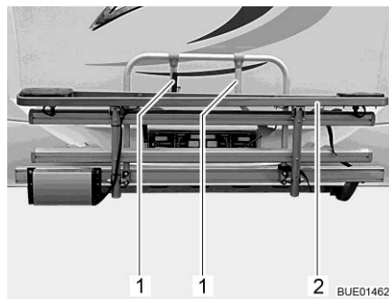
Fig. 4 Portabiciclette e-bike
