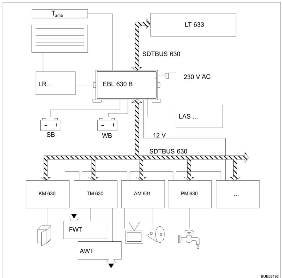
Fig. 202 Schema a blocchi alimentazione energia EBL 630
