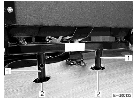
Fig. 30 Longheroni (inseriti)
