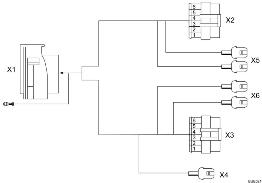
Fig. 205 Schema elettrico esterno
