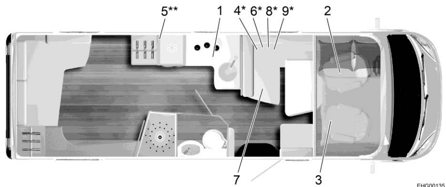
Fig. 319 Pianta I 746
