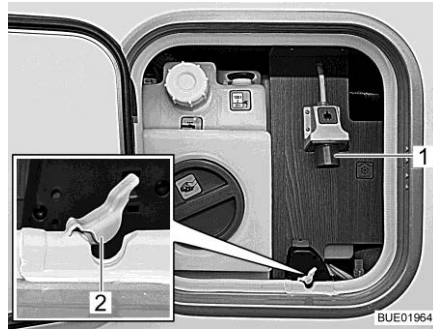
Fig. 188 Collegamento a 230 V al veicolo (con unità di servizio)
