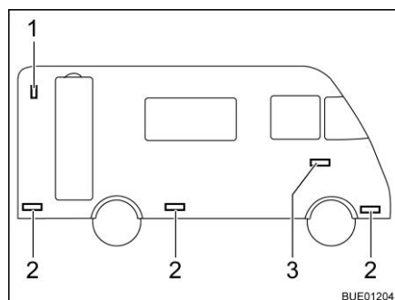
Fig. 295 Luci laterali
