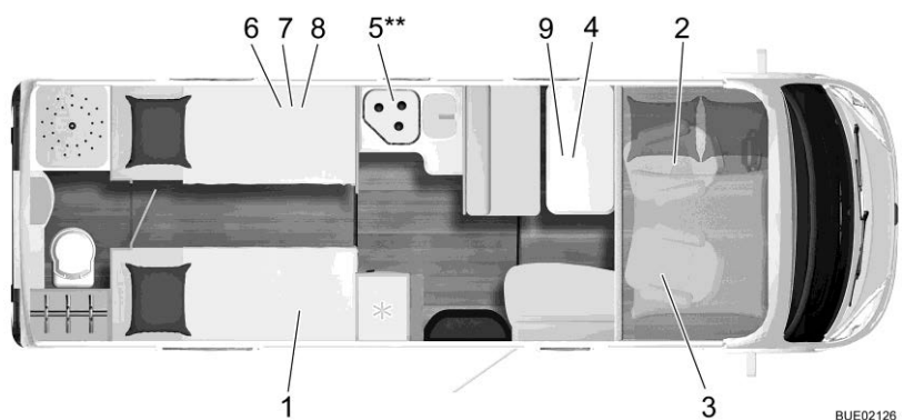
Fig. 308 Pianta I 720
