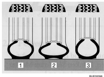
Fig. 230 Base di appoggio dei pneumatici
