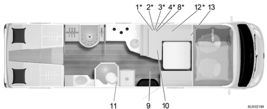
Fig. 232 Pianta I 910 G Elegance
