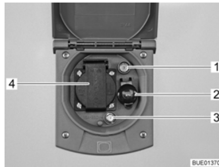
Fig. 148 Presa esterna
