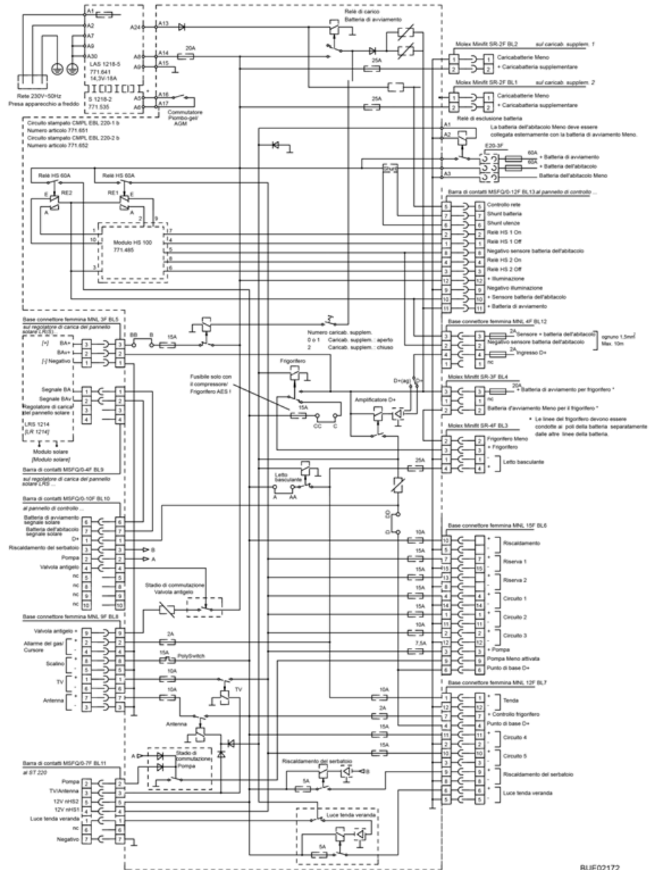
Fig. 151 Schema elettrico interno (EBL 223)
