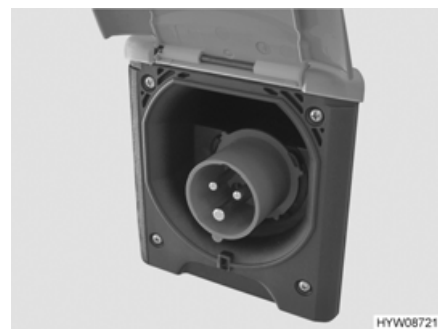
Fig. 142 Collegamento a 230 V sul veicolo
