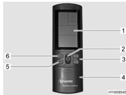
Fig. 168 Telecomando (impianto di climatizzazione)
