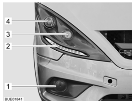
Fig. 215 Luci frontali
