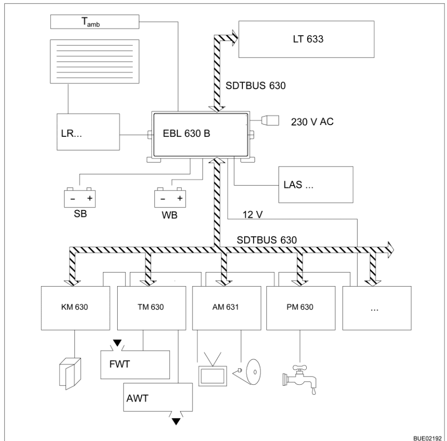
Fig. 199 Schema a blocchi alimentazione energia EBL 630
