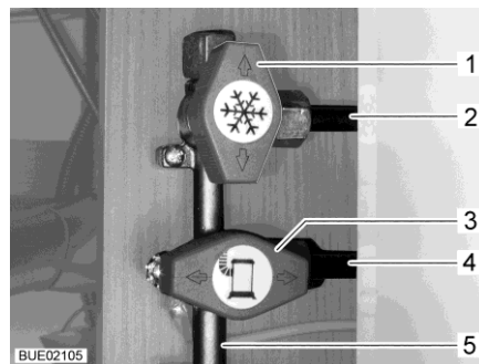
Fig. 168 Posizione dei rubinetti di arresto del gas (esempio)
