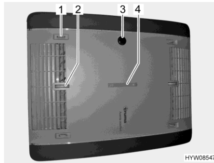
Fig. 223 Indicatore di funzionamento e distribuzione dell'aria (impianto di climatizzazione)
