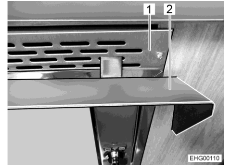
Fig. 230 Lamiera di protezione dal calore (agganciata)
