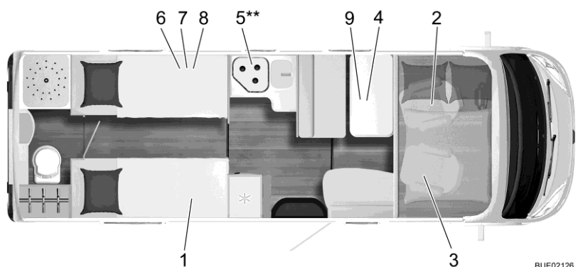
Fig. 308 Pianta I 720
