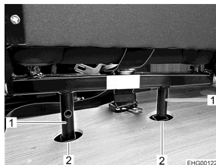
Fig. 32 Longheroni (inseriti)
