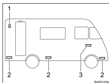
Fig. 293 Luci laterali
