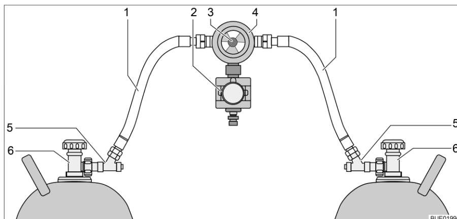
Fig. 17 Regolatore del gas con CPU e dispositivo antirottura del tubo flessibile
