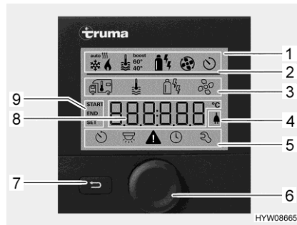
Fig. 206 Centralina di controllo con indicazioni
