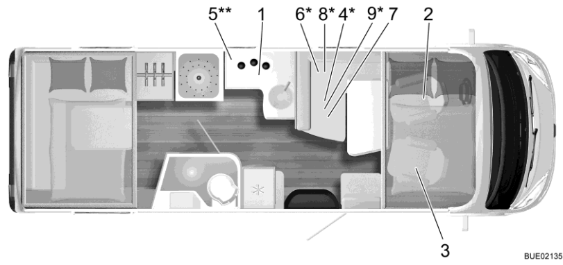
Fig. 318 Pianta I 744
