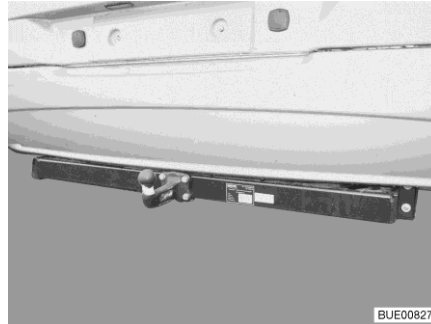
Fig. 9 Gancio di traino, fisso
