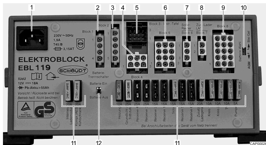
Fig. 179 Centralina elettrica (EBL 119)
