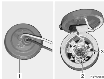
Fig. 289 Luce fendinebbia
