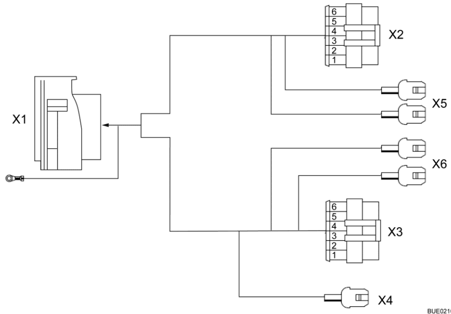
Fig. 202 Schema elettrico esterno
