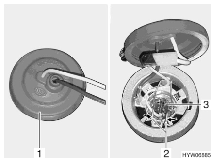
Fig. 284 Faro (vista dall'interno)
