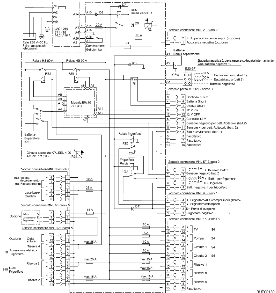
Fig. 198 Schema elettrico interno (EBL 119)
