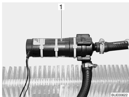
Fig. 215 Pompa di circolazione aggiuntiva
