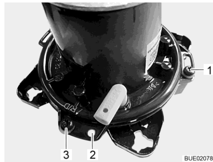
Fig. 285 Regolazione faretto (in figura: guida a destra)
