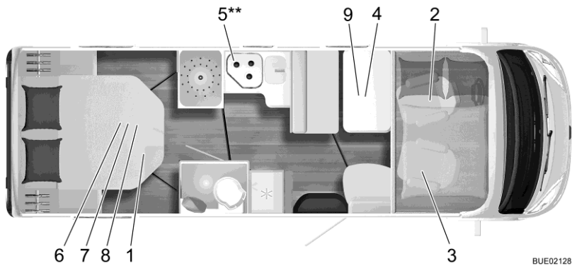
Fig. 310 Pianta I 734 G
