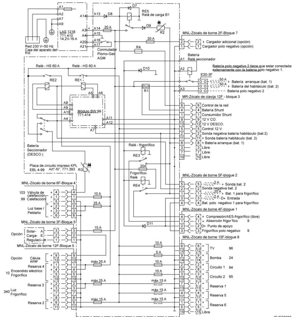
Fig. 198 Esquema de circuitos interior (EBL 119)
