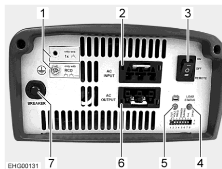
Fig. 180 Ondulator
