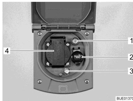
Fig. 195 Caja de enchufe exterior
