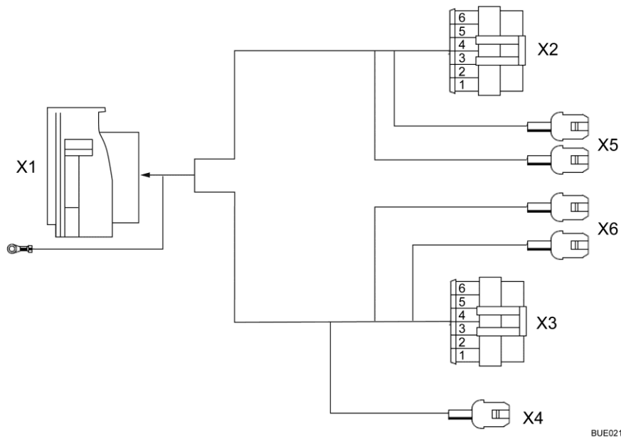
Fig. 202 Esquema de circuitos exterior
