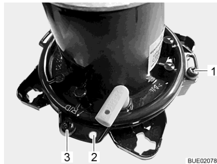
Fig. 285 Ajuste de faros (representación: circulación por la derecha)
