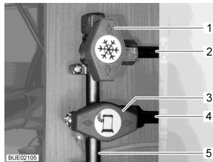
Fig. 168 Posición de las válvulas de paso de gas (ejemplo)
