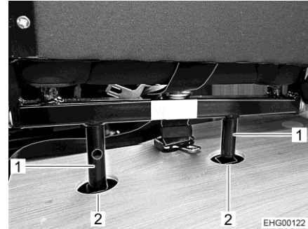
Fig. 32 Largueros (insertados)
