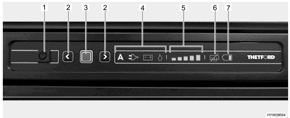
Fig. 239 Cuadro de mando de LED (frigorífico Thetford)
