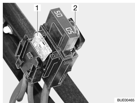
Fig. 191 Fusibles en la batería del motor de arranque
