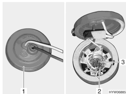
Fig. 284 Faros (vista desde el interior)
