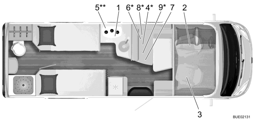
Fig. 313 Esquema I 720
