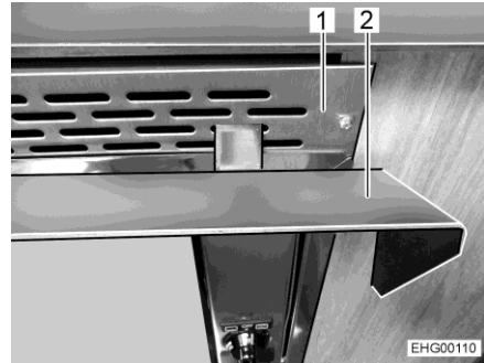
Fig. 230 Chapa protectora de calor (enganchada)
