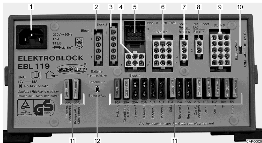
Fig. 179 Bloque eléctrico (EBL 119)
