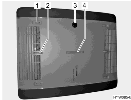
Fig. 223 Visualización de funcionamiento y distribución de aire (instalación de aire acondicionado)
