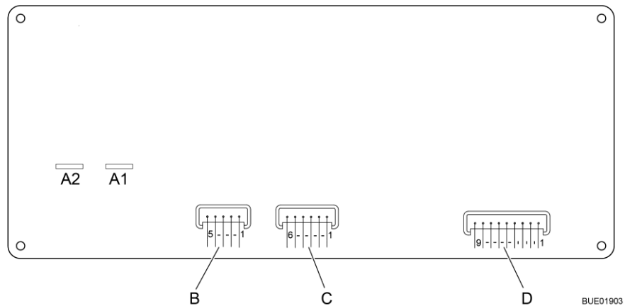
Fig. 200 Esquema de conexión, panel (LT 96)
