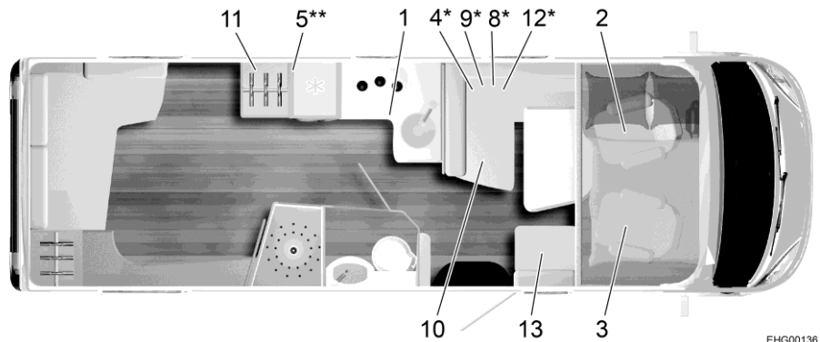
Fig. 320 Esquema I 746 Comoencasa 6.0
