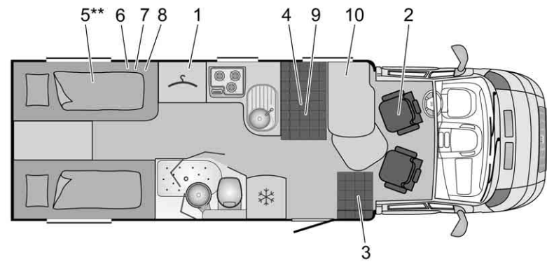
Fig. 301 Pianta T 729 Nexxo
