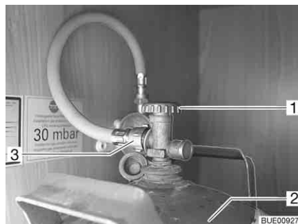
Fig. 157 Vano portabombole
