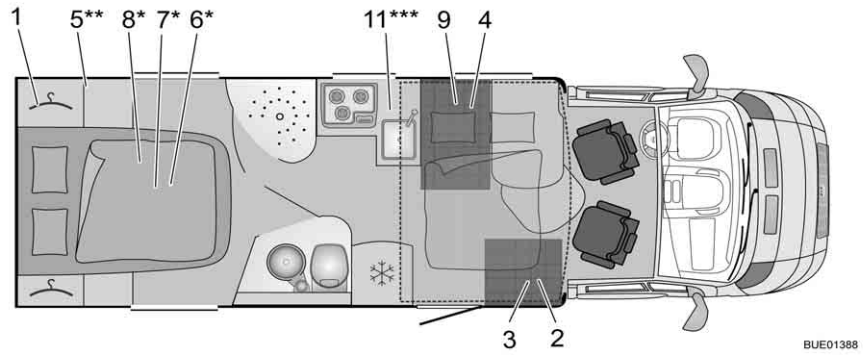
Fig. 303 Pianta IT 735 Ixeo
