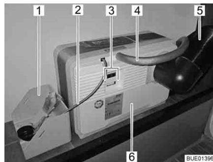
Fig. 168 Pila a combustibile con cartuccia del serbatoio
