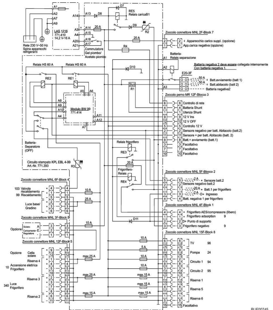
Fig. 188 Schema elettrico interno (EBL 99)
