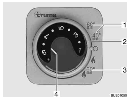
Fig. 215 Centralina di controllo per riscaldamento/boiler
