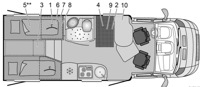
Fig. 294 Pianta T 690 G Nexxo
