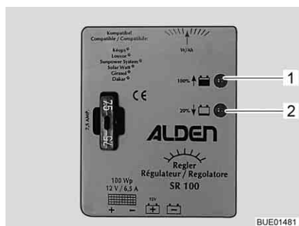
Fig. 171 Regolatore di carica del pannello solare 100 W
