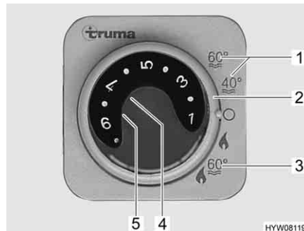
Fig. 212 Centralina di controllo per riscaldamento/boiler
