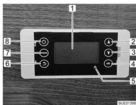
Fig. 170 Centralina di controllo per pila a combustibile
