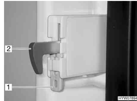
Fig. 232 Fissaggio del gancio di bloccaggio
