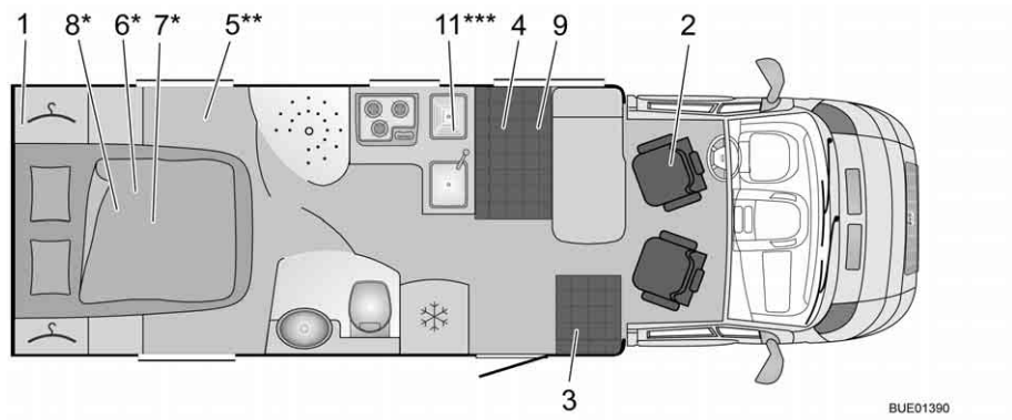
Fig. 304 Pianta T 740 Nexxo
