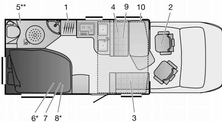
Fig. 292 Pianta IT 664 Ixeo
