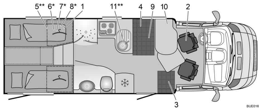
Fig. 300 Pianta T 728 G Nexxo
