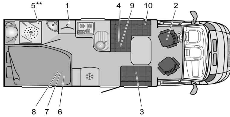
Fig. 291 Pianta T 660 Nexxo
