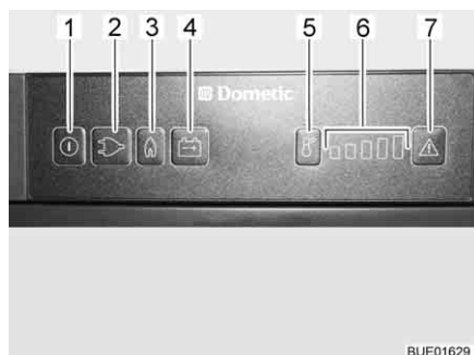
Fig. 228 Elementi di comando per il frigorifero (serie Dometic 8 con SMSE)
