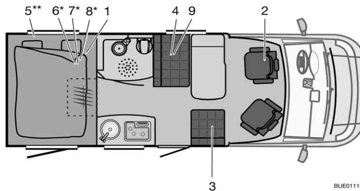
Fig. 286 Pianta T 571 G Travel Van
