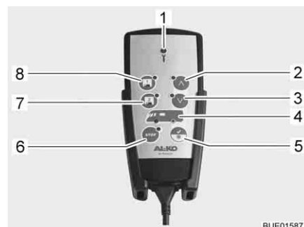
Fig. 27 Telecomando
