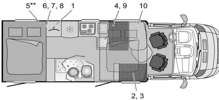
Fig. 297 Pianta IT 710 G Ixeo Time
