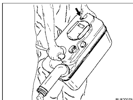
Afb. 219 Thetford-cassette leegmaken
