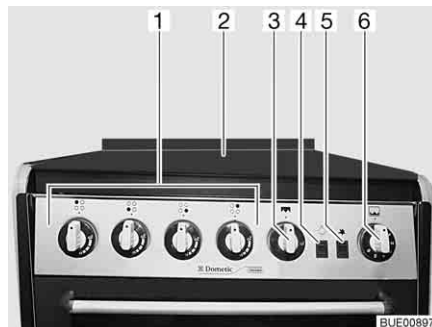
Afb. 181 Gaskooktoestel met bakoven en grill
