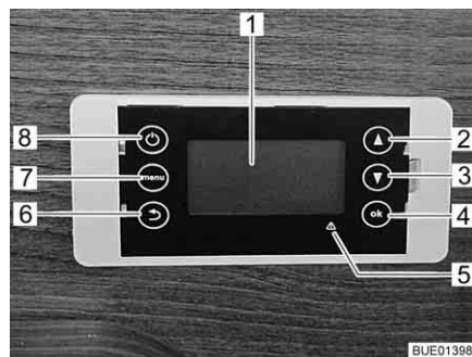
Afb. 136 Bedieningspaneel brandstofcel
