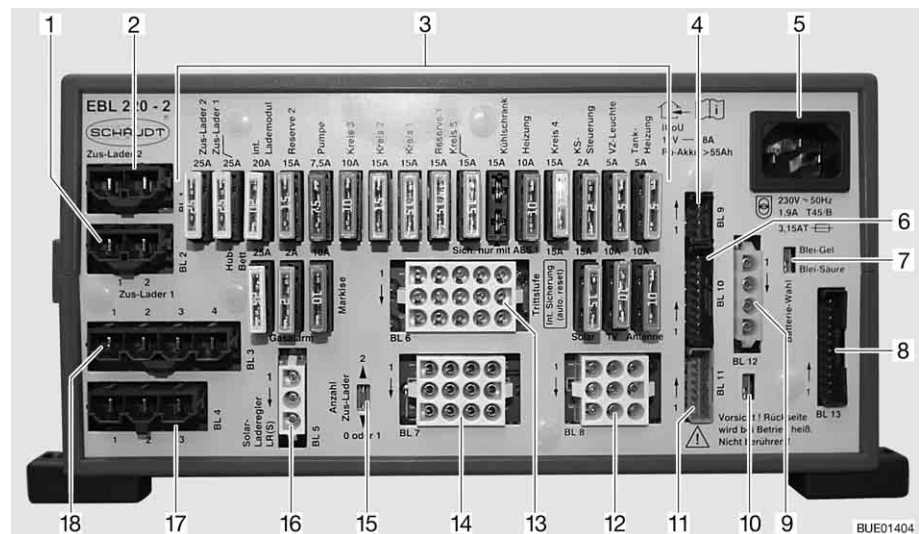
Afb. 131 Elektroblok (EBL 220)
