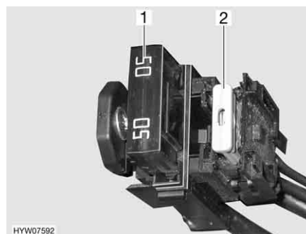
Afb. 143 Zekeringen aan de woonruimteaccu
