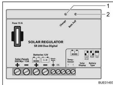
Afb. 138 Zonneregelaar 200 W
