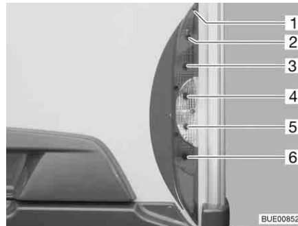
Afb. 238 Verlichting achter
