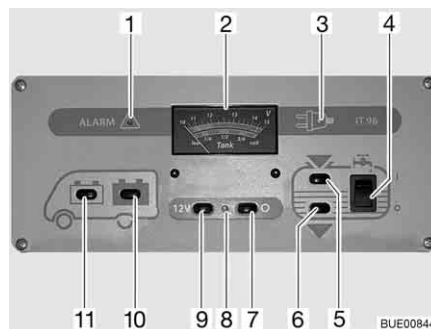
Afb. 132 Paneel IT 96-2
