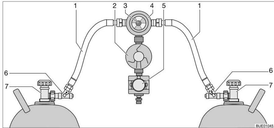
Afb. 125 Omschakelinstallatie Crash-Protection-Unit
