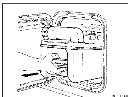
Afb. 217 Thetford-cassette uitnemen
