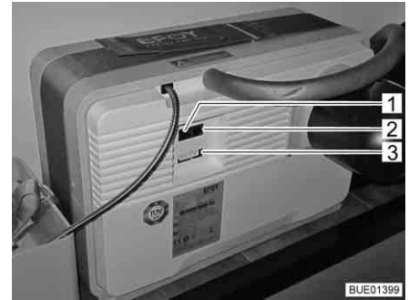
Afb. 135 Aansluitveld brandstofcel
