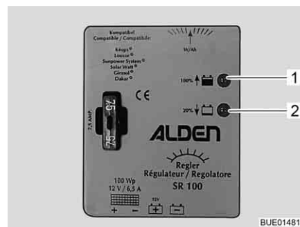
Afb. 137 Zonneregelaar 100 W
