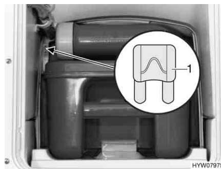
Afb. 144 Zekering van het Thetford-toilet
