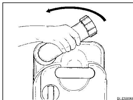
Afb. 223 Aftapaansluiting draaien
