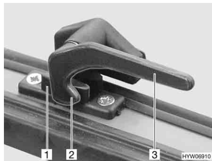
Afb. 96 Vergrendelingshendel in stand "gesloten"
