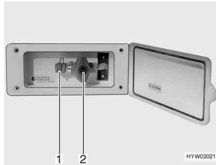
Afb. 124 Externe gasaansluiting, gasafsluitkraan gesloten
