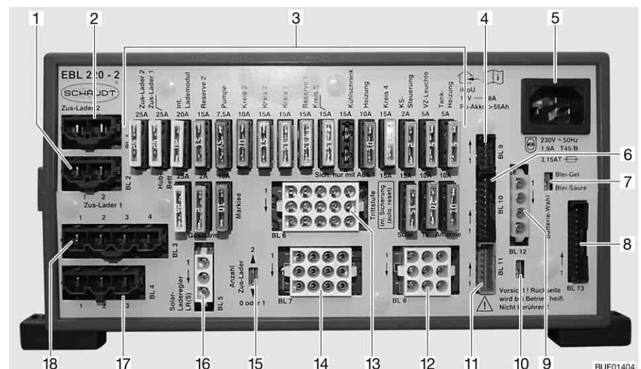
Afb. 155 Elektroblok (EBL 220)
