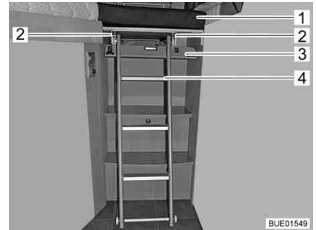
Afb. 138 Bedverbreding met bedladder
