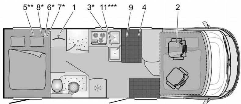
Afb. 323 Plattegrond I 737 G Viso
