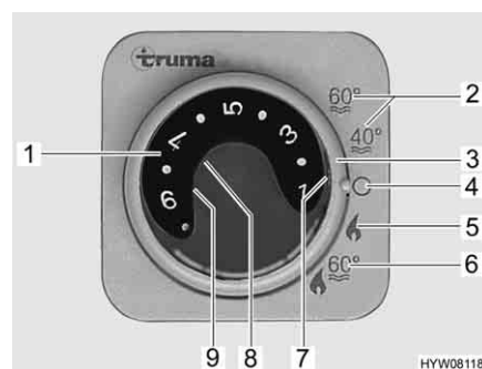
Afb. 189 Bedieningspaneel voor verwarming/boiler
