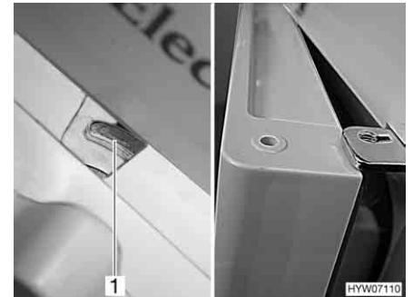
Afb. 224 Koelkastdeur/vriesvakdeur in ventilatiestand (Dometic 7-serie met apart vriesvak)
