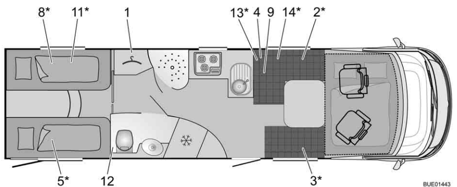
Afb. 331 Plattegrond | 895 G Elegance
