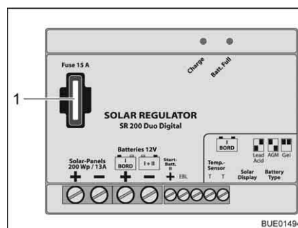
Afb. 175 Zekering zonneregelaar 200 W
