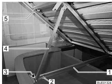
Afb. 127 Vast bed
