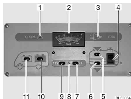
Afb. 156 Paneel IT 96-2
