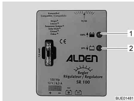
Afb. 163 Zonneregelaar 100 W
