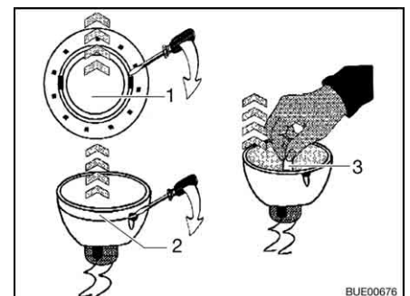
Afb. 298 De halogeengloeilamp verwisselen
