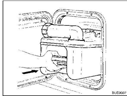
Afb. 259 Thetford-cassette inschuiven
