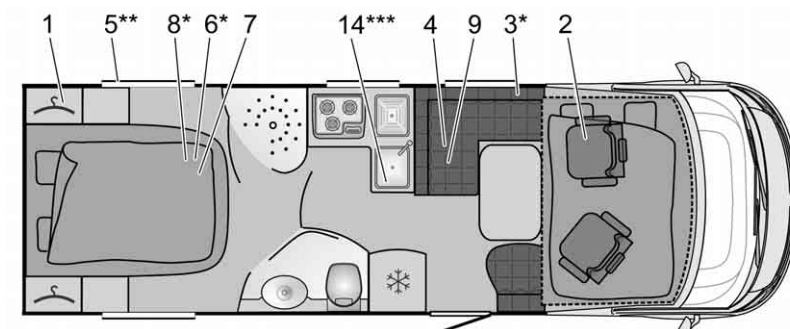
Afb. 319 Plattegrond I 726 Viseo
