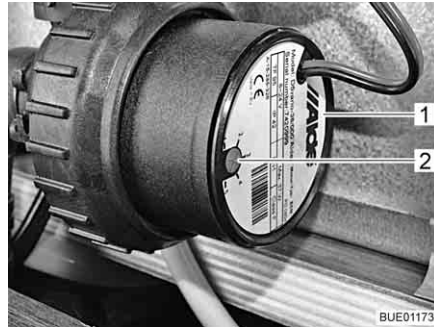
Afb. 193 Toerentalverlaging
