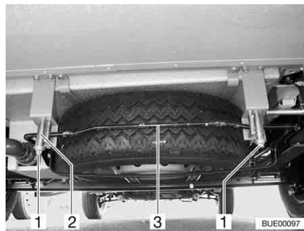
Afb. 311 Reservewielhouder (korf)
