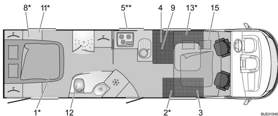
Afb. 332 Plattegrond I 910 G Grand Panorama
