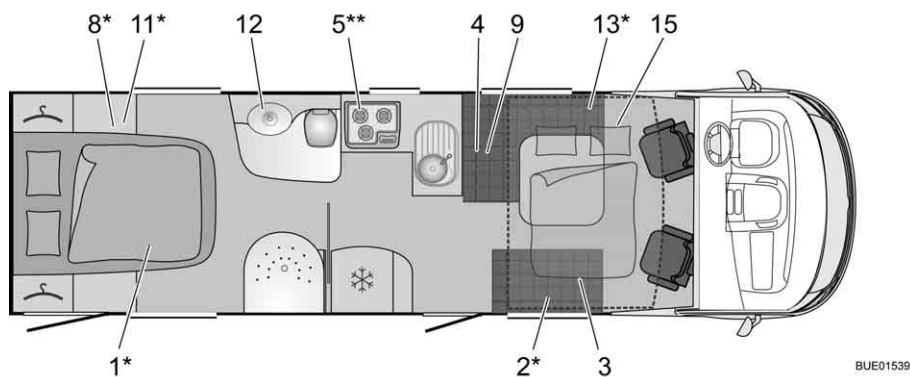
Afb. 327 Plattegrond | 830 G Grand Panorama
