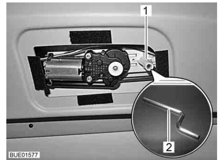
Afb. 35 Noodontgrendeling voorruitverduistering
