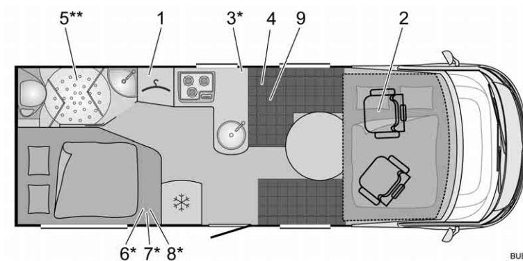
Afb. 317 Plattegrond I 709 Aviano
