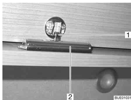
Afb. 68 Meubelluik met ontgrendelingslijst
