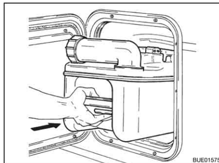
Afb. 247 Thetford-cassette inschuiven
