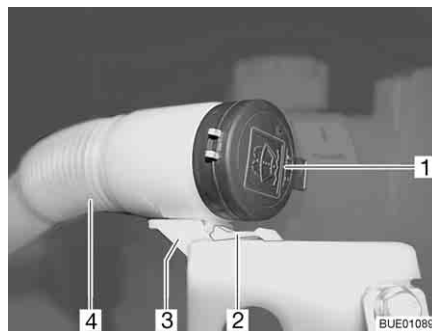
Afb. 42 Vulopening vloeistofreservoir
