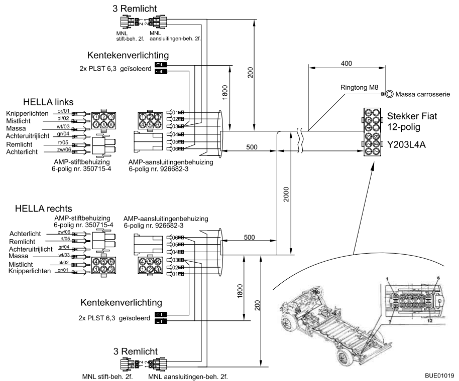
Afb. 186 Stroomschema buiten
