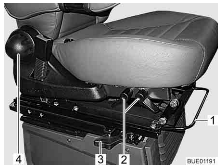
Afb. 22 Stoelverstelling
