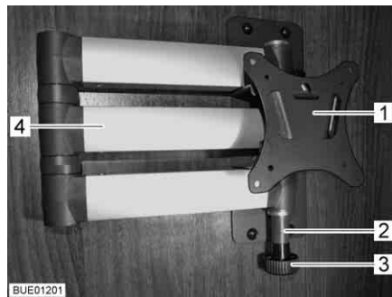
Afb. 86 Houder met scharnierarm
