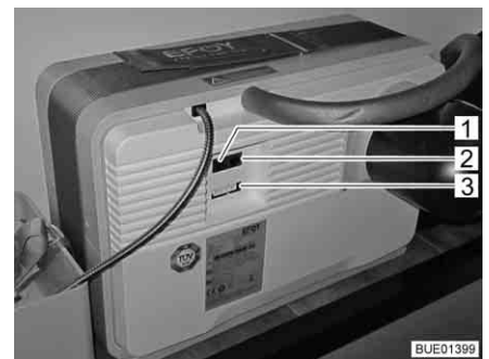
Afb. 161 Aansluitveld brandstofcel
