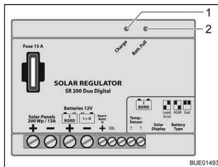
Afb. 164 Zonneregelaar 200 W
