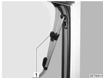
Afb. 90 Uitzetbaar raam met draaibare uitzetters
