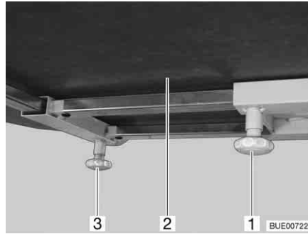
Afb. 114 Tafelblad verschuiven (alternatief)
