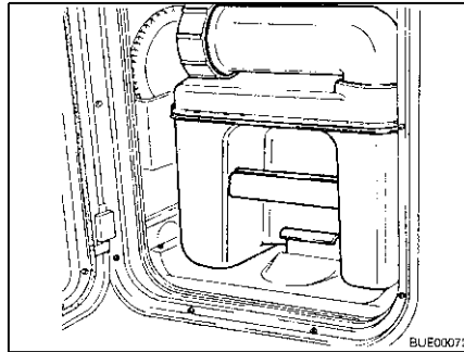
Afb. 248 Thetford-cassette vergrendeld
