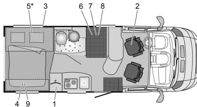
Fig. 166 Pianta T 600 Brevio
