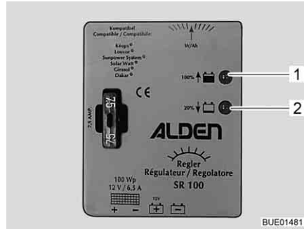
Fig. 88 Regolatore di carica del pannello solare 100 W
