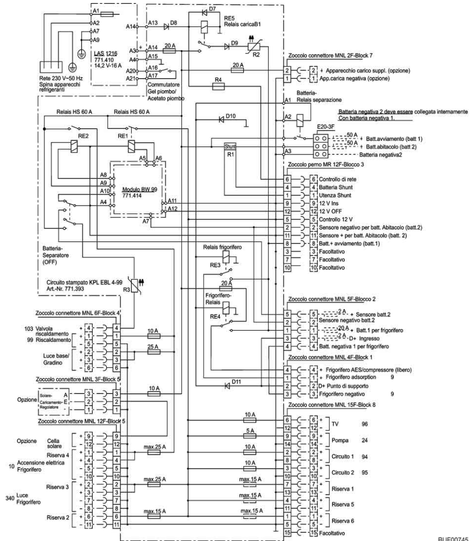
Fig. 100 Schema elettrico interno (EBL 99)
