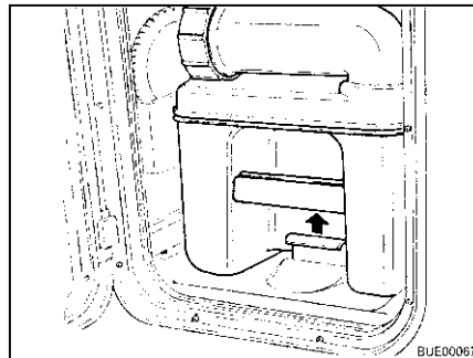
Fig. 138 Azionamento della staffa di supporto
