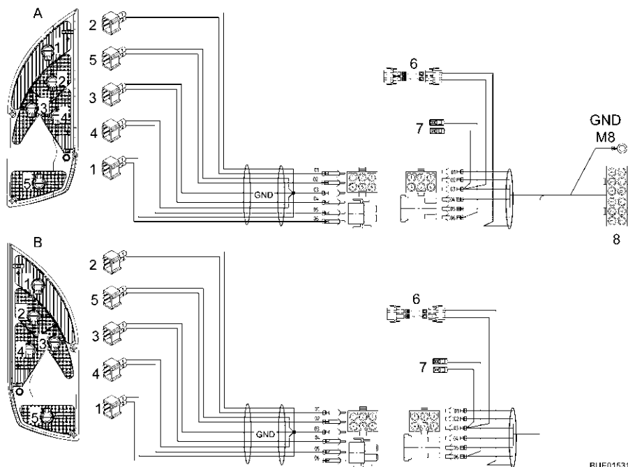
Fig. 102 Schema elettrico esterno
