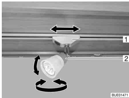
Fig. 45 Faretto
