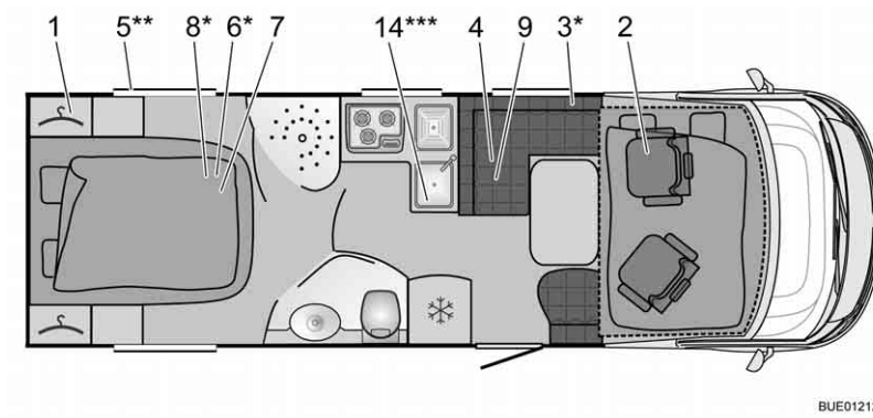
Fig. 319 Traços gerais I 726 Viseo
