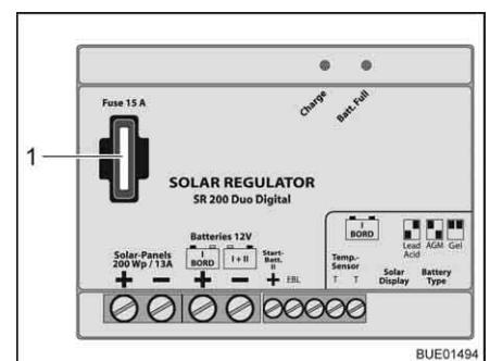
Fig. 175 Fusível do regulador de carga do painel solar 200 W
