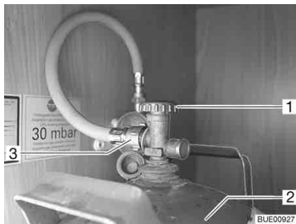
Fig. 146 Arca para as garrafas de gás
