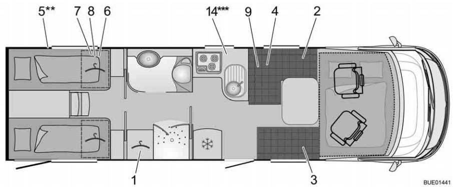
Fig. 329 Traços gerais I 875 G Aviano
