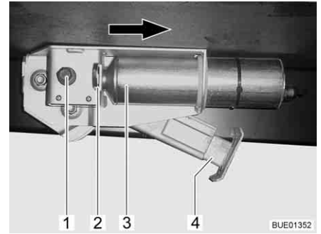
Fig. 49 Apoio de elevação elétrico no veículo
