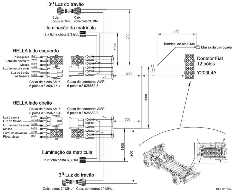
Fig. 186 Esquema elétrico exterior
