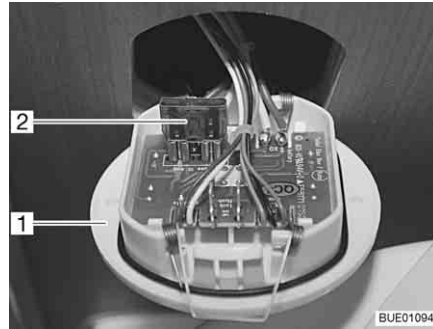
Fig. 172 Fusível da sanita
