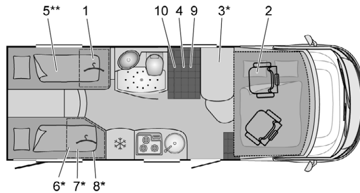
Fig. 314 Traços gerais I 690 G Viseo
