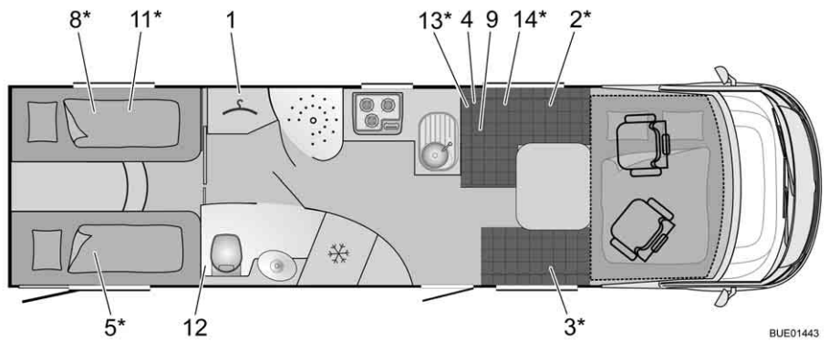
Fig. 331 Traços gerais I 895 G Elegance
