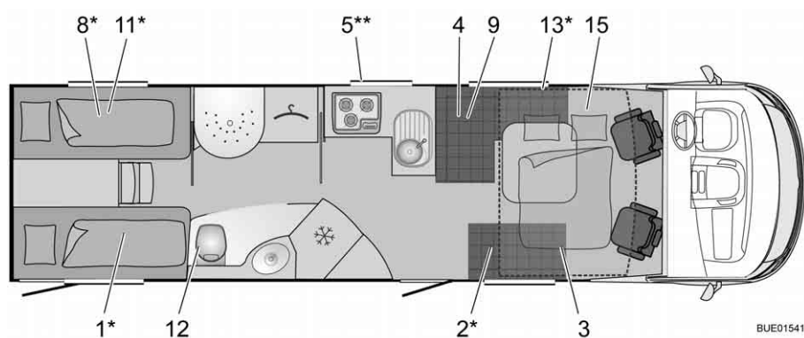
Fig. 333 Traços gerais I 915 G Grand Panorama
