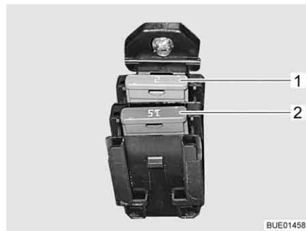
Fig. 173 Fusíveis para o gerador 12 V
