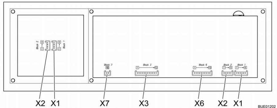
Fig. 184 Esquema elétrico da central elétrica, painel de controlo (LT 510)
