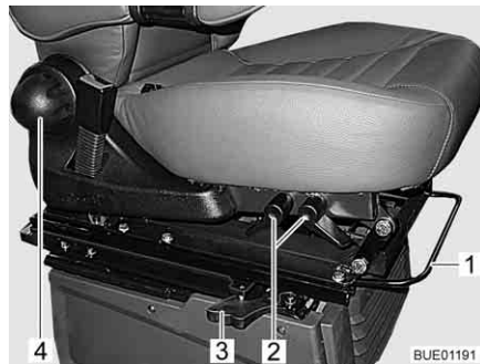
Fig. 22 Regulagem do banco
