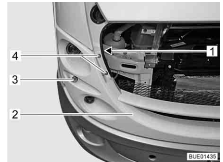
Fig. 291 Estrutura avançada de plástico com lâmpadas
