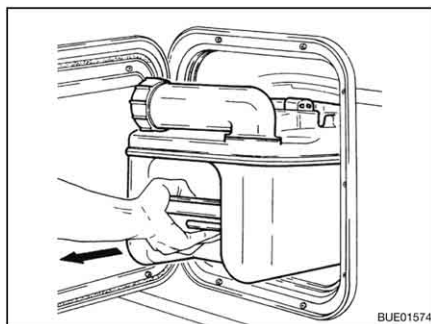
Fig. 244 Retirar a cassete Thetford
