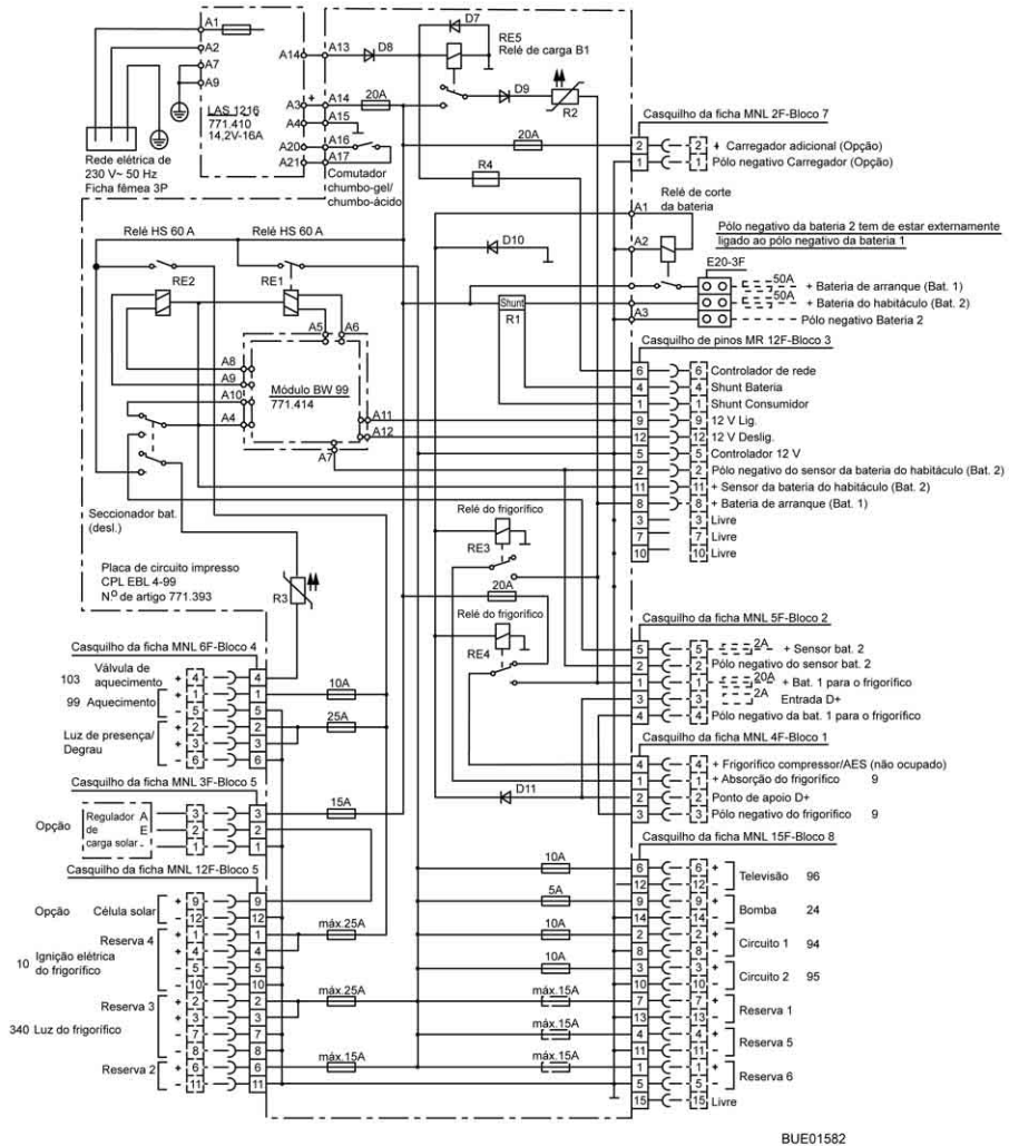
Fig. 180 Esquema elétrico interior (EBL 99)
