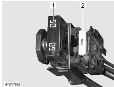
Fig. 169 Fusíveis na bateria do habitáculo
