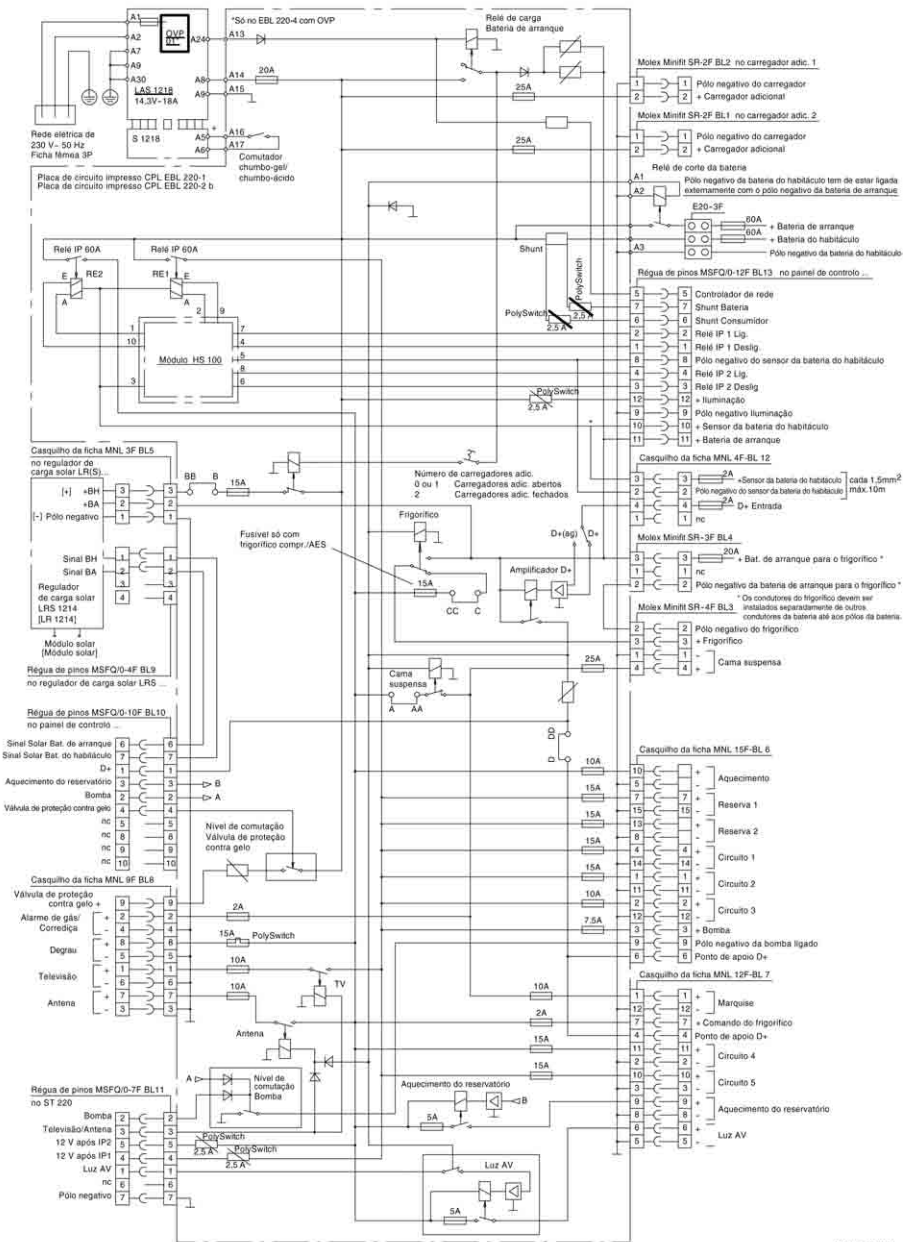
Fig. 181 Esquema elétrico interior (EBL 220)
