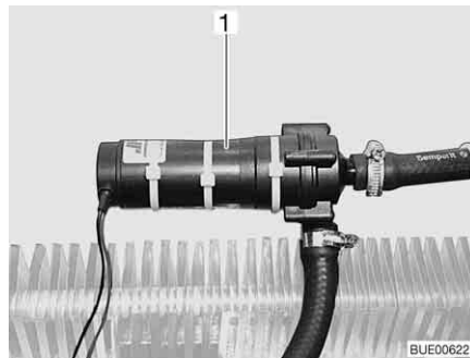
Fig. 196 Bomba de recirculação adicional
