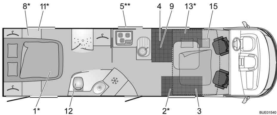
Fig. 332 Traços gerais I 910 G Grand Panorama
