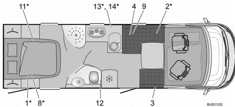
Fig. 325 Traços gerais I 800 G Elegance
