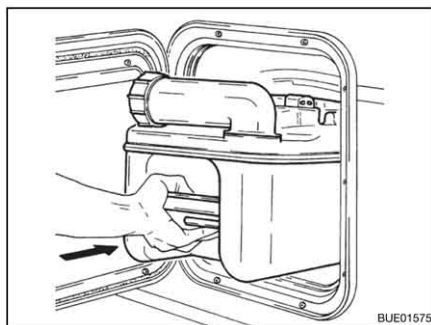
Fig. 247 Inserir para dentro a cassete Thetford
