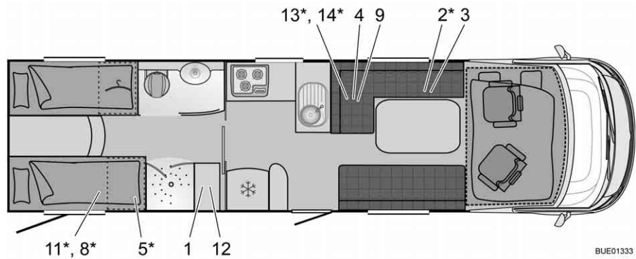
Fig. 326 Traços gerais I 810 G Elegance
