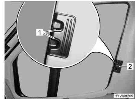
Fig. 39 Estore opaco plissado para as janelas do condutor/passageiro
