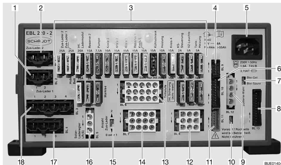
Fig. 155 Central elétrica (EBL 220)
