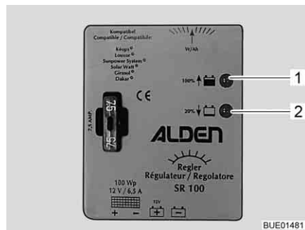
Fig. 163 Regulador de carga do painel solar 100 W
