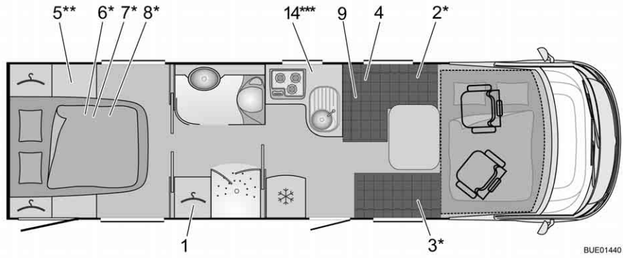
Fig. 328 Traços gerais I 870 G Aviano
