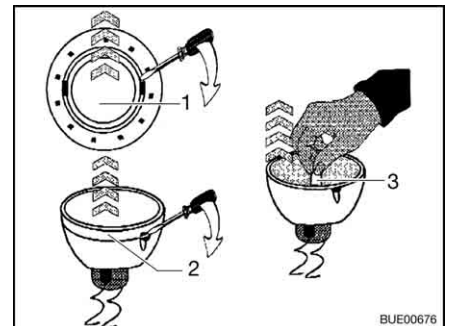
Fig. 298 Trocar a lâmpada de halogéneo
