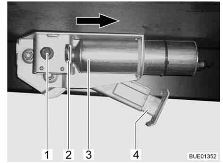
Fig. 49 Piedino di stazionamento elettrico sul veicolo
