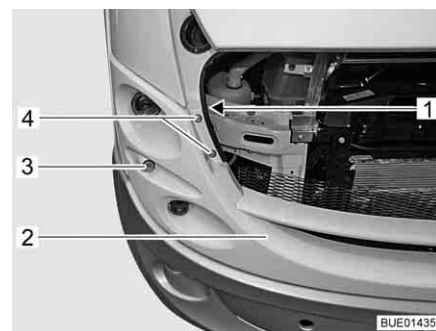
Fig. 291 Parte anteriore in plastica con lampade
