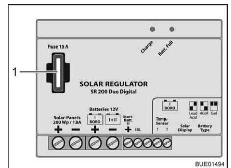
Fig. 175 Fusibile regolatore di carica del pannello solare 200 W
