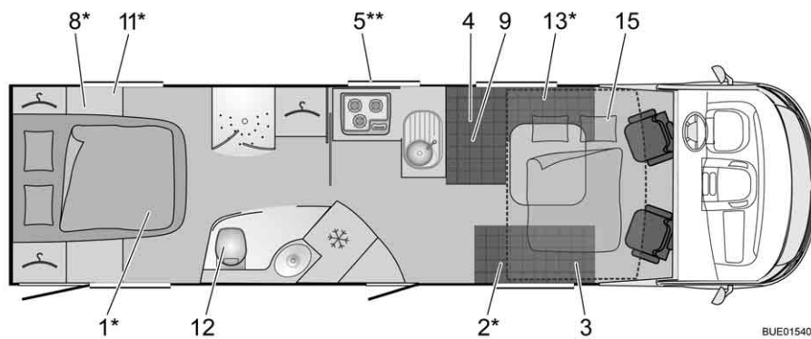
Fig. 332 Pianta I 910 G Grand Panorama
