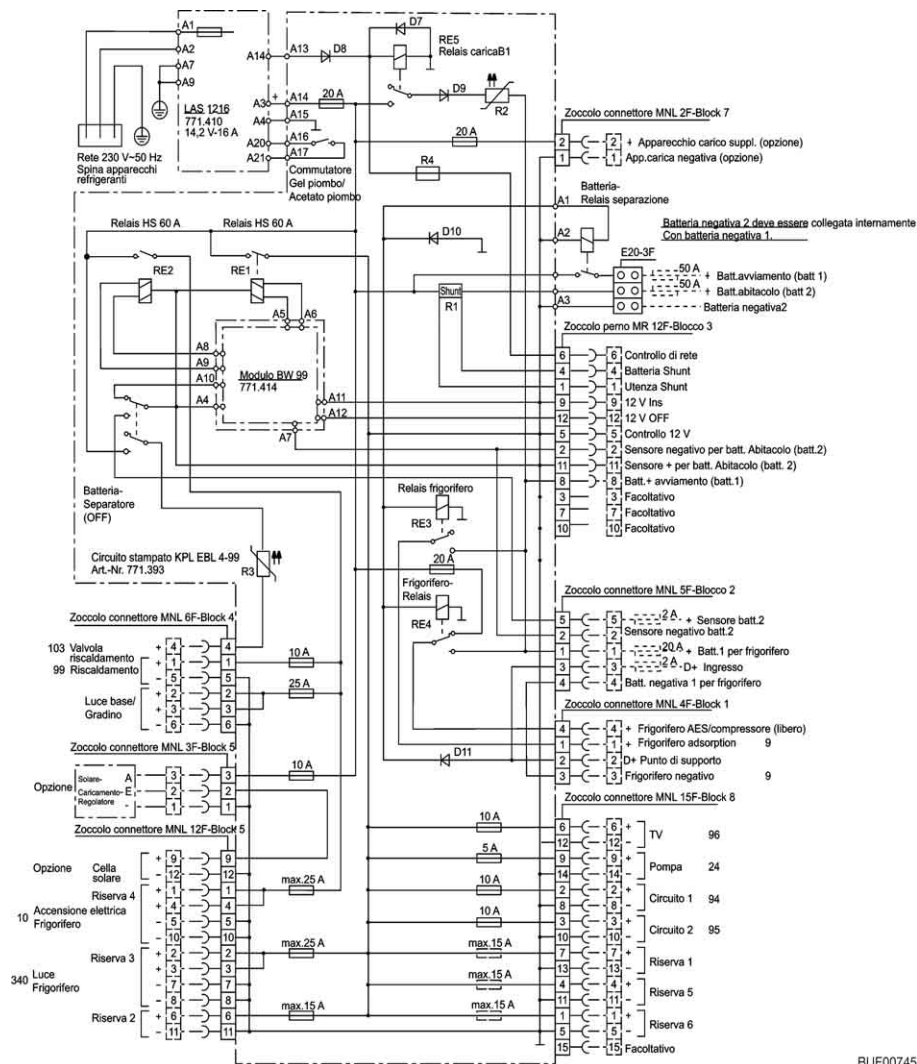
Fig. 180 Schema elettrico interno (EBL 99)
