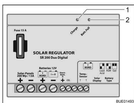
Fig. 164 Regolatore di carica del pannello solare 200 W
