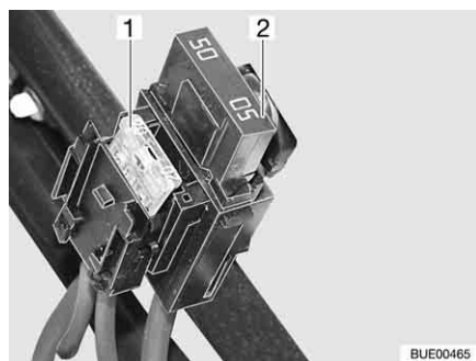
Fig. 168 Fusibili nella batteria di avviamento
