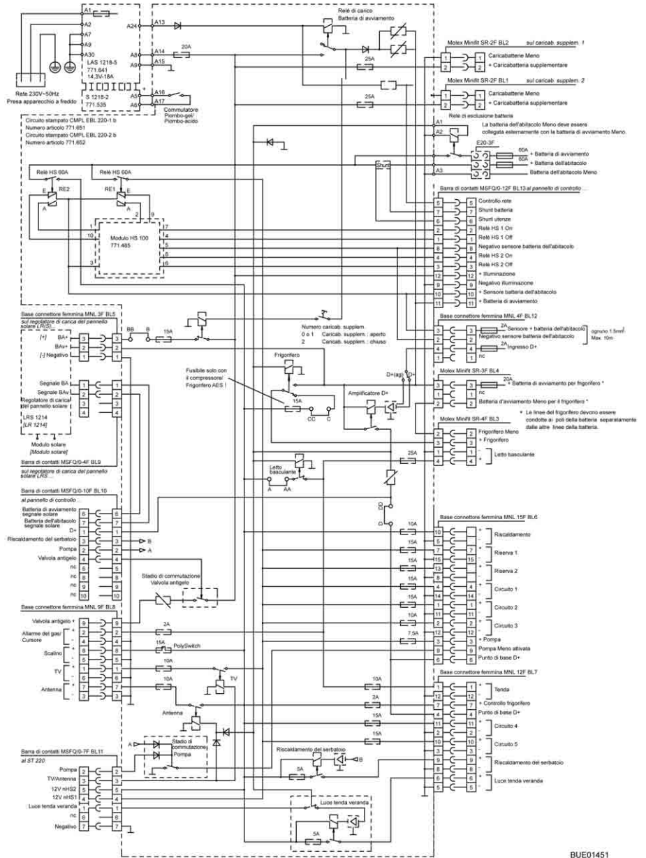
Fig. 181 Schema elettrico interno (EBL 220)
