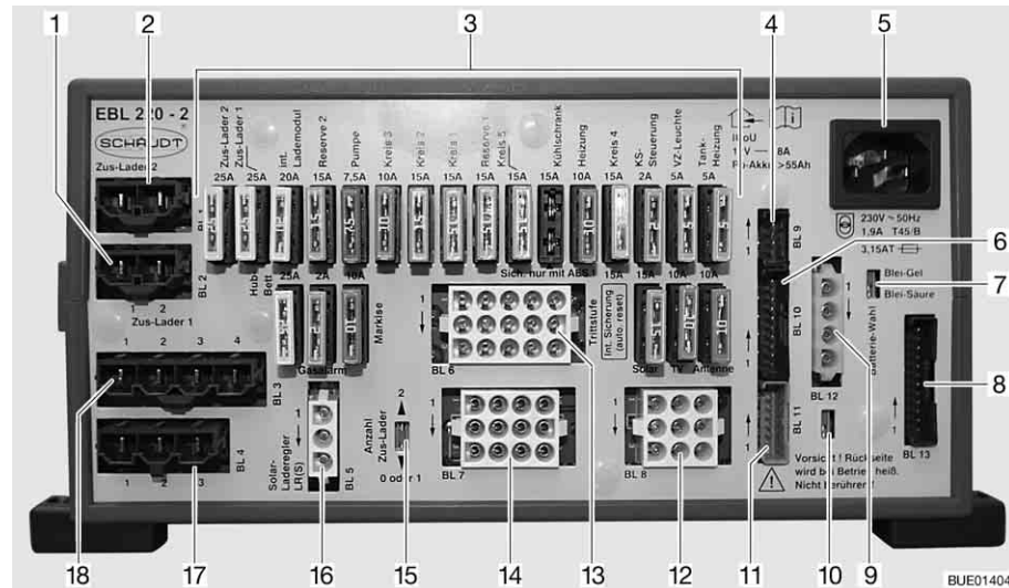
Fig. 155 Centralina elettrica (EBL 220)
