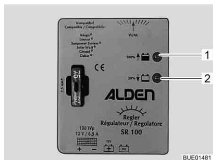
Fig. 163 Regolatore di carica del pannello solare 100 W
