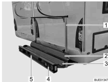
Fig. 7 Porte-charges
