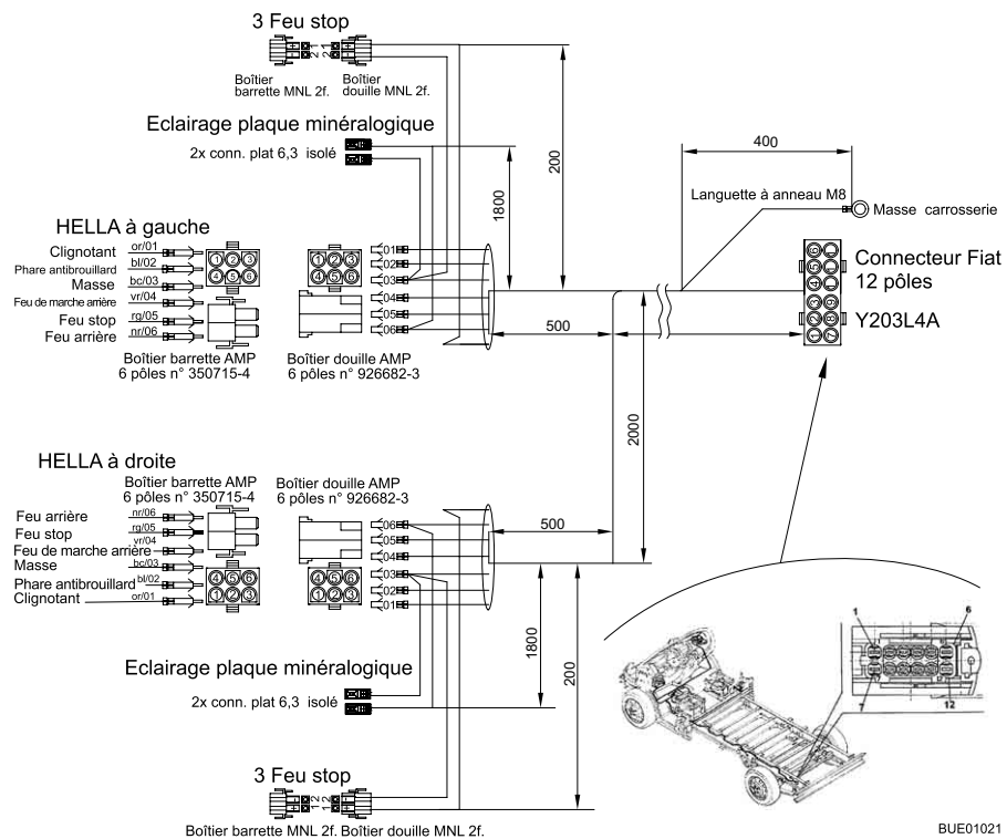
Fig. 184 Schéma électrique extérieur
