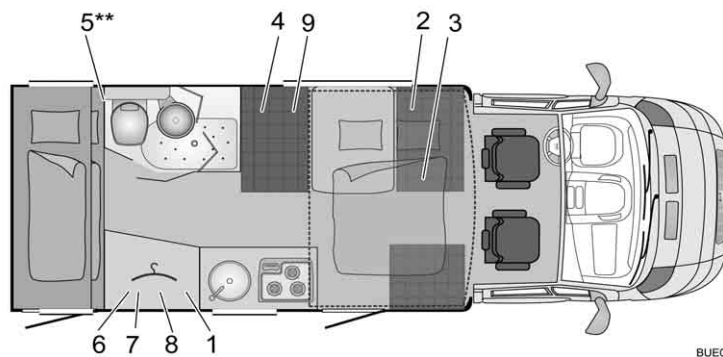
Afb. 307 Plattegrond IT 660 Ixeo Time
