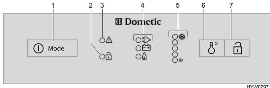
Afb. 220 Bedieningselementen voor de koelkast (Dometic 8-serie met HES)
