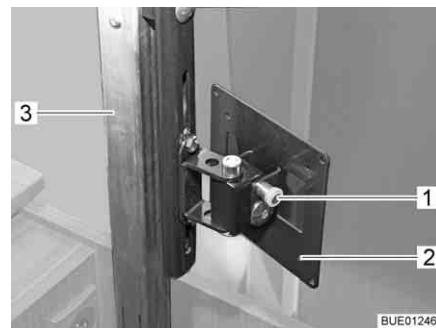
Afb. 63 Hefmechanisme
