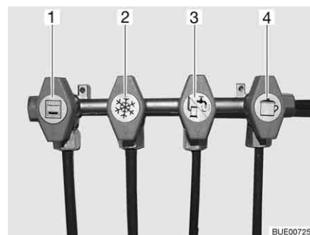
Afb. 185 Symbolen van de gasafsluitkranen
