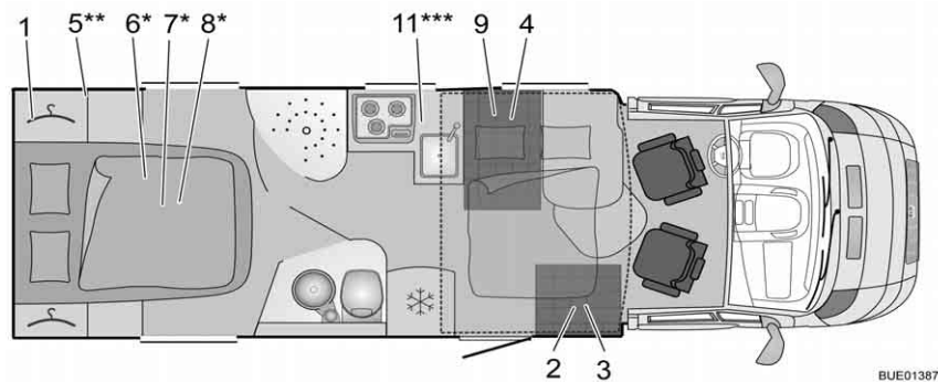
Afb. 323 Plattegrond IT 734 Ixeo Time
