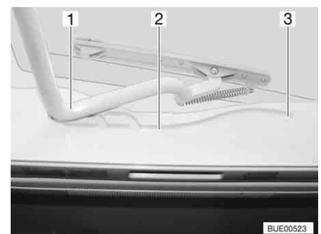
Afb. 77 Heki-dakluik, geleiding
