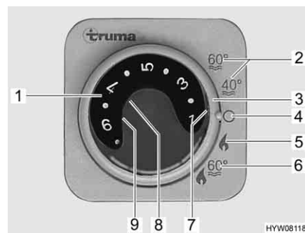
Afb. 187 Bedieningspaneel voor verwarming/boiler
