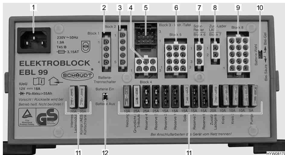
Afb. 160 Elektroblok (EBL 99)
