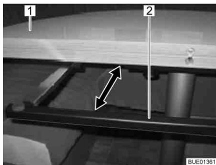
Afb. 96 Steunbeugel
