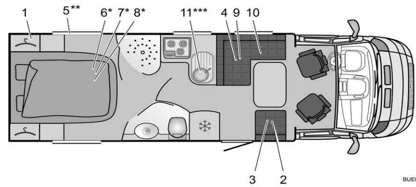
Afb. 319 Plattegrond T 727 Solano/Privilège
