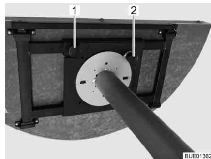
Afb. 97 Vaste tafel (aanzicht van onder)
