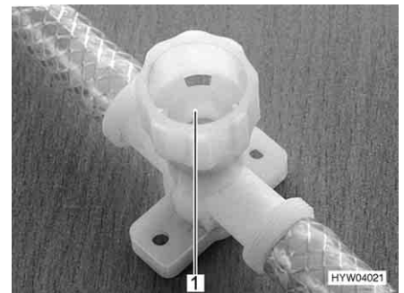
Afb. 237 Aftapkraan (met draaikap)
