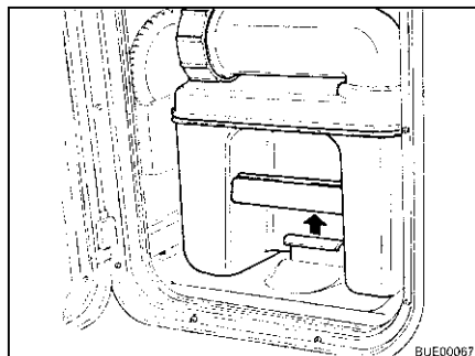
Afb. 240 Bevestigingsbeugel trekken
