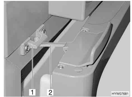
Afb. 228 Koelkastdeur in ventilatiestand (Thetford)
