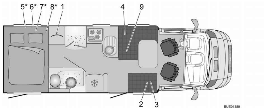
Afb. 325 Plattegrond T 736 Solano/Privilège
