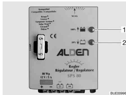
Afb. 166 Zonneregelaar
