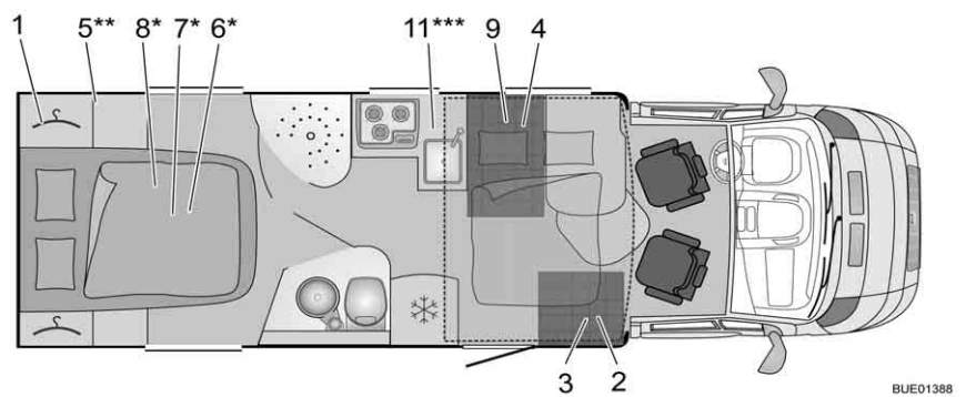
Afb. 324 Plattegrond IT 735 Ixeo
