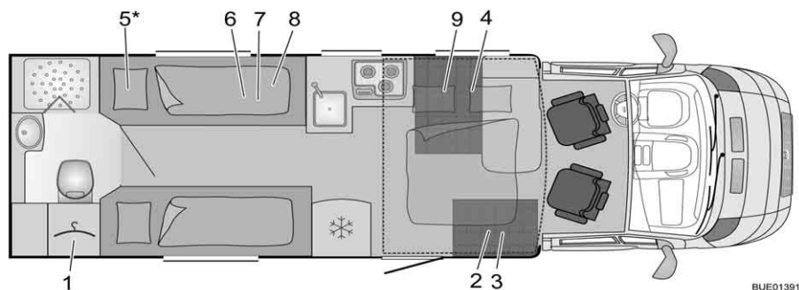
Afb. 327 Plattegrond IT 740 Ixeo
