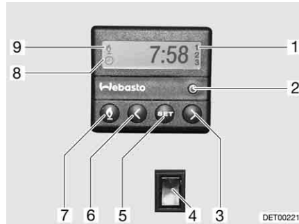
Afb. 199 Bedieningspaneel voor standverwarming
