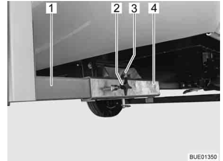
Afb. 8 Bevestiging aan het voertuig
