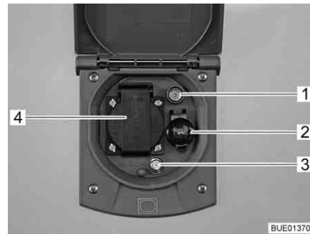
Afb. 178 Buitencontactdoos
