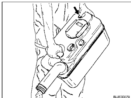
Afb. 275 Fecaliëntank leegmaken
