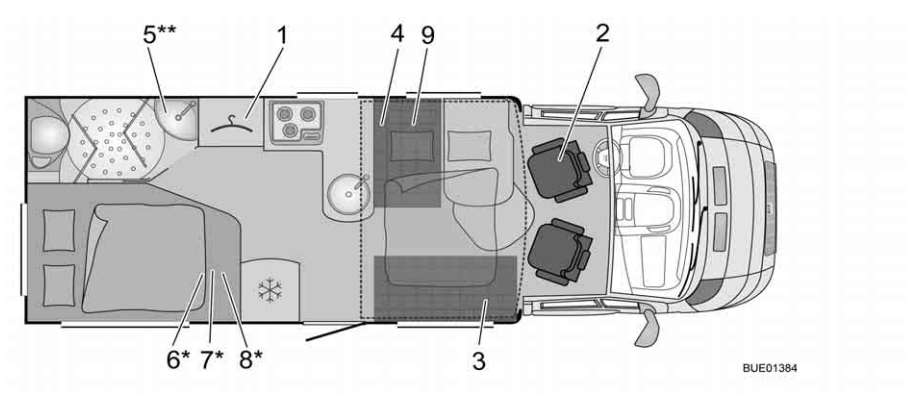
Afb. 312 Plattegrond IT 700 Ixeo
