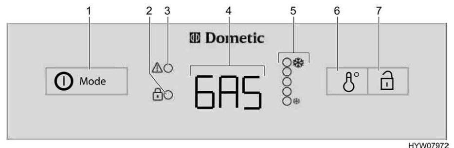
Afb. 221 Bedieningselementen voor de koelkast (Dometic 8-serie met AES)
