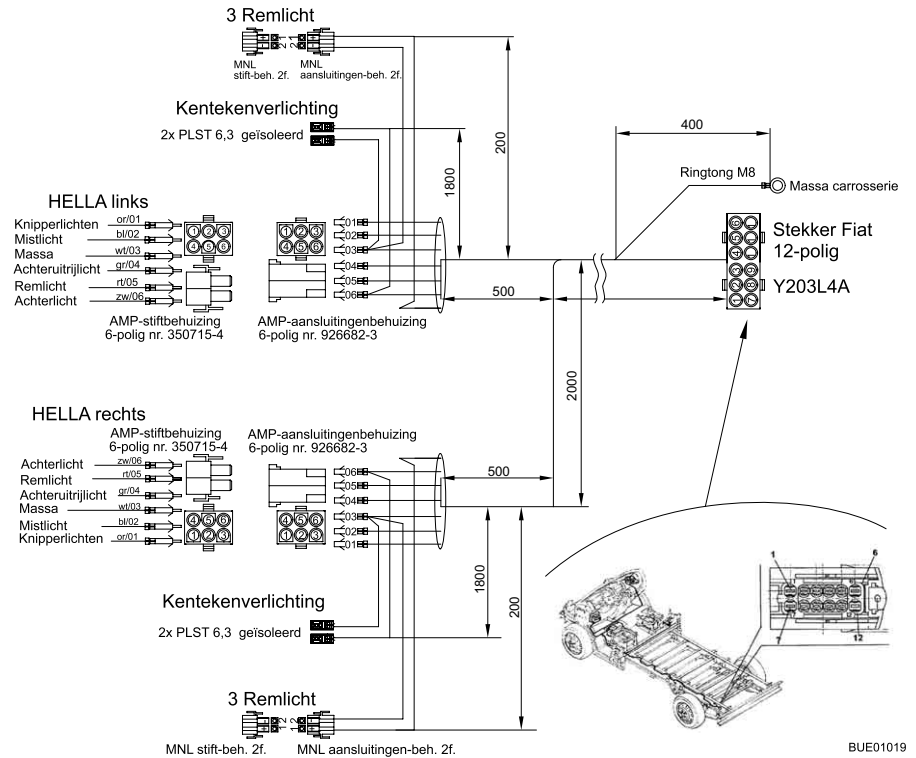
Afb. 184 Stroomschema buiten
