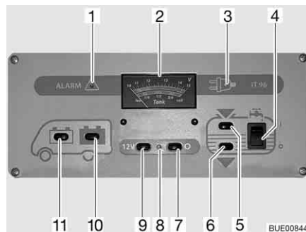
Afb. 161 Paneel IT 96-2
