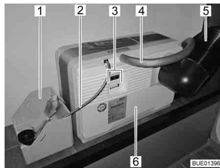
Afb. 163 Brandstofcel met tankpatroon
