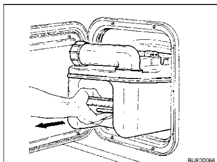
Afb. 252 Thetford-cassette uitnemen
