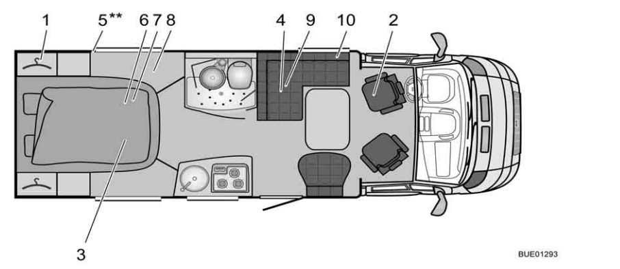
Afb. 311 Plattegrond T 687 Nexxo
