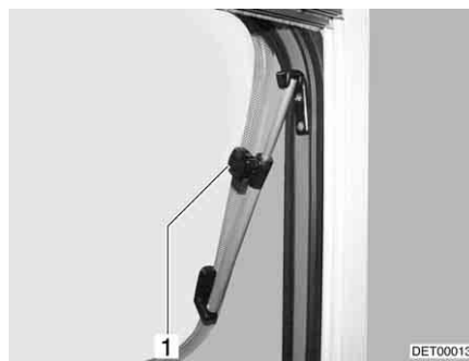
Afb. 65 Uitzetbaar raam met draaibare uitzetters, geopend
