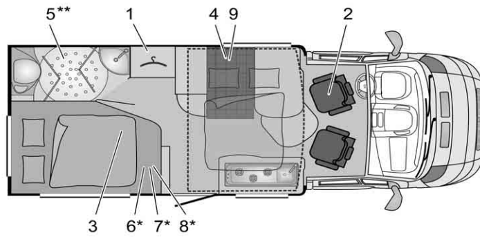
Afb. 305 Plattegrond IT 630 Ixeo Time
