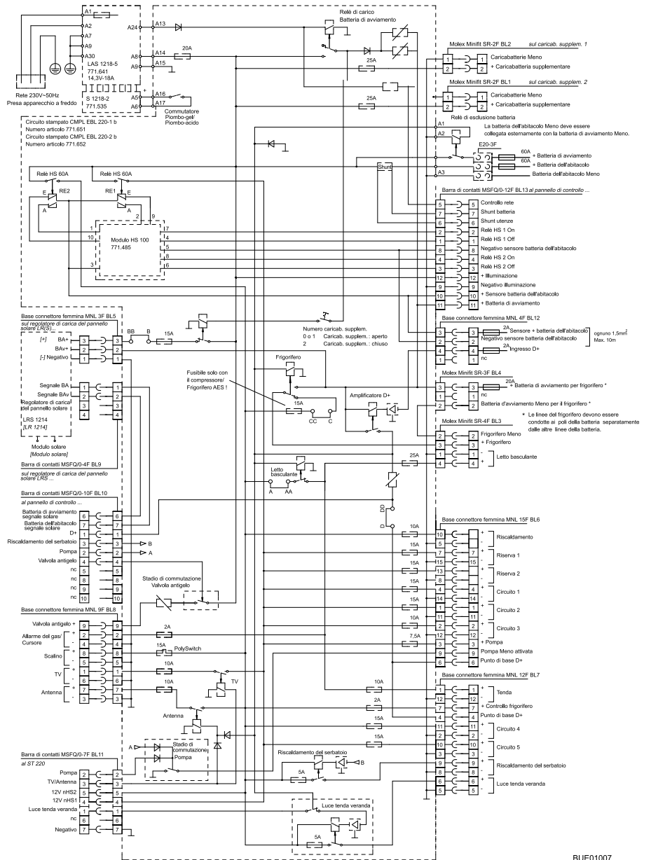
Fig. 157 Schema elettrico interno (EBL 220)
