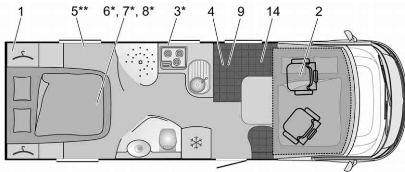
Fig. 291 Pianta I 727 Aviano
