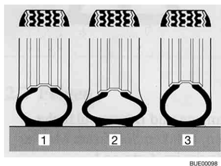
Fig. 279 Base di appoggio dei pneumatici
