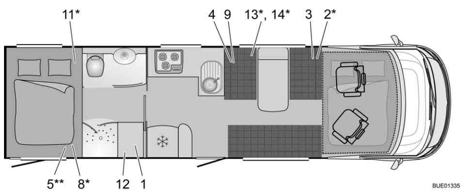
Fig. 299 Pianta I 822 Elegance
