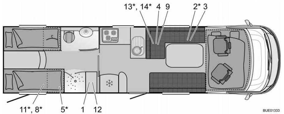
Fig. 296 Pianta I 810 Elegance
