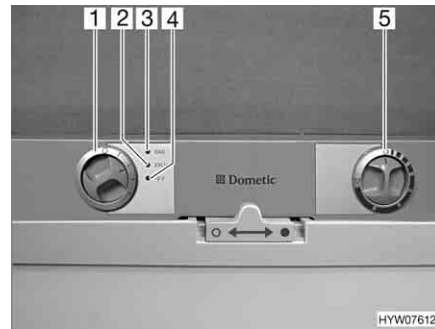
Fig. 192 Elementi di comando per il frigorifero (serie Dometic 7)
