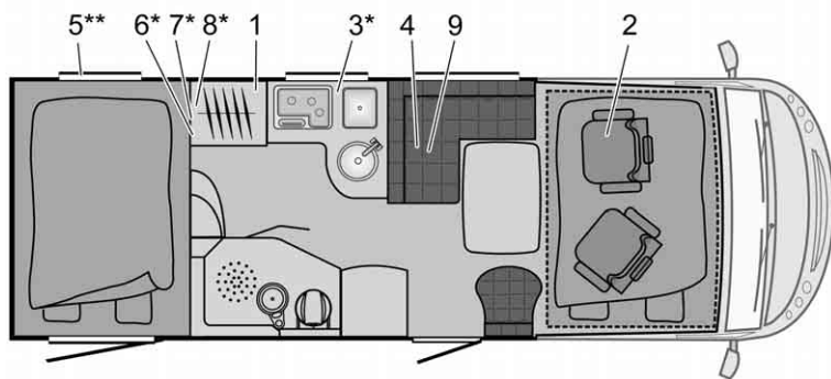
Fig. 285 Pianta I 694 Aviano
