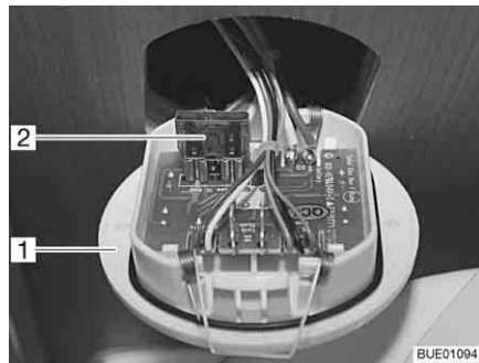
Fig. 149 Fusibile della toilette
