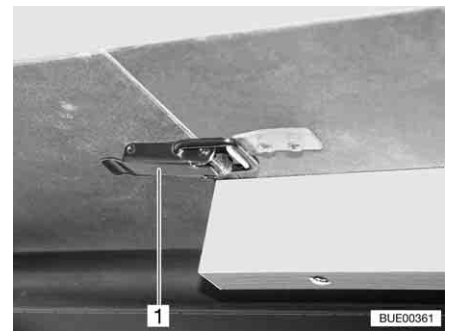
Fig. 92 Cerniera
