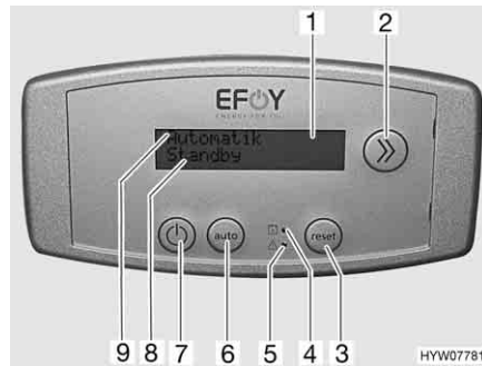
Fig. 140 Centralina di controllo per pila a combustibile
