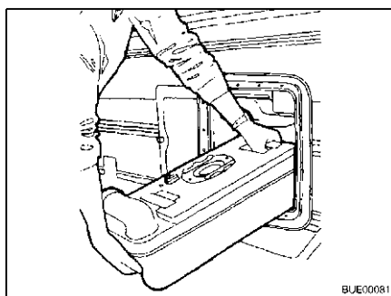
Fig. 231 Cassetta Thetford, rimozione
