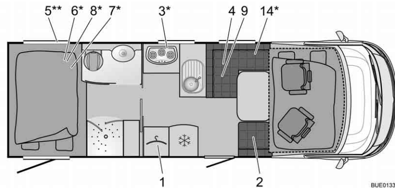
Fig. 293 Pianta I 729 Elegance
