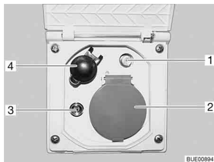
Fig. 153 Presa esterna
