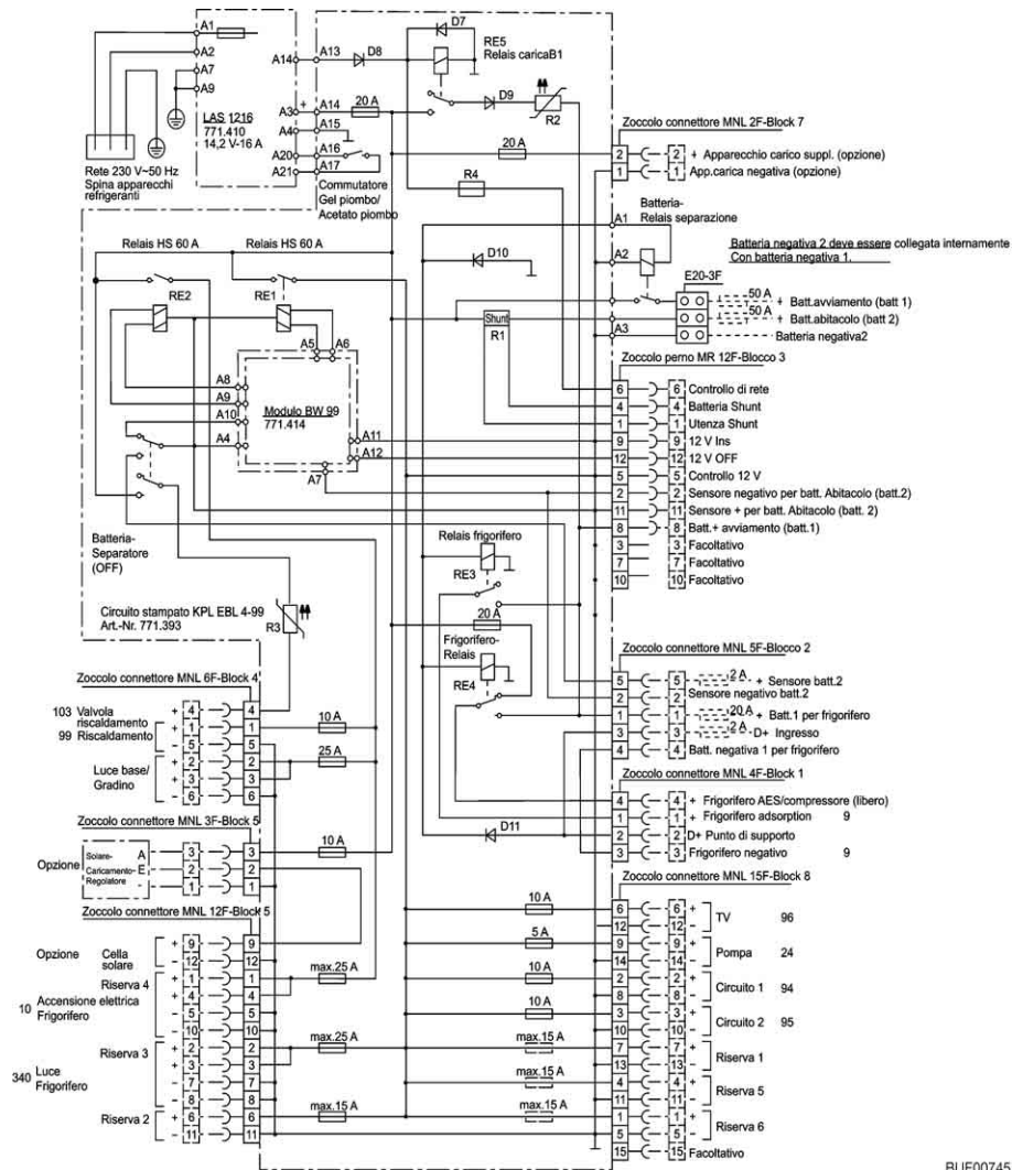
Fig. 156 Schema elettrico interno (EBL 99)
