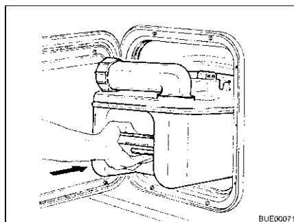
Fig. 229 Inserimento della cassetta Thetford
