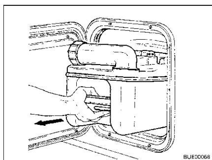
Fig. 226 Cassetta Thetford, rimozione
