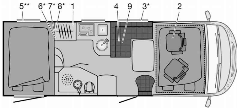
Fig. 284 Pianta I 694 Viséo
