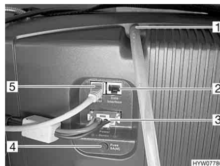
Fig. 139 Campo di collegamento pila a combustibile
