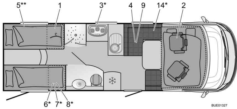
Fig. 290 Pianta I 726 Elegance
