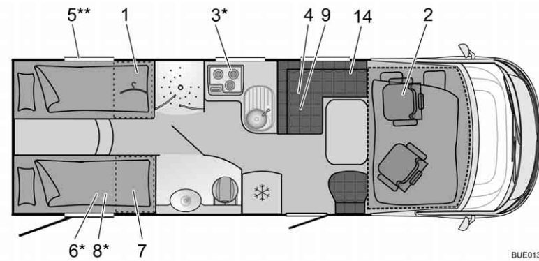
Fig. 292 Pianta I 728 Aviano
