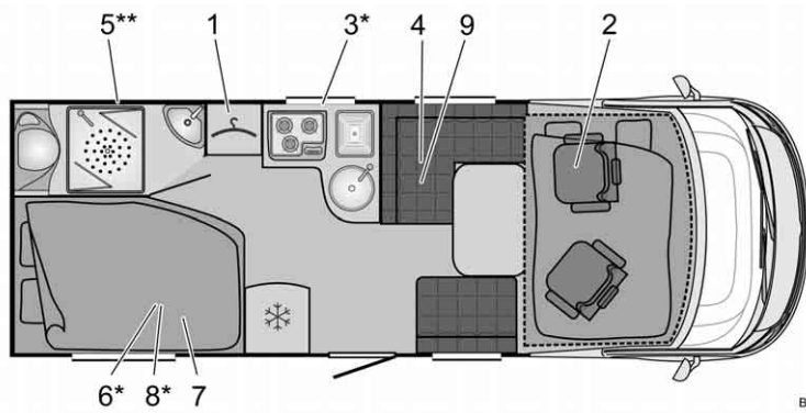
Fig. 283 Pianta I 684 Aviano
