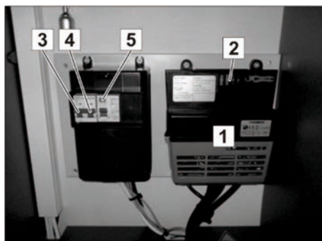
Fig. 63: Omformer (nettapparat) (1) og automatsikringer
