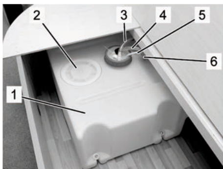
Fig. 88: Ferskvannstank, eksempel
