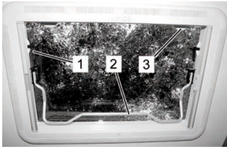
Fig. 121: Betjene løfte-vippetak Heki 2
