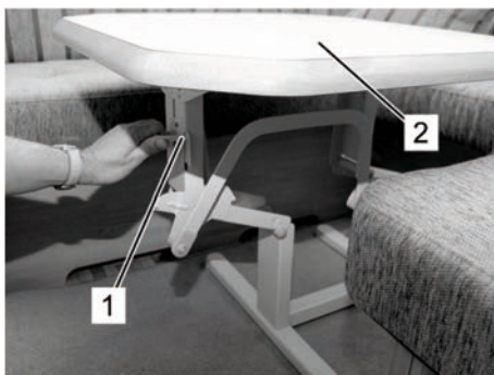
Fig. 134: Bord med løftemekanisme
