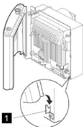
Fig. 126: Oppvarmingspanel svingt ut
