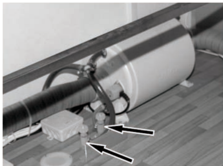
Fig. 131: Tappeventiler
