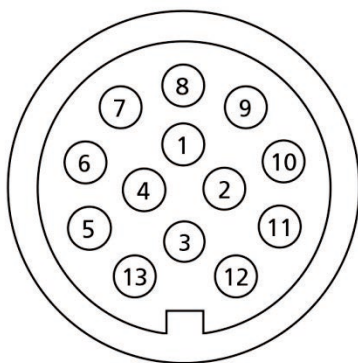
Fig. 2: 13-polet støpsel
