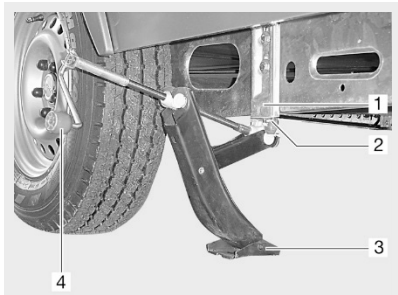
Fig. 160: Jekk AL-KO
