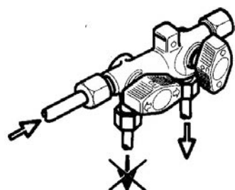
Fig. 82: Stenge- og utløsningsstilling
