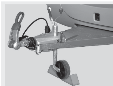
Fig. 139:: Sikre støttehjul
