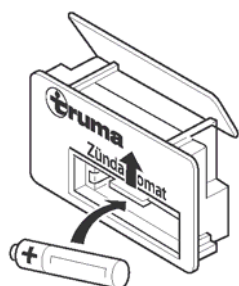
Fig. 109: Udskiftning af batteri
