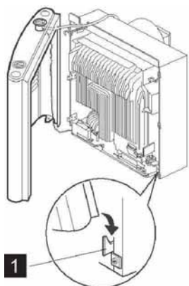
Fig. 108: Varmerens beklædning vippet op
