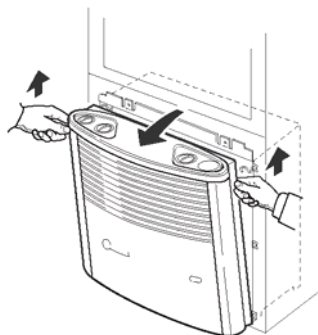
Fig. 107: Vip varmerens beklædning op.
