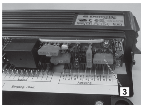
Fig. 57: 12 V-kompletforsyning
