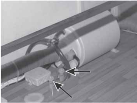
Fig. 82: Truma-vandvarmer og vandafnapningsventiler
