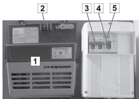
Fig. 55: Omformer (netdel) (1) og sikringsautomater
