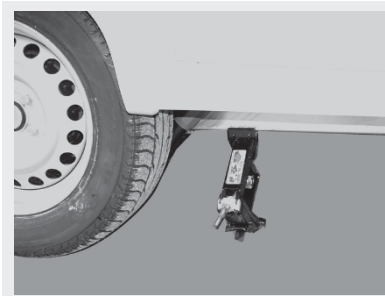
Fig. 141:: Donkraft, normal
