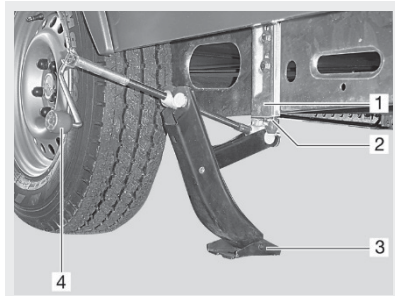
Fig. 142:: Donkraft AL-KO
