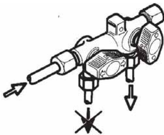
Fig. 71: Afspærrings- og frigivelsesstilling
