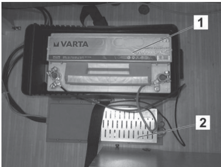
Fig. 58: Autarkpakke
