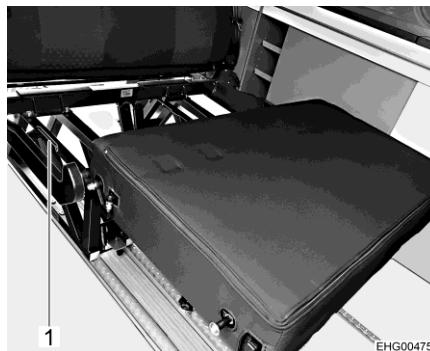
Bild 22 Sitsdel (infälld)
