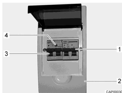
Bild 46 Ledningsskyddsbrytare och FI-brytare (230 V-säkringslåda)
