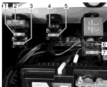
Bild 49 Säkringar för bodelsbatteriet och ytterligare enheter
