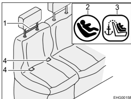
Bild 3 Stöl med Isofix
