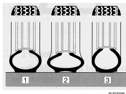
Bild 72 Däckets kontaktyta
