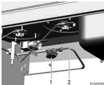
Bild 42 Gasavstängningsventil
