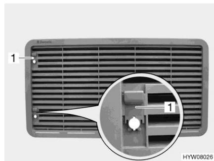
Fig. 183 Grille d'aération du réfrigérateur (avec curseur)
