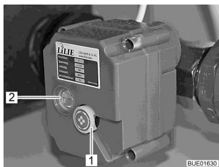
Fig. 198 Robinet de vidange à commande électrique
