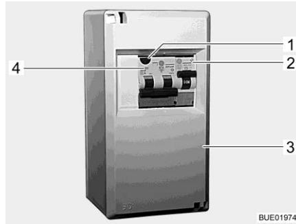
Fig. 142 Coffret de fusibles 230 V avec disjoncteur de protection de circuit et disjoncteur FI
