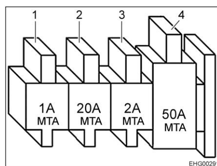
Fig. 147 Fusibles (batterie de cellule avec booster de charge)
