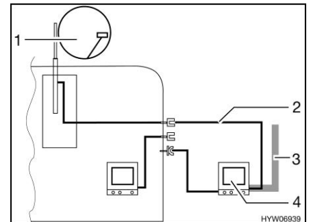
Fig. 152 TV dans l'auvent
