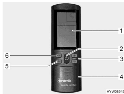
Fig. 170 Télécommande (climatisation)
