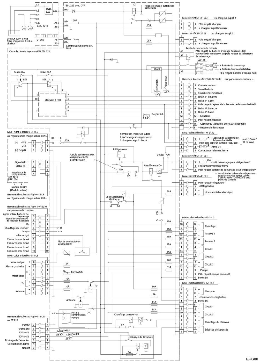
Fig. 153 Schéma électrique intérieur (EBL 223)
