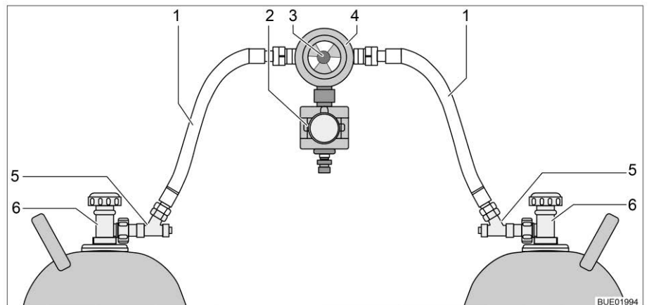
Fig. 22 Régulateur de gaz avec CPU et sécurité de rupture de tuyau
