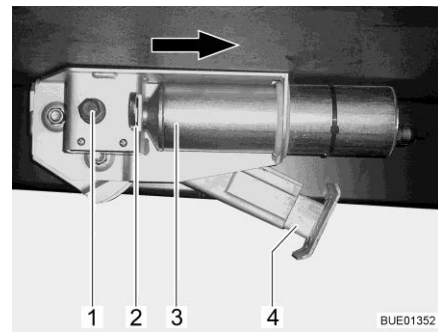
Fig. 52 Vérin stabilisateur électrique sur le véhicule
