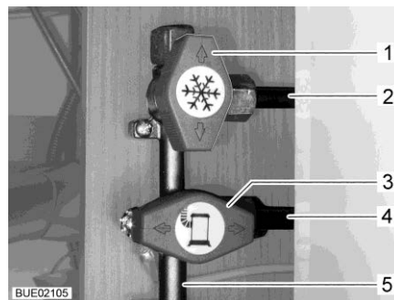
Fig. 130 Position des robinets d'arrêt de gaz (exemple)
