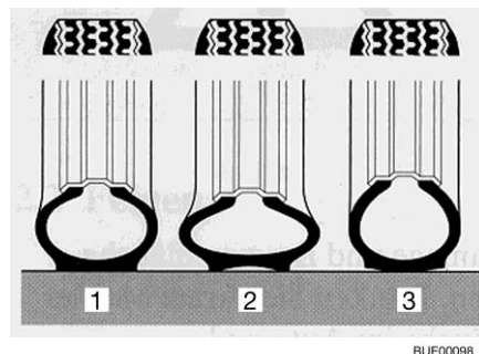
Fig. 232 Surface de contact du pneu
