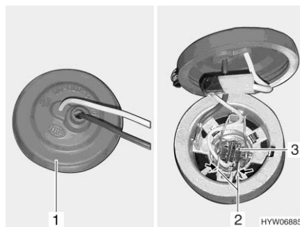
Fig. 220 Projecteur antibrouillard
