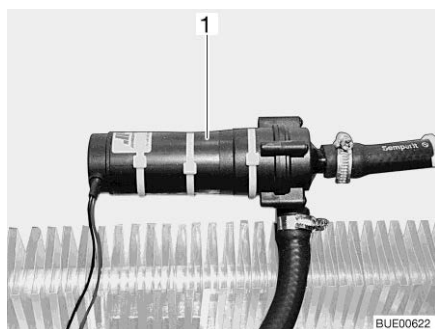
Fig. 163 Circulateur supplémentaire
