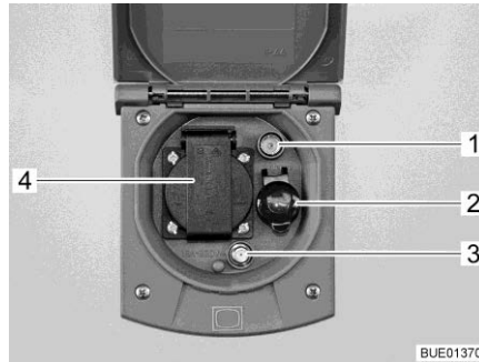
Fig. 150 Prise extérieure
