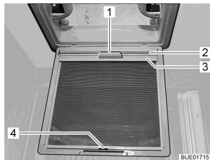
Afb. 63 Verduisteringsrollo (dakluik)
