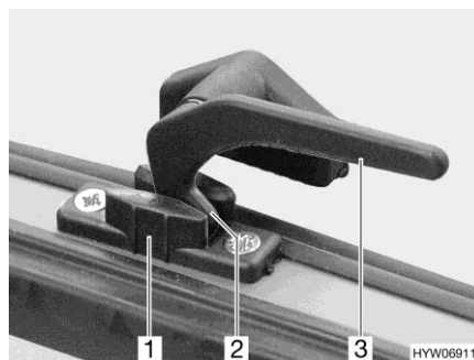
Afb. 56 Vergrendelingshendel (stand "continue ventilatie")
