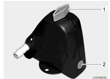
Afb. 139 Veiligheids-/aftapventiel gesloten
