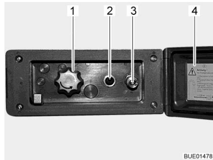
Afb. 86 Doucheaansluiting buiten
