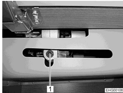
Afb. 80 Toegang tot de aandrijving
