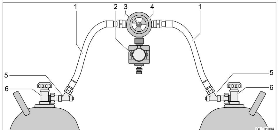
Afb. 13 Gasdrukregelaar met CPU en slangbreukbeveiliging
