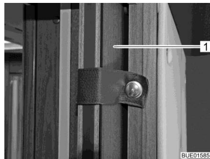
Afb. 11 Schuifdeur
