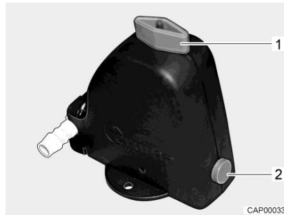
Afb. 138 Veiligheids-/aftapventiel geopend
