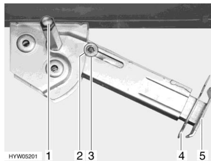
Afb. 26 Hefsteun
