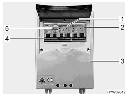
Afb. 100 Beveiligingsautomaat en FI-schakelaar (230-V-zekeringenkast)
