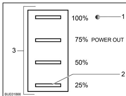
Afb. 99 Statusweergave zonneregelaar
