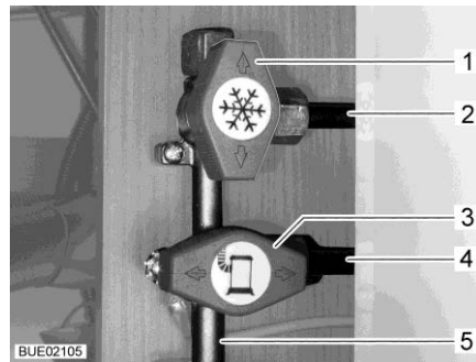
Afb. 88 Stand gasafsluitkranen (voorbeeld)
