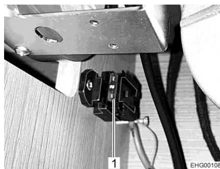
Afb. 106 Zekering hefbed (Ixeo T)
