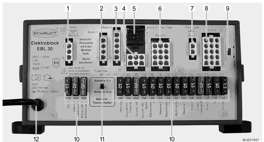
Afb. 97 Elektroblok (EBL 30)
