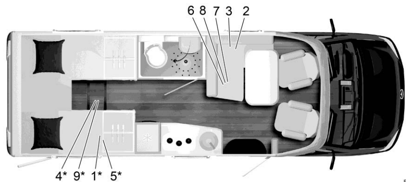
Afb. 175 Plattegrond Lyseo M 690G
