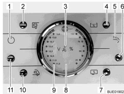
Afb. 98 Paneel LT 96
