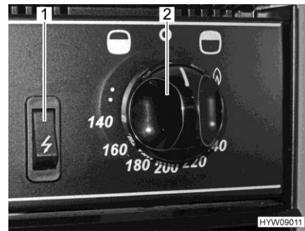
Afb. 130 Bedieningselementen (gasbakoven met grill)
