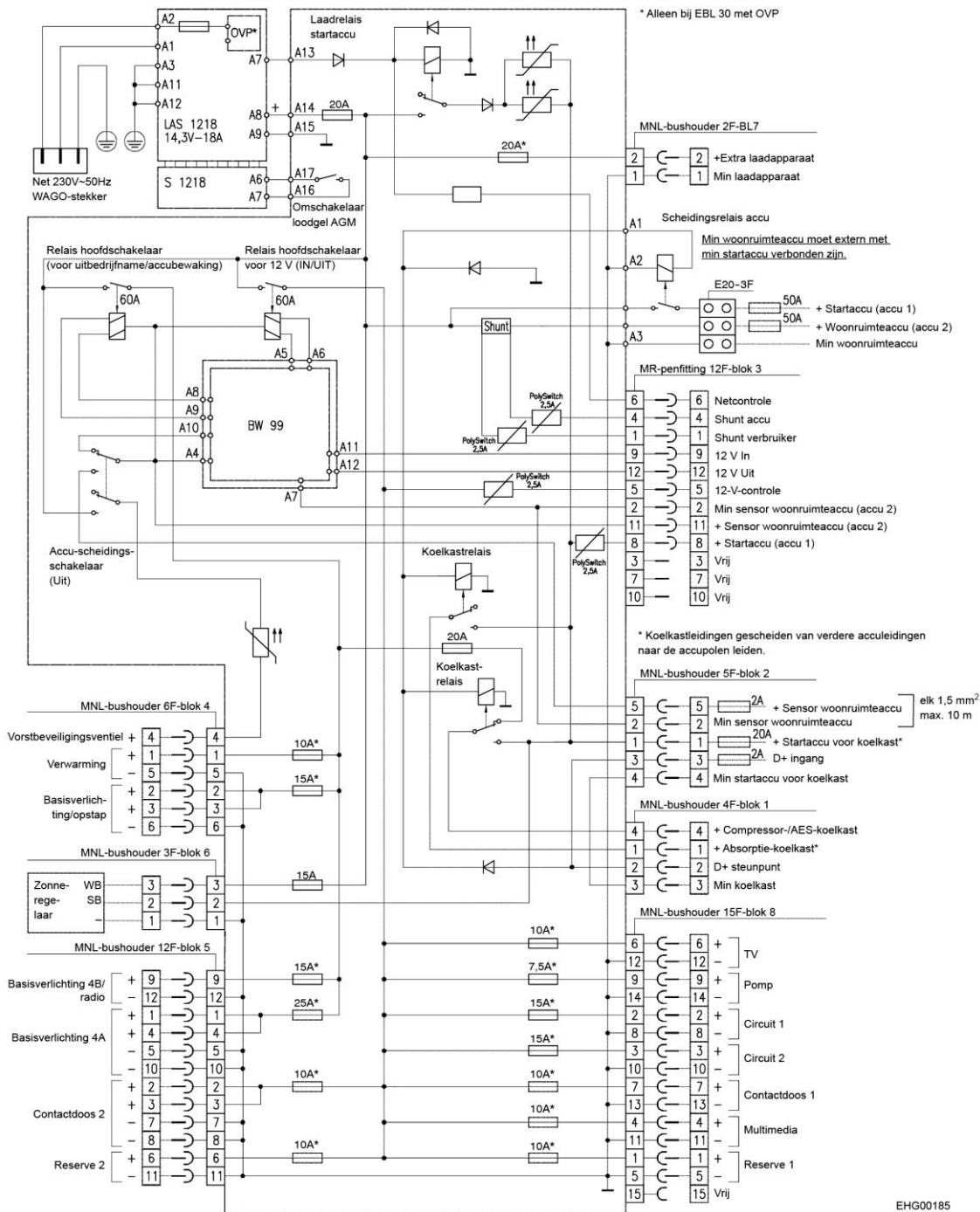
Afb. 111 Stroomschema binnen (EBL 30)
