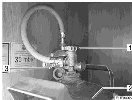
Afb. 94 Gaskast
