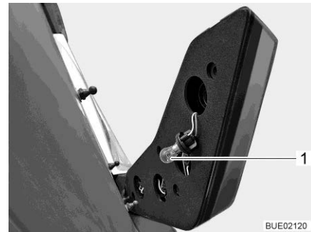
Afb. 164 Achterlicht
