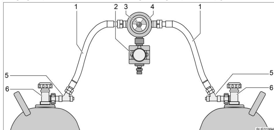
Afb. 91 Omschakelinstallatie voor gasflessen met CPU
