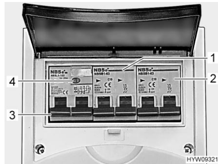
Afb. 107 Beveiligingsautomaat en FI-schakelaar (230-V-zekeringenkast)
