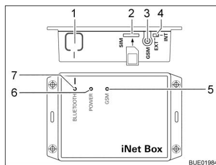
Afb. 127 Truma iNet-Box
