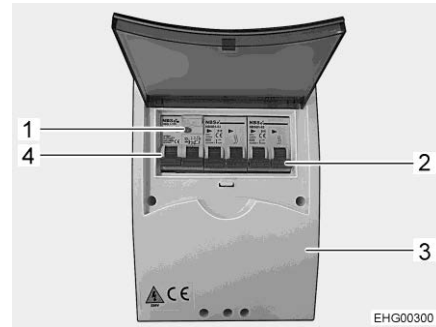
Afb. 197 230-V-zekeringenkast (variant)
