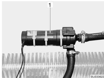
Afb. 218 Extra circulatiepomp
