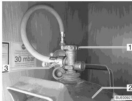
Afb. 176 Gaskast
