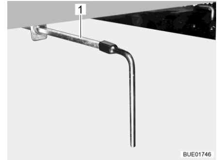
Afb. 263 Aftapkraan
