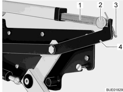
Afb. 142 Aandrijving voor hefbed
