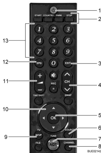
Afb. 61 Afstandsbediening
