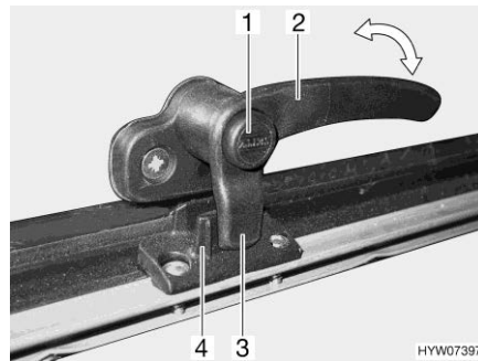
Afb. 109 Vergrendelingshendel met vergrendelingsknop in stand "gesloten"
