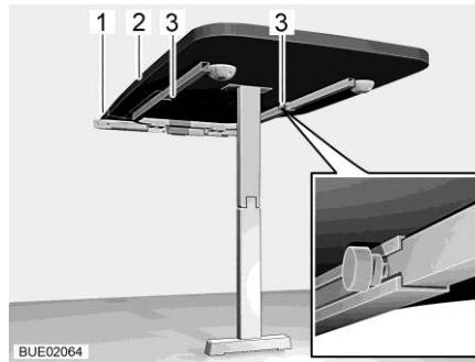
Afb. 134 Hangtafel met scharnier-steunpoot
