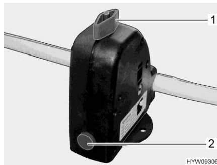
Afb. 211 Veiligheids-/aftapventiel (boiler)
