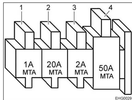
Afb. 193 Zekeringen (woonruimteaccu met laadbooster)
