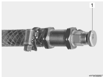
Afb. 284 Ontluchtingsventiel warmwaterverwarming
