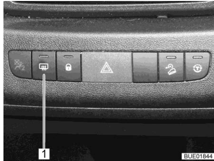
Afb. 41 Schakelaar buitenspiegelverwarming
