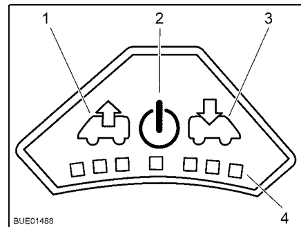
Afb. 128 Bedieningsveld van de ventilator
