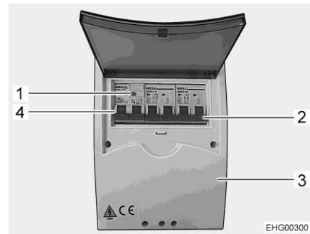
Afb. 187 230-V-zekeringenkast (variant)
