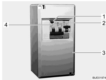
Afb. 186 230-V-zekeringenkast
