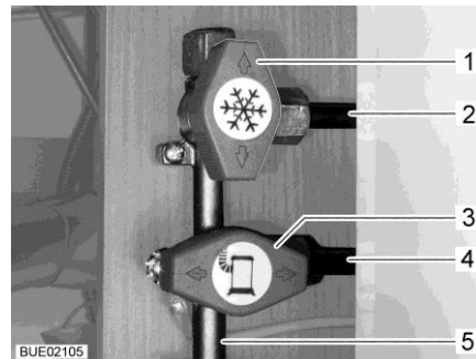
Afb. 170 Stand gasafsluitkranen (voorbeeld)
