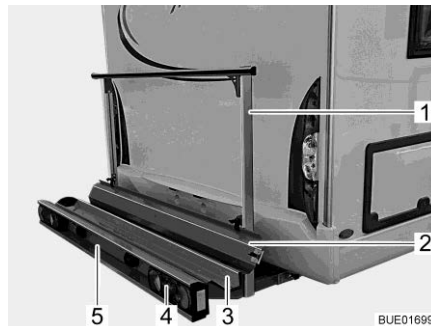
Afb. 6 Lastdrager
