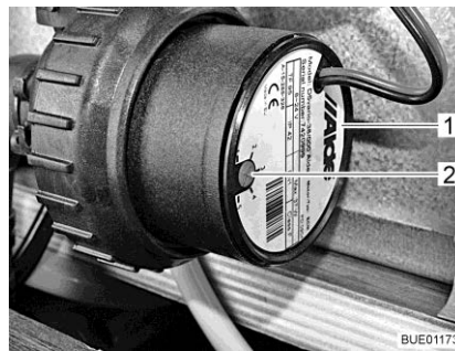
Afb. 215 Toerentalverlaging
