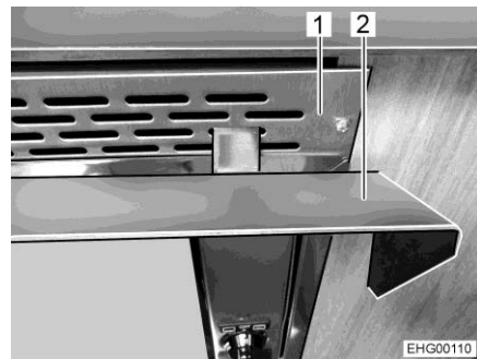
Afb. 233 Hittescherm (ingehangen)
