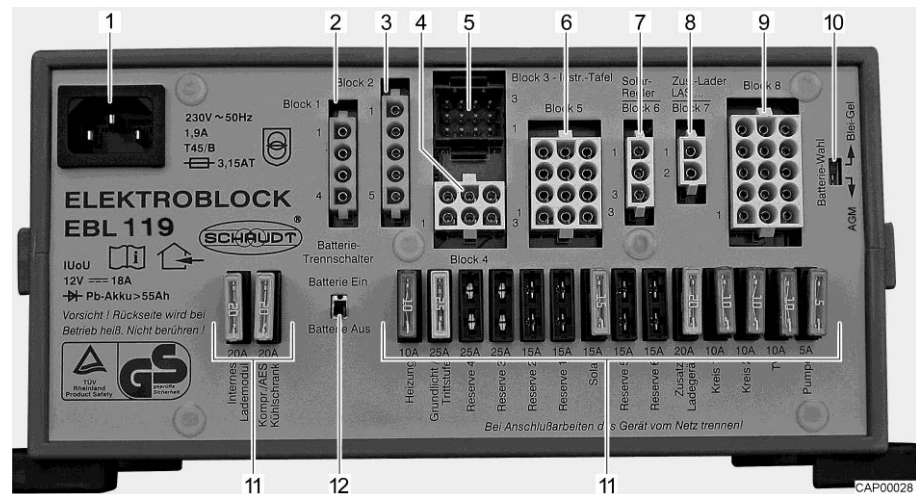
Afb. 181 Elektroblok (EBL 119)
