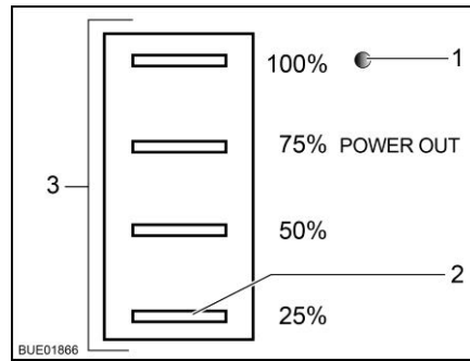
Afb. 185 Statusweergave zonnere-gelaar
