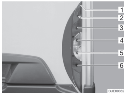
Fig. 187 Eclairage arrière
