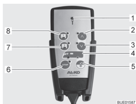
Fig. 15 Télécommande
