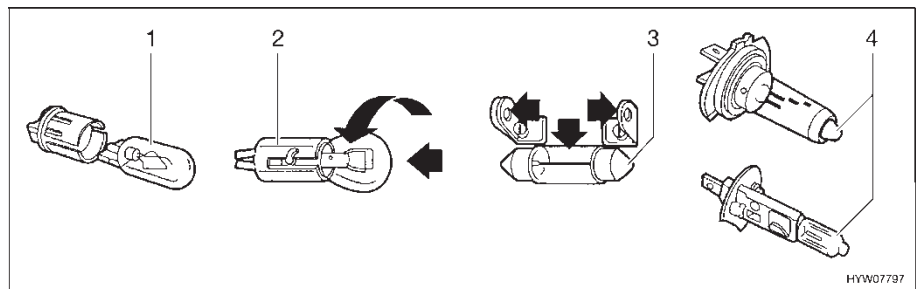
Fig. 186 Types d'ampoules
