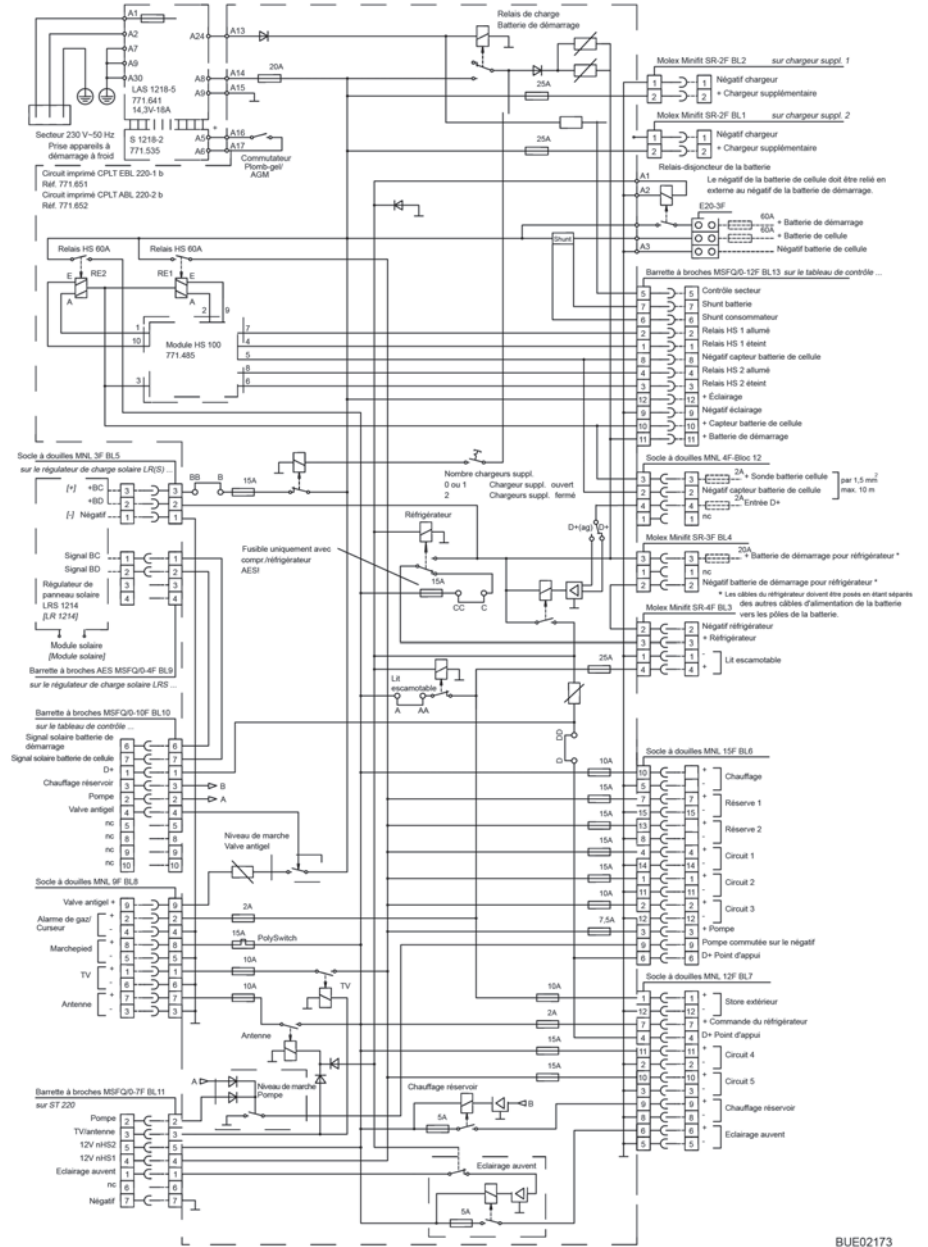
Fig. 131 Schéma électrique intérieur (EBL 223)
