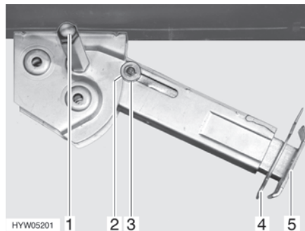
Fig. 25 Vérin stabilisateur
