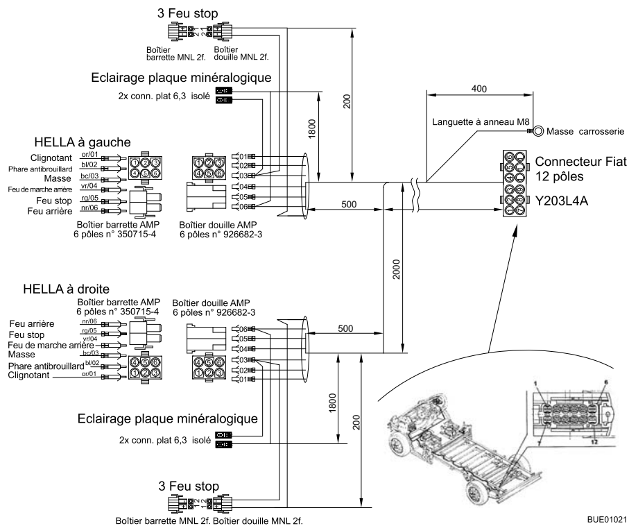
Fig. 133 Schéma électrique extérieur
