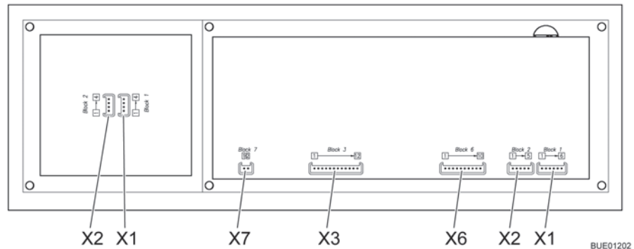
Fig. 132 Schéma fonctionnel, panneau de contrôle (LT 511)
