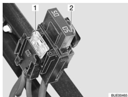
Afb. 144 Zekeringen aan de startaccu
