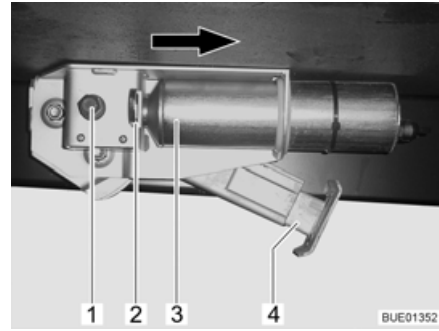
Afb. 51 Elektrische hefsteun aan het voertuig
