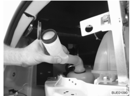
Afb. 43 Vulopening in vulpositie
