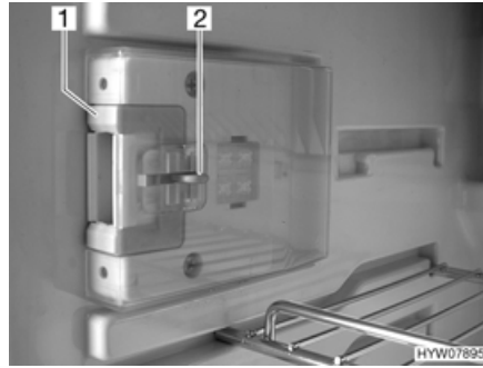
Afb. 187 Sluiting (normale stand)
