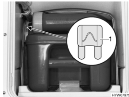
Afb. 146 Zekering van het Thetford-toilet
