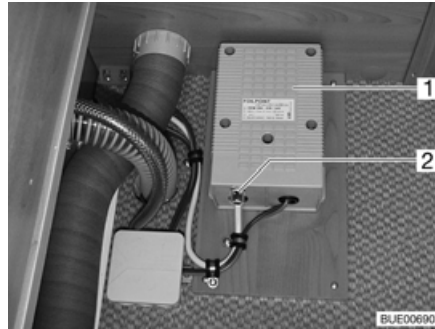
Afb. 166 Transformator voor de elektrische vloerverwarming
