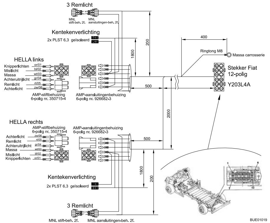
Afb. 153 Stroomschema buiten
