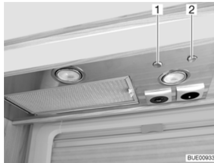
Afb. 179 Afzuigkap
