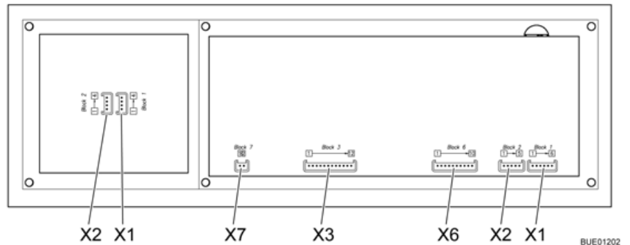
Afb. 152 Blokschema paneel (LT 511)
