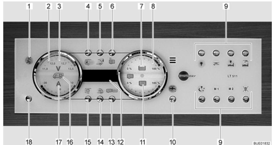
Afb. 139 Paneel LT 511
