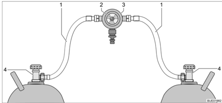
Afb. 131 Omschakelinstallatie voor gasflessen
