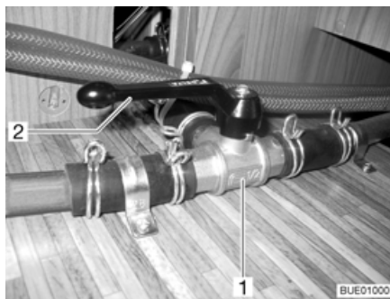
Afb. 159 3-wegventiel
