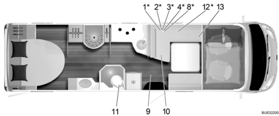
Afb. 233 Plattegrond I 920 G Elegance
