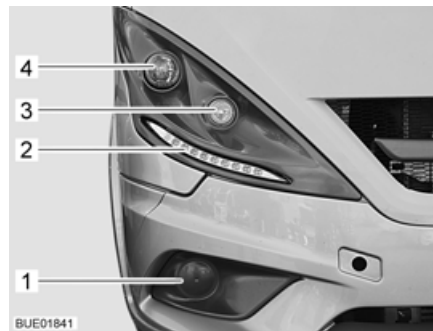
Afb. 215 Verlichting front
