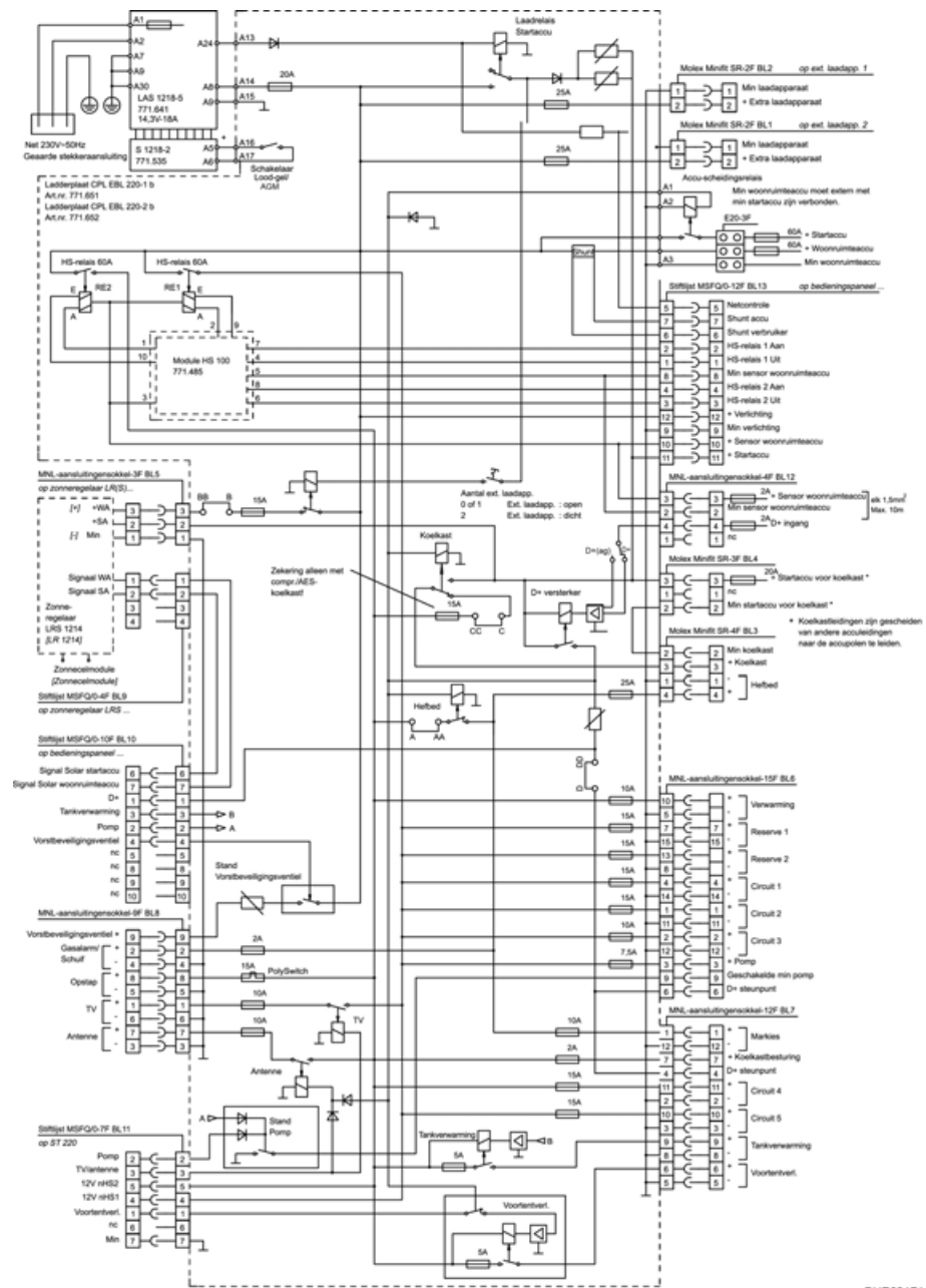
Afb. 151 Stroomschema binnen (EBL 223)
