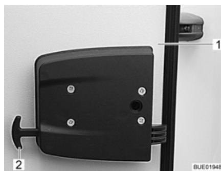
Afb. 67 Noodontgrendeling garageluik
