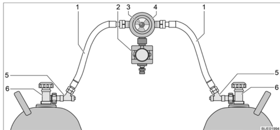
Afb. 132 Omschakelinstallatie voor gasflessen met CPU
