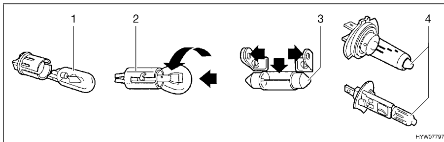
Afb. 214 Gloeilamptypen
