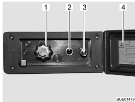
Afb. 127 Doucheaansluiting buiten
