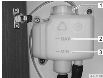
Afb. 212 Buffertank zonder afscherming
