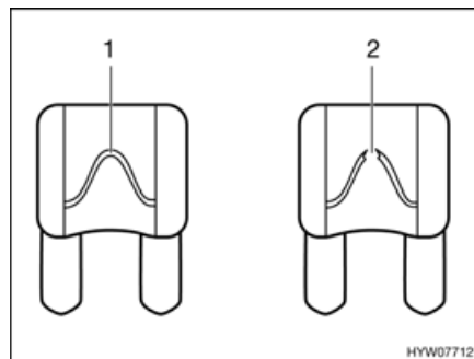
Afb. 143 Zekering 12 V
