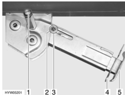
Afb. 48 Hefsteun
