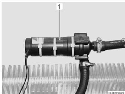
Afb. 161 Extra circulatiepomp
