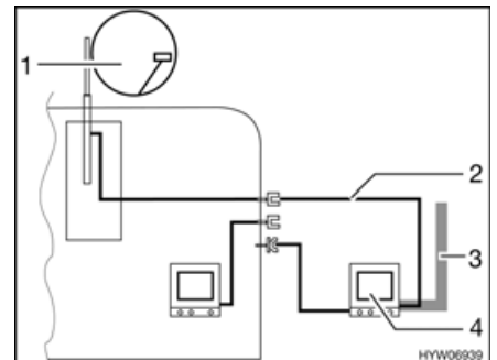
Afb. 150 TV in de voortent
