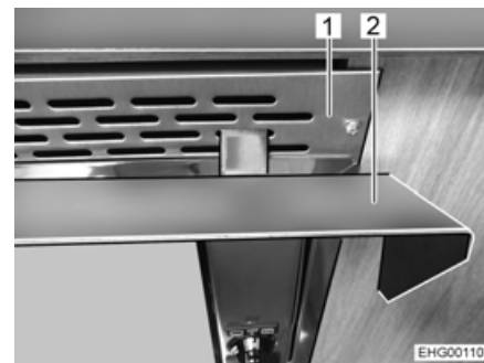
Afb. 175 Hittescherm (ingehangen)
