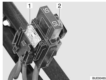
Fig. 143 Fusibili nella batteria di avviamento
