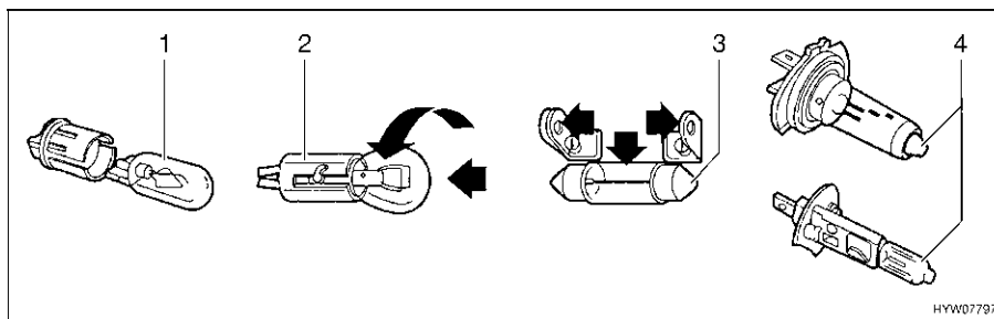
Fig. 236 Tipi di lampade ad incandescenza
