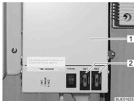
Fig. 147 Regolatore riscaldamento per tubazioni delle acque grigie
