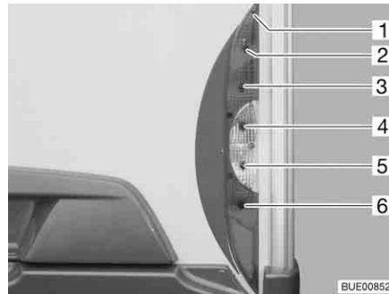
Fig. 237 Luci posteriori
