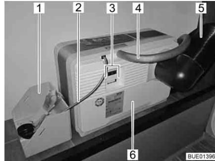
Fig. 135 Pila a combustibile con cartuccia del serbatoio
