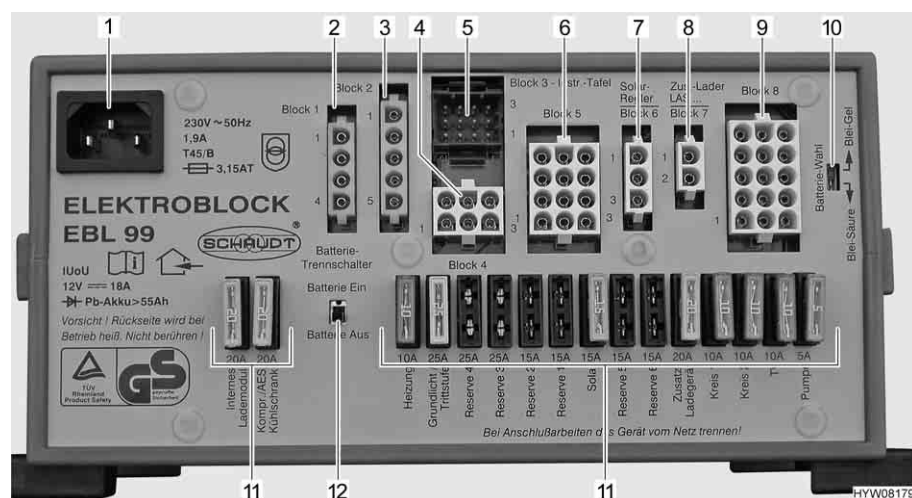
Fig. 131 Centralina elettrica (EBL 99)
