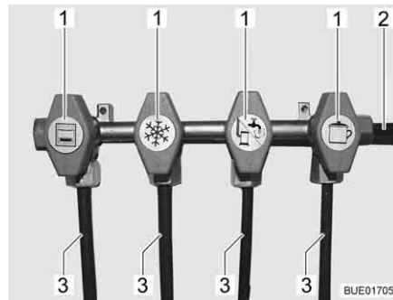
Fig. 123 Posizione dei rubinetti di arresto del gas (esempio)
