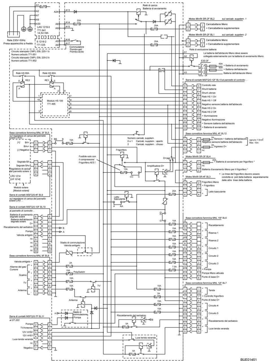
Fig. 156 Schema elettrico interno (EBL 220)
