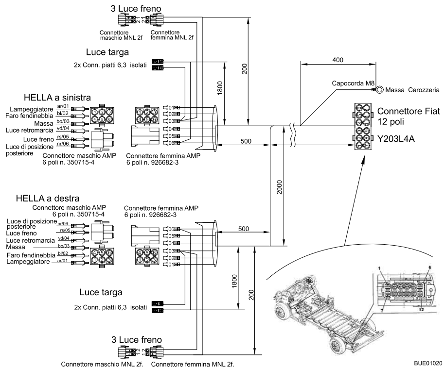
Fig. 159 Schema elettrico esterno
