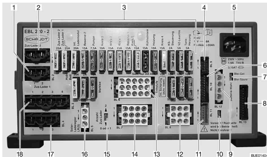
Fig. 132 Centralina elettrica (EBL 220)
