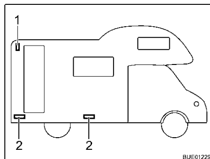
Fig. 238 Luci laterali
