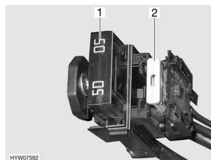
Fig. 144 Fusibili nella batteria dell'abitacolo
