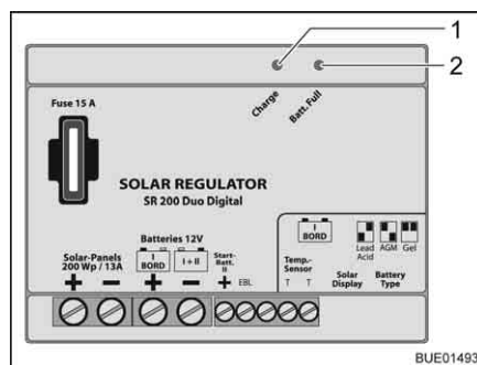
Fig. 139 Regolatore di carica del pannello solare 140/200 W
