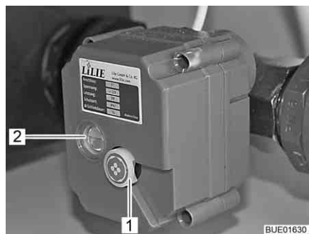
Fig. 212 Rubinetto di scarico ad azionamento elettrico
