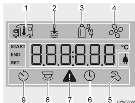
Afb. 143 Display
