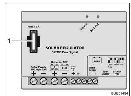
Afb. 117 Zekering zonneregelaar 140/200 W
