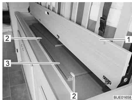
Afb. 82 Bedverbreding, vergrendeld
