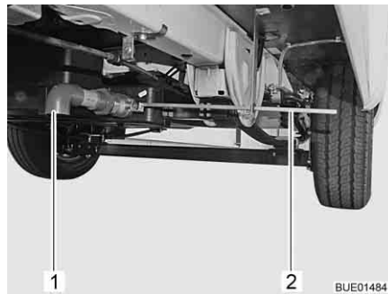
Afb. 160 Aftapkraan
