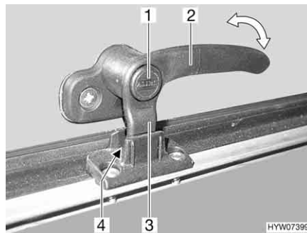
Afb. 59 Vergrendelingshendel met vergrendelingsknop in stand "continue ventilatie"
