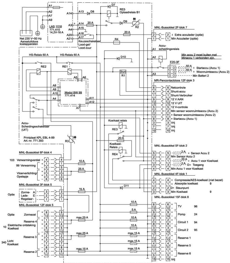
Afb. 122 Stroomschema binnen (EBL 99)
