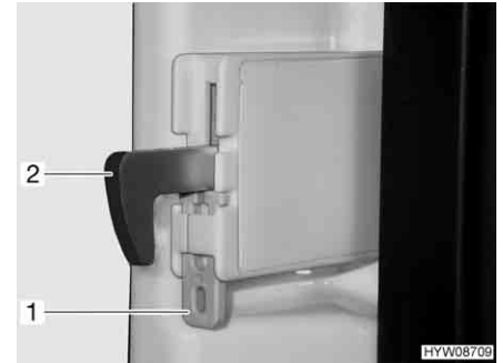
Afb. 150 Vastzetten vergrendelingshaak
