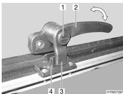
Afb. 51 Vergrendelingshendel met vergrendelingsknop in stand "gesloten"
