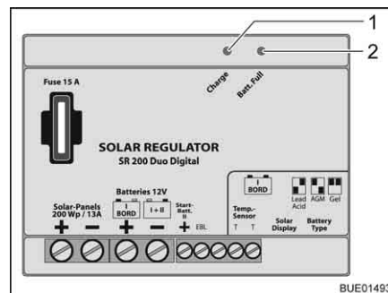
Afb. 107 Zonneregelaar 140/200 W
