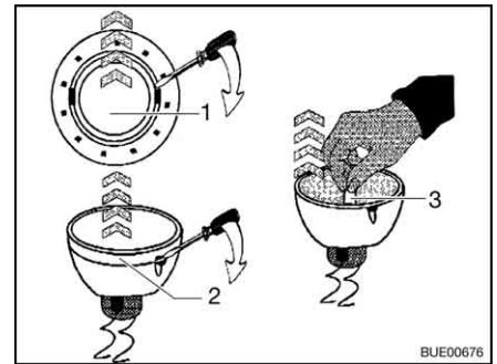
Fig. 269 Sostituire la lampada alogena ad incandescenza
