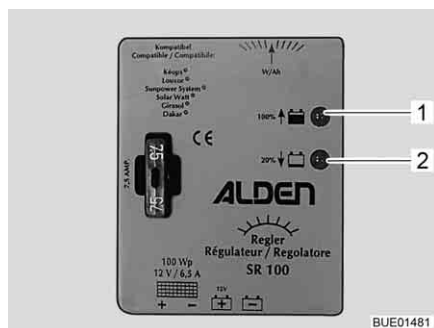
Fig. 158 Regolatore di carica del pannello solare 100 W
