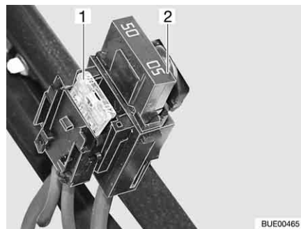
Fig. 163 Fusibili nella batteria di avviamento
