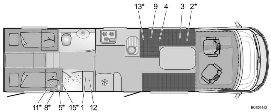
Fig. 289 Pianta I 810 G Elegance
