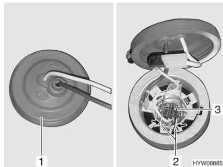
Fig. 261 Luce fendinebbia
