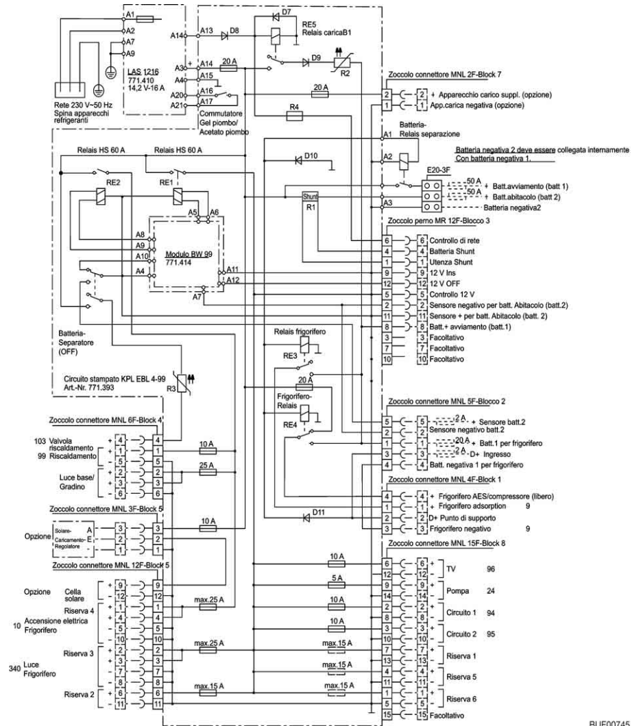
Fig. 176 Schema elettrico interno (EBL 99)
