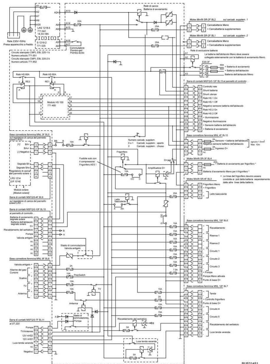
Fig. 177 Schema elettrico interno (EBL 220)
