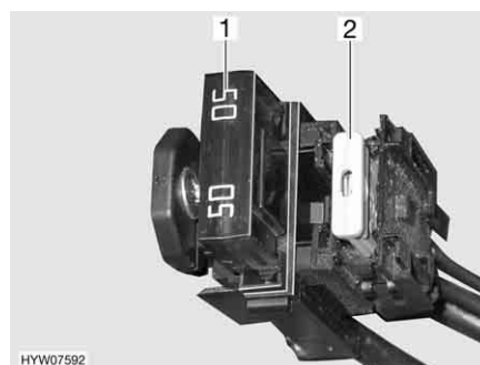
Fig. 164 Fusibili nella batteria dell'abitacolo
