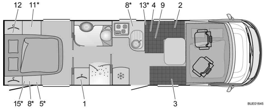
Fig. 292 Pianta I 870 G Aviano
