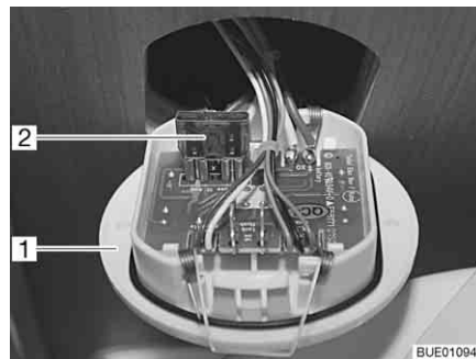
Fig. 167 Fusibile della toilette
