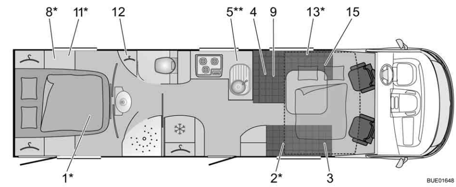
Fig. 295 Pianta I 920 G Grand Panorama
