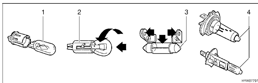
Fig. 257 Tipi di lampade ad incandescenza
