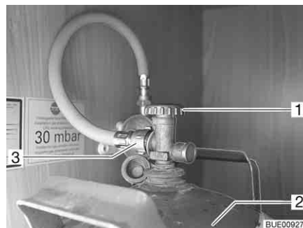
Fig. 140 Vano portabombole
