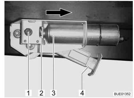
Fig. 51 Piedino di stazionamento elettrico sul veicolo
