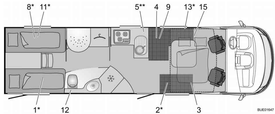
Fig. 294 Pianta I 915 G Grand Panorama
