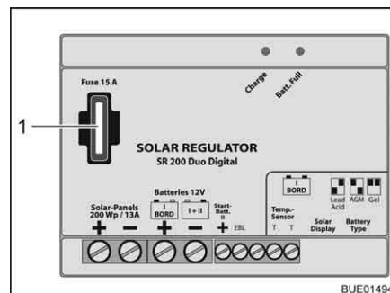
Fig. 171 Fusibile regolatore di carica del pannello solare 200 W
