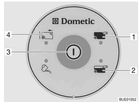
Fig. 250 Centralina di controllo e di comando della toilette
