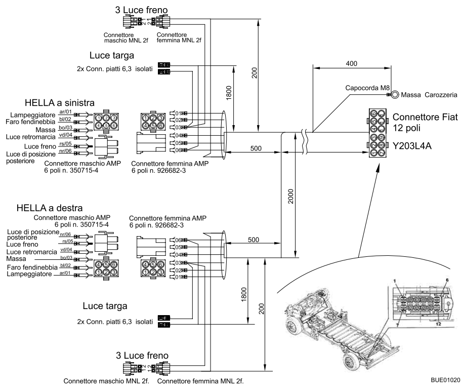
Fig. 182 Schema elettrico esterno
