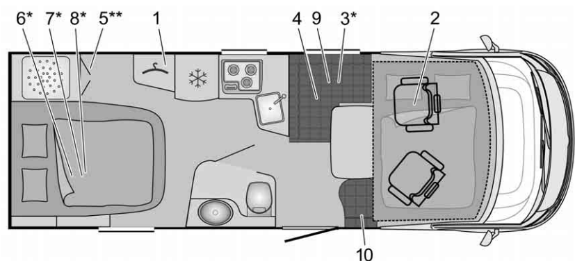
Fig. 283 Pianta I 695 Aviano
