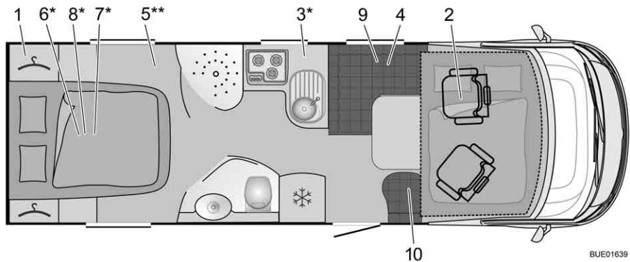
Fig. 286 Pianta I 727 Aviano
