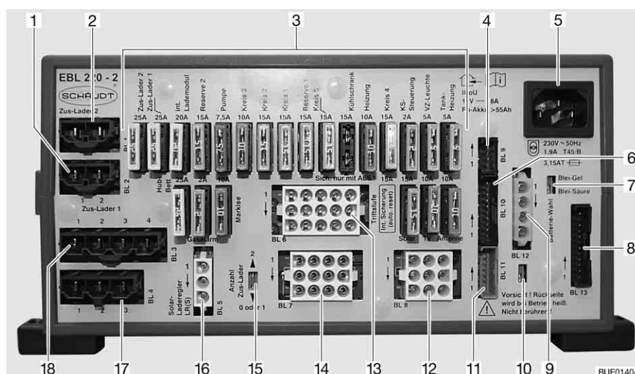
Fig. 150 Centralina elettrica (EBL 220)
