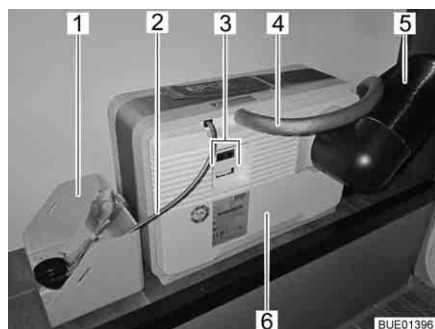
Fig. 155 Pila a combustibile con cartuccia del serbatoio
