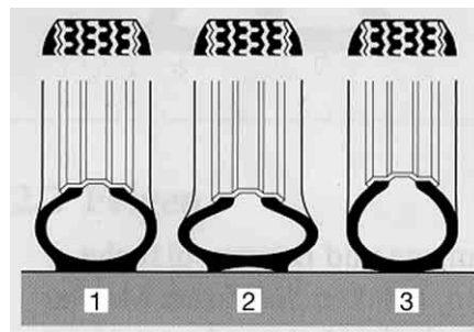
Fig. 281 Base di appoggio dei pneumatici
