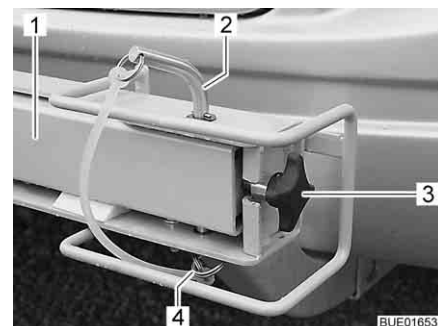
Fig. 2 Verrouillage porte-vélos
