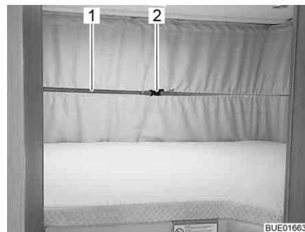
Fig. 88 Lit escamotable avec bande de serrage fermée
