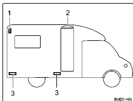
Fig. 177 Eclairage latéral
