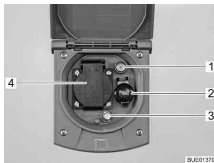
Fig. 120 Prise extérieure
