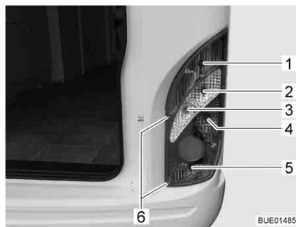
Fig. 176 Eclairage arrière
