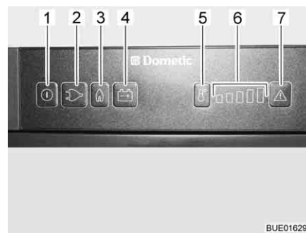
Fig. 144 Boutons de commande pour le réfrigérateur (Dometic Série 8 avec SMSE)
