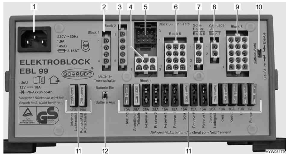
Fig. 105 Bloc électrique (EBL 99)
