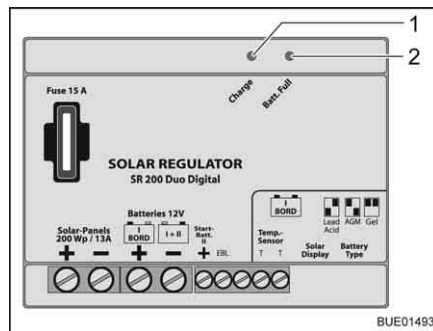
Fig. 177 Régulateur de panneau solaire 200 W
