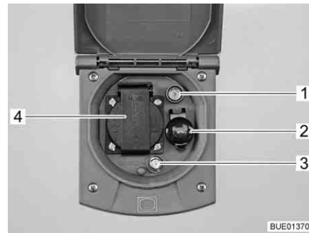
Fig. 190 Prise extérieure
