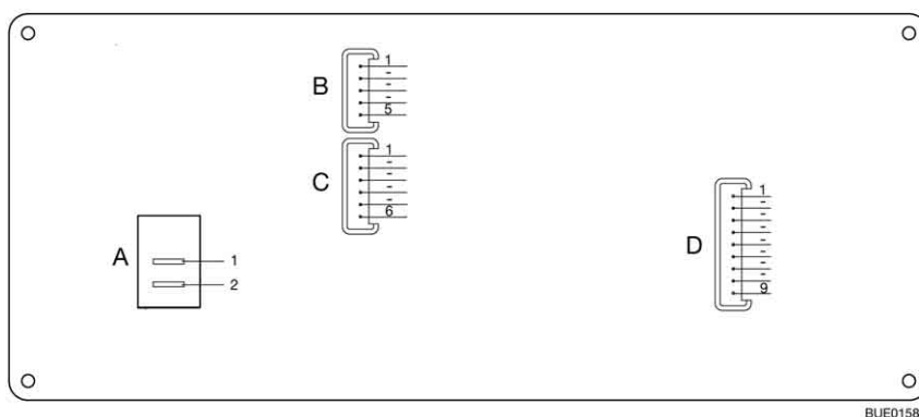
Fig. 194 Schéma de connexions, panneau de contrôle (IT 96-2)
