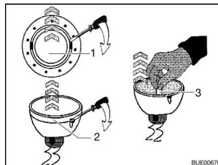
Fig. 295 Remplacer l'ampoule halogène
