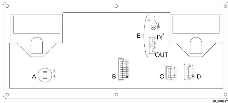
Fig. 195 Schéma fonctionnel panneau de contrôle (IT 994)
