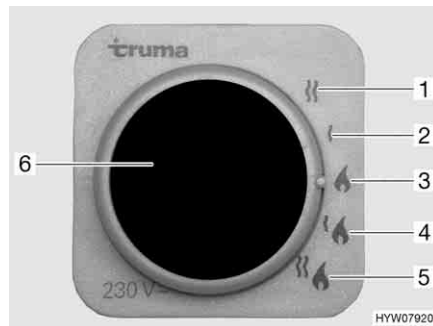
Fig. 220 Sélecteur de source d'énergie pour chauffage/chauffe-eau
