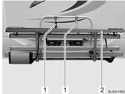
Fig. 6 Porte-vélos e-bike
