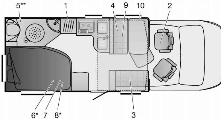
Afb. 319 Plattegrond IT 664 Ixeo
