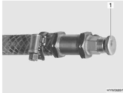
Afb. 290 Ontluchtingsventiel warmwaterverwarming
