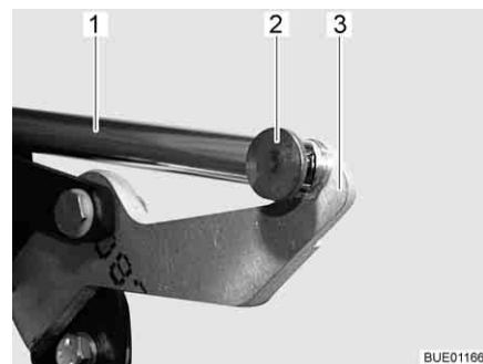
Afb. 117 Aandrijving
