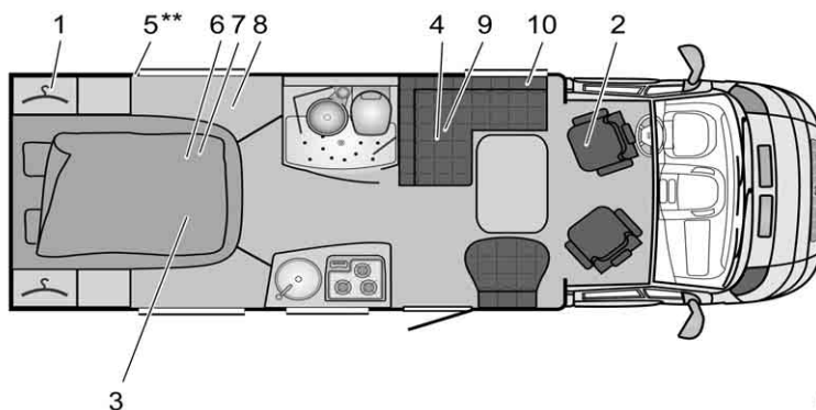
Afb. 321 Plattegrond T 687 Nexxo
