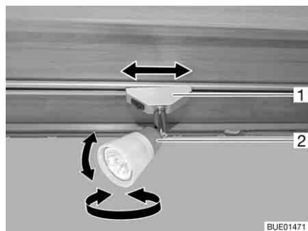
Afb. 62 Spotlight
