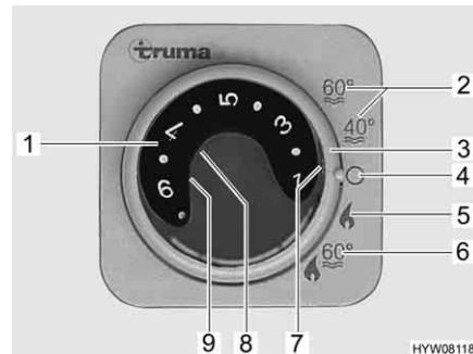
Afb. 199 Bedieningspaneel voor verwarming/boiler
