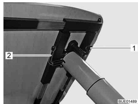
Afb. 104 Verstelling heftafel (alternatief)
