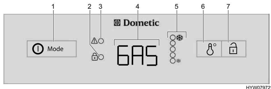
Afb. 235 Bedieningselementen voor de koelkast (Dometic 8-serie met AES)
