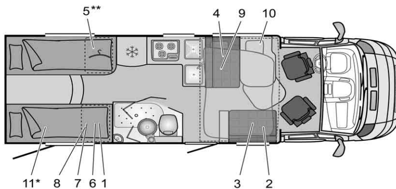
Afb. 329 Plattegrond IT 726 Ixeo/Ixeo Plus
