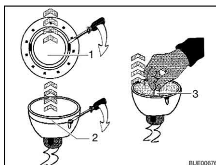
Afb. 295 De halogeengloeilamp verwisselen
