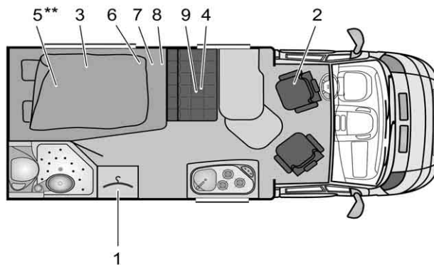
Afb. 311 Plattegrond T 569 Nexxo
