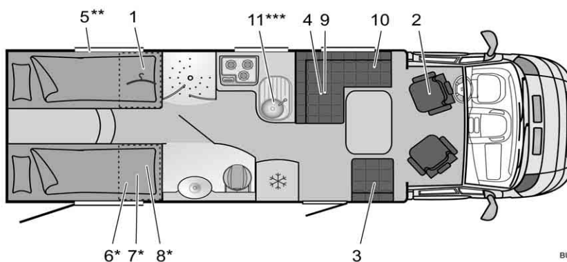
Afb. 330 Plattegrond T 728 Nexxo
