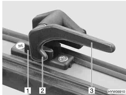
Afb. 91 Vergrendelingshendel in stand "gesloten"
