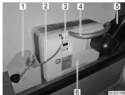
Afb. 173 Brandstofcel met tankpatroon
