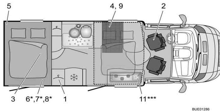
Afb. 320 Plattegrond IT 670 Ixeo Time
