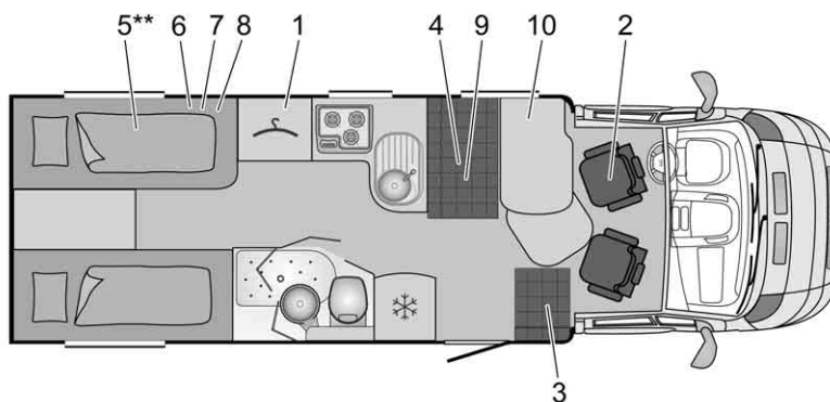
Afb. 331 Plattegrond T 729 Nexxo
