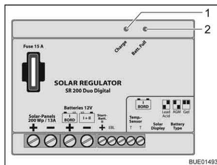
Afb. 177 Zonneregelaar 200 W
