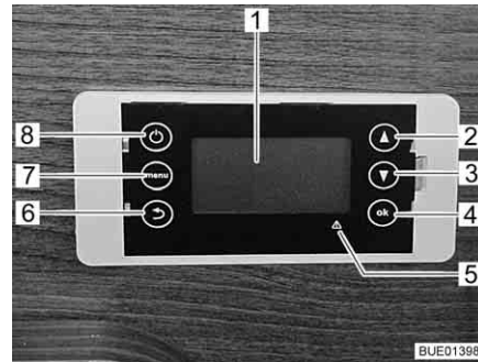
Afb. 175 Bedieningspaneel brandstofcel
