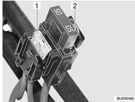
Afb. 181 Zekeringen aan de startaccu
