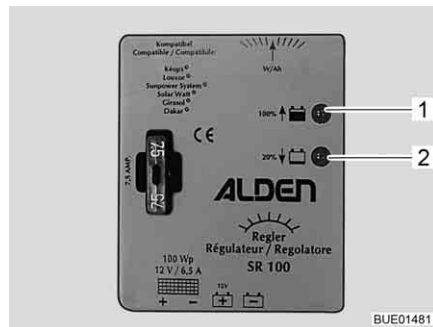
Afb. 176 Zonneregelaar 100 W
