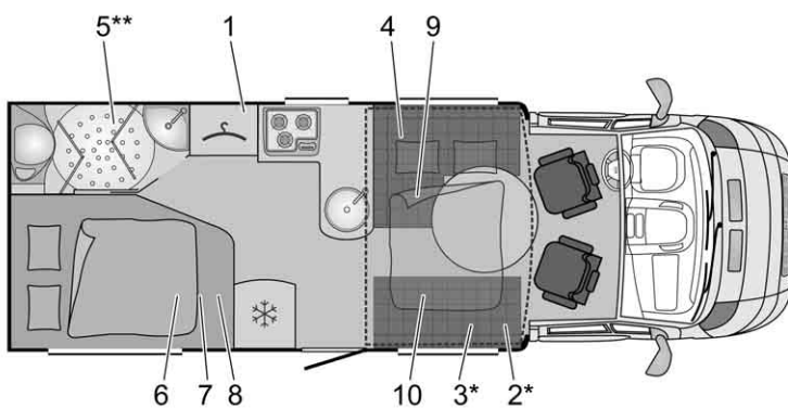
Afb. 324 Plattegrond IT 700 Ixeo Plus
