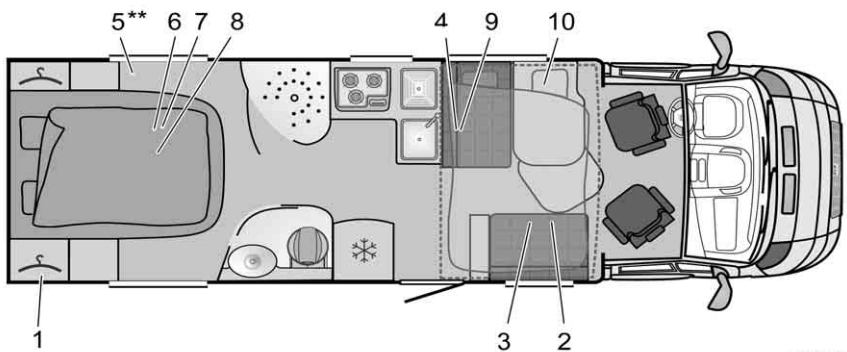
Afb. 328 Plattegrond IT 724 Ixeo Plus
