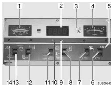
Afb. 172 Paneel IT 994
