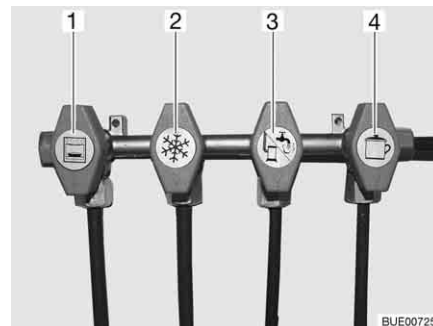
Afb. 197 Symbolen van de gasafsluitkranen
