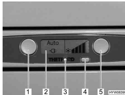
Afb. 236 Bedieningselementen voor de koelkast (Thetford met SES)
