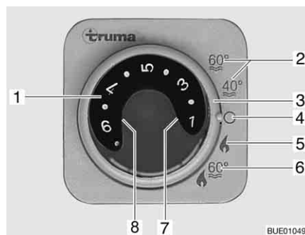
Afb. 201 Bedieningspaneel voor verwarming/boiler
