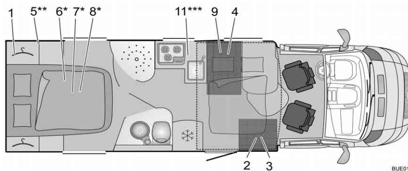
Afb. 332 Plattegrond IT 734 Ixeo Time
