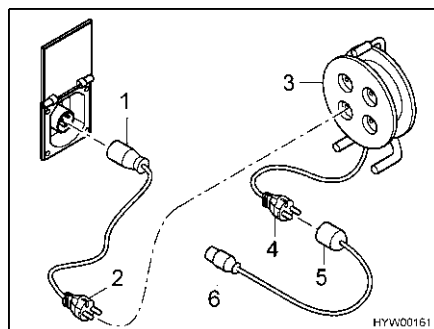
Fig. 113 Possibilità di collegamento per il collegamento a 230 V
