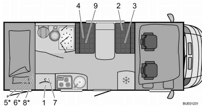
Fig. 213 Pianta A 535-2
