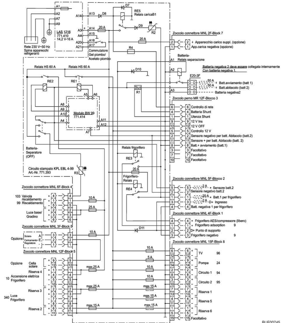
Fig. 125 Schema elettrico interno (EBL 99)
