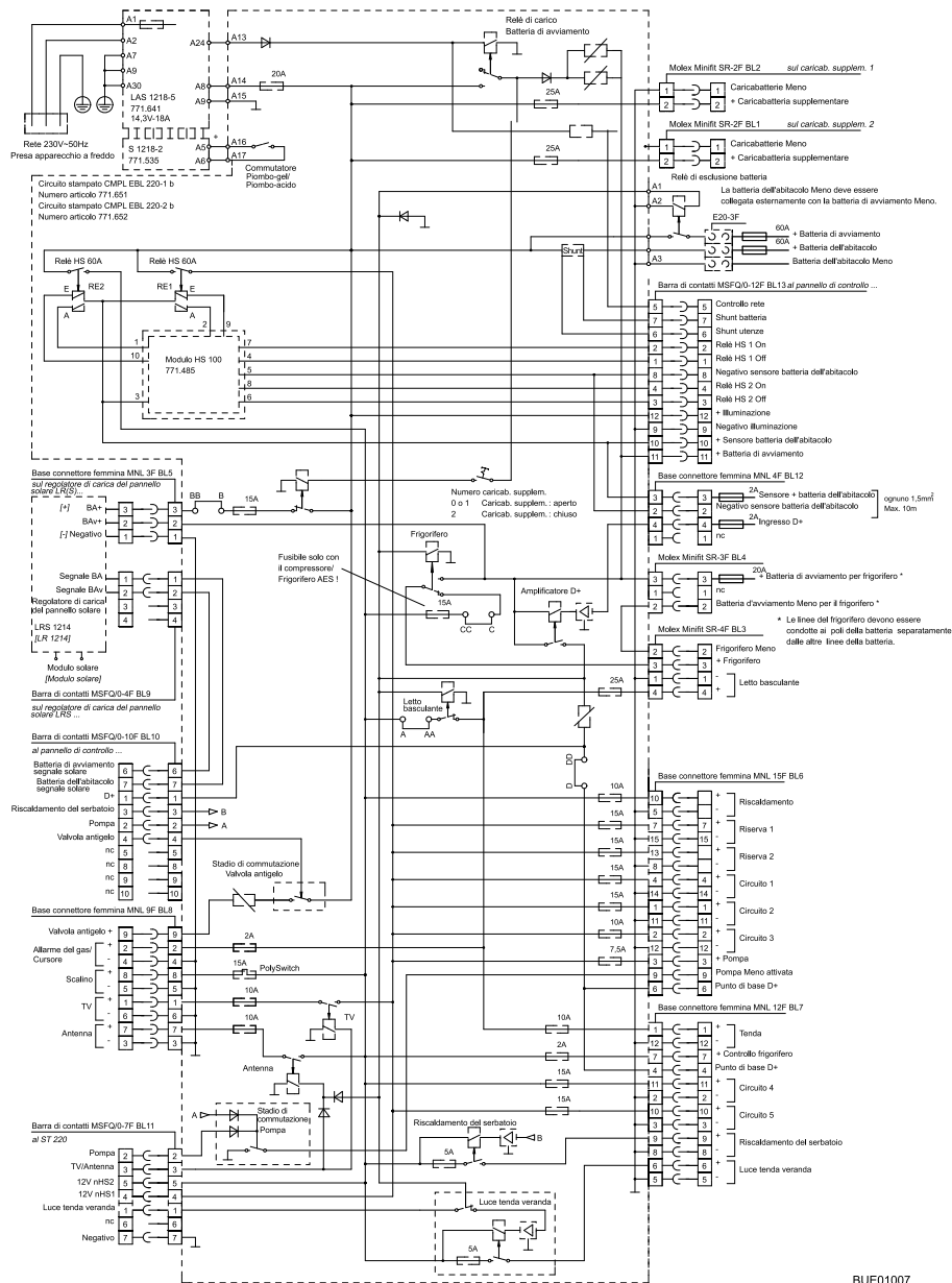
Fig. 126 Schema elettrico interno (EBL 220)
