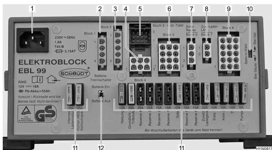
Fig. 105 Centralina elettrica (EBL 99)
