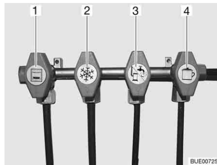
Fig. 98 Simboli dei rubinetti di arresto del gas
