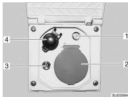
Fig. 122 Presa esterna
