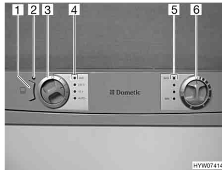
Fig. 159 Elementi di comando per il frigorifero (serie Dometic 7 con AES e RT)
