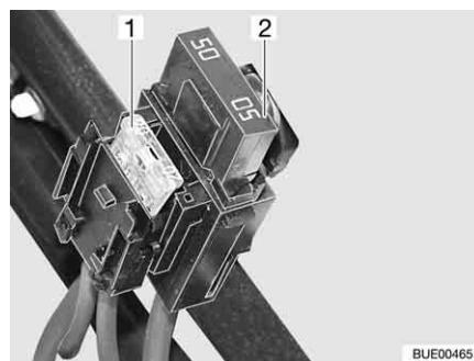
Fig. 116 Fusibili nella batteria di avviamento
