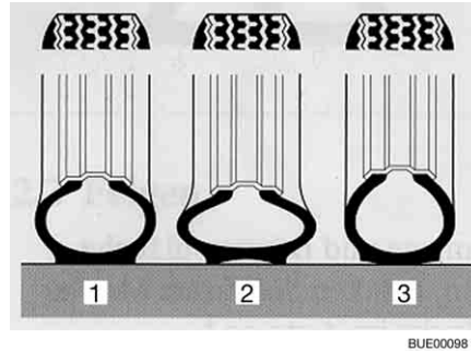
Fig. 212 Base di appoggio dei pneumatici
