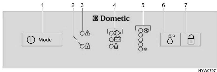
Fig. 160 Elementi di comando per il frigorifero (serie Dometic 8 con SMSE)
