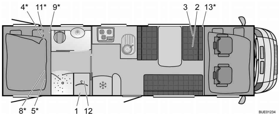
Fig. 217 Pianta A 747-2
