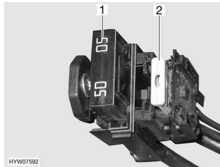
Fig. 117 Fusibili nella batteria dell'abitacolo
