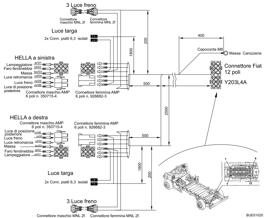
Fig. 129 Schema elettrico esterno
