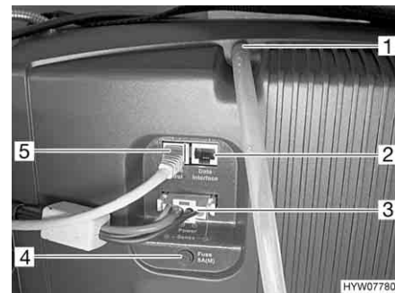
Fig. 110 Campo di collegamento pila a combustibile
