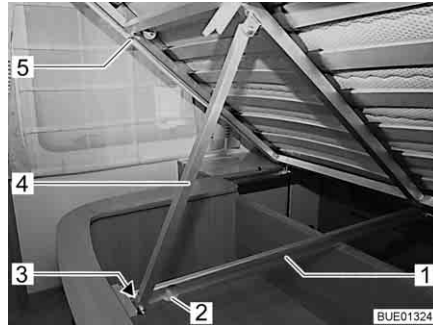
Afb. 110 Vast bed
