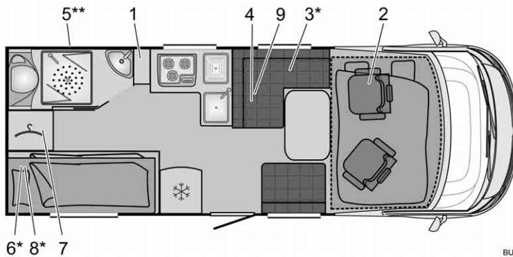
Afb. 282 Plattegrond | 676 Visio
