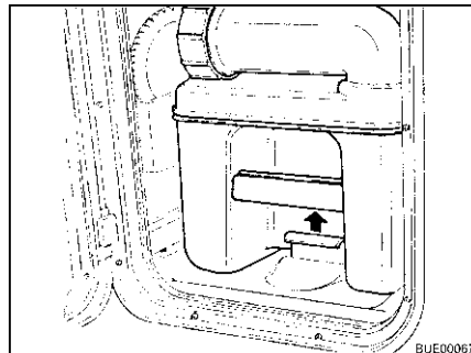
Afb. 214 Bevestigingsbeugel trekken
