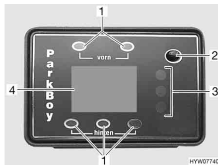
Afb. 10 Bedieningspaneel parkeerstandscontrole
