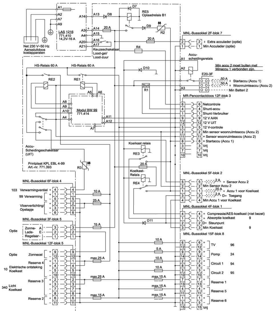
Afb. 156 Stroomschema binnen (EBL 99)
