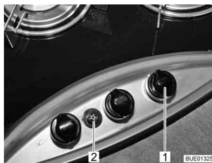
Afb. 185 Bedieningselementen voor gaskooktoestel
