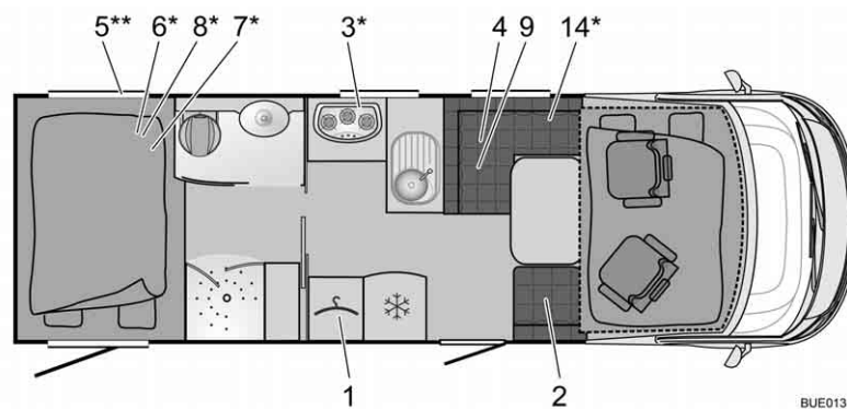
Afb. 293 Plattegrond | 729 Elegance
