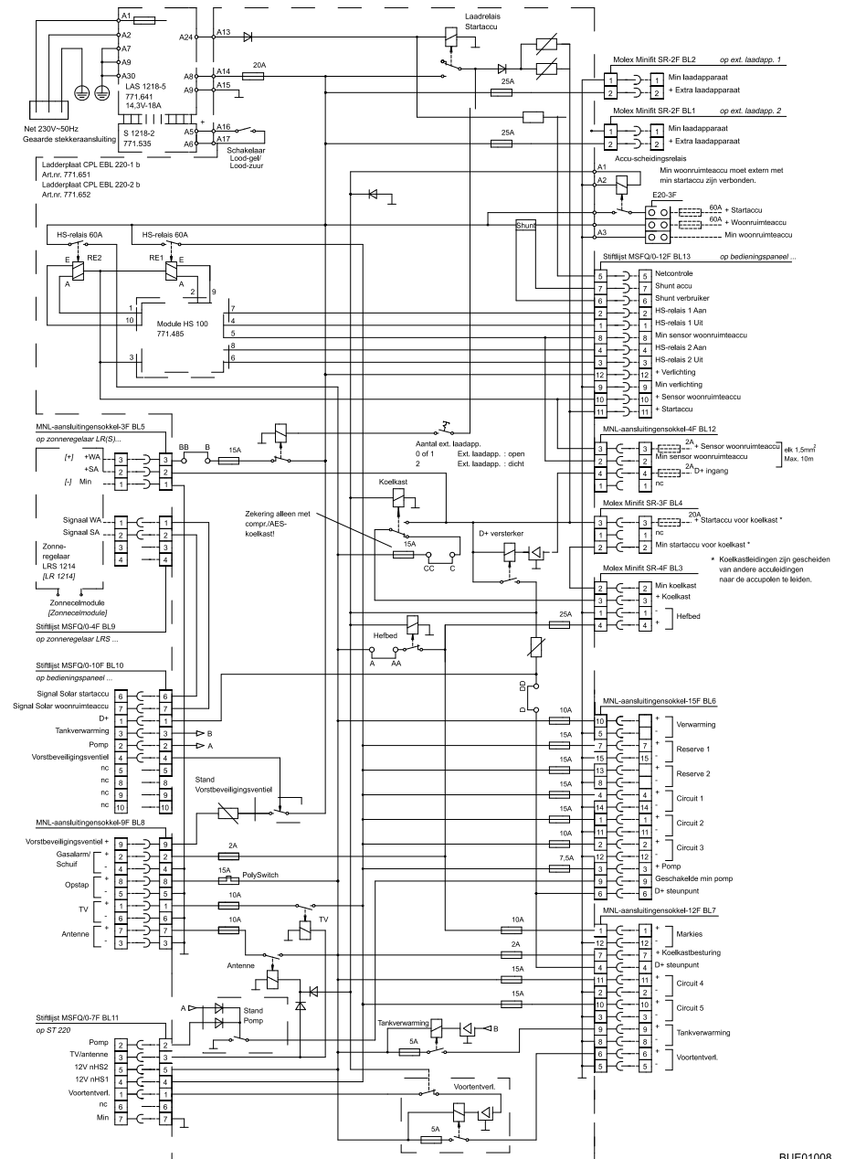
Afb. 157 Stroomschema binnen (EBL 220)
