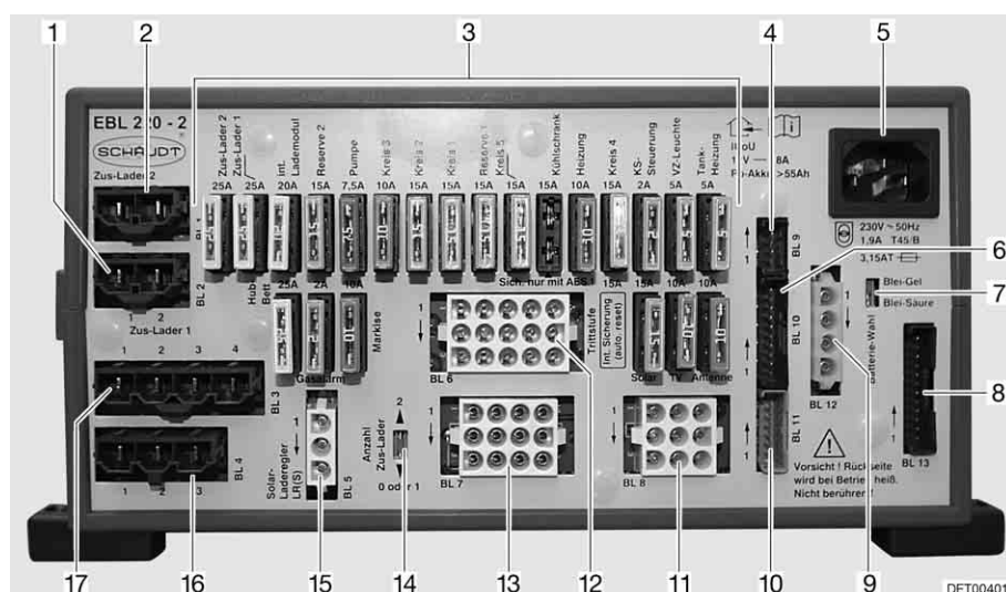
Afb. 134 Elektroblok (EBL 220)
