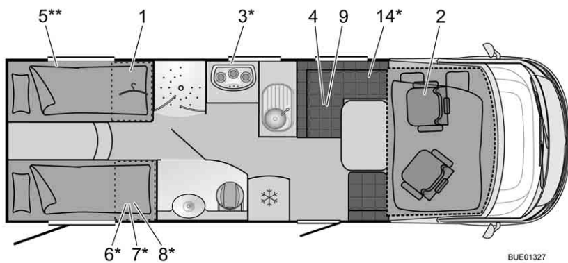
Afb. 290 Plattegrond | 726 Elegance
