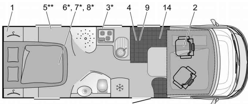
Afb. 291 Plattegrond | 727 Aviano
