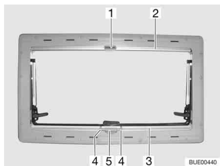
Afb. 82 Uitzetbaar raam
