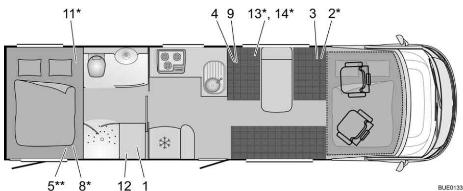
Afb. 299 Plattegrond | 822 Elegance
