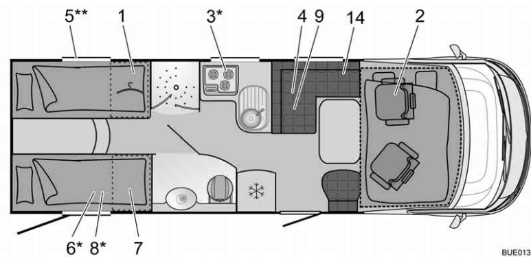
Afb. 292 Plattegrond | 728 Aviano
