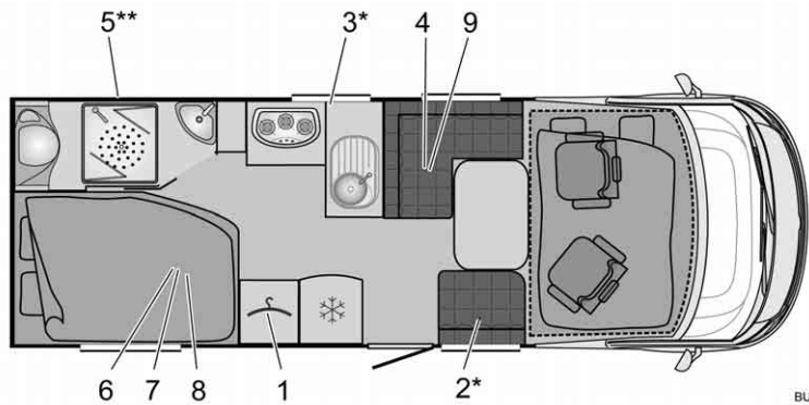
Afb. 287 Plattegrond | 705 Elegance
