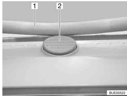
Afb. 86 Vergrendelingsknop aan het Heki-dakluik
