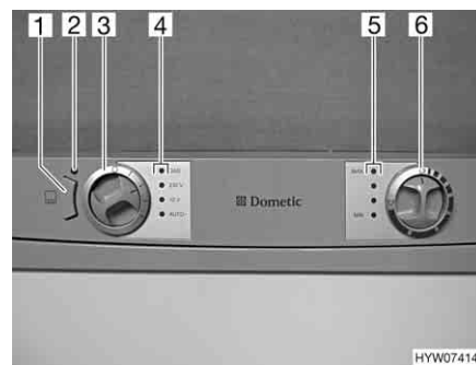
Afb. 193 Bedieningselementen voor de koelkast (Dometic 7-serie met AES en FV)
