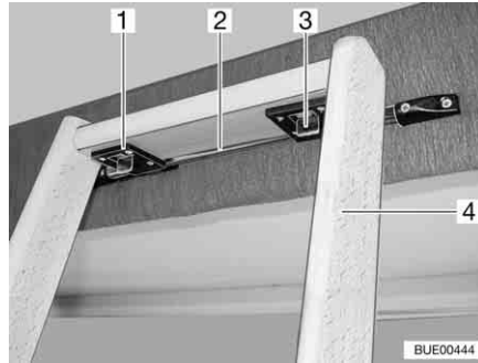
Afb. 101 Bedladder, vergrendeling
