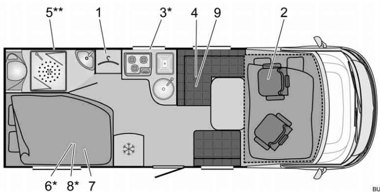
Afb. 283 Plattegrond | 684 Aviano
