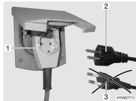
Afb. 143 Aansluiting aan een hoekkoppeling met contactdoos
