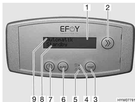
Afb. 140 Bedieningspaneel brandstofcel
