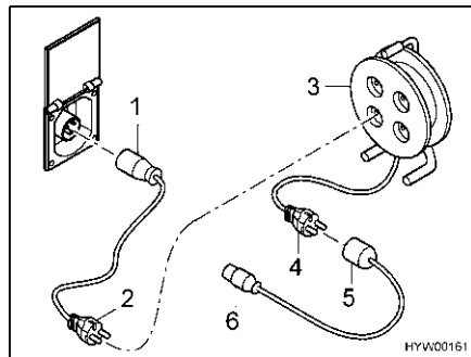
Afb. 142 Aansluitmogelijkheden 230-V-aansluiting
