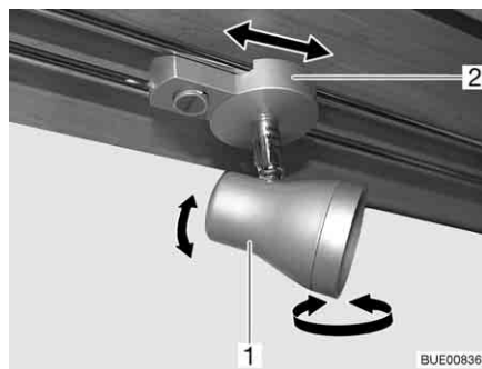
Afb. 49 Spotlight
