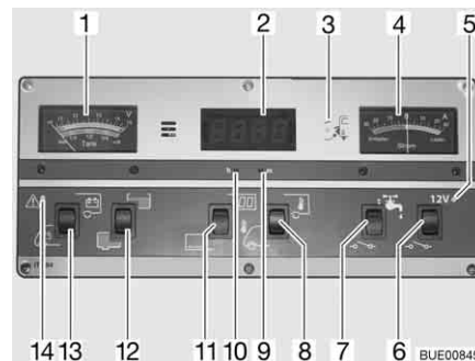
Afb. 152 Paneel IT 994
