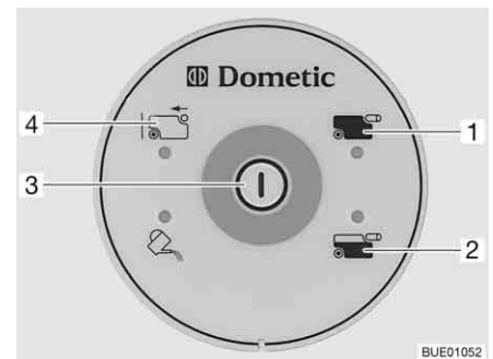
Afb. 263 Controle- en bedieningspaneel toilet
