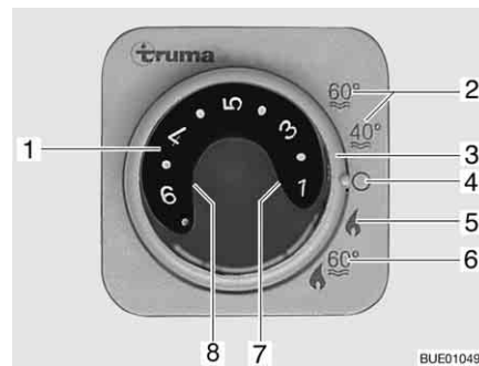
Afb. 179 Bedieningspaneel voor verwarming/boiler
