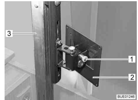
Afb. 55 Hefmechanisme
