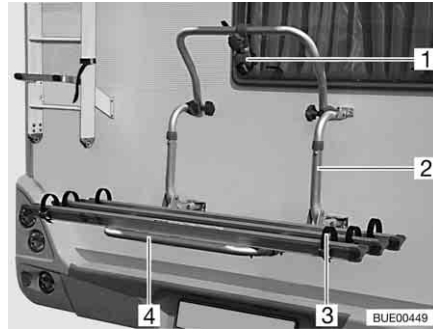
Afb. 3 Fietsenrek, niet neerlaatbaar
