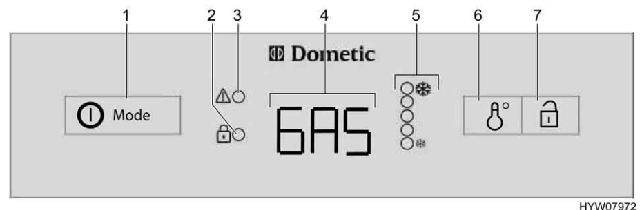
Afb. 210 Bedieningselementen voor de koelkast (Dometic 8-serie met AES)
