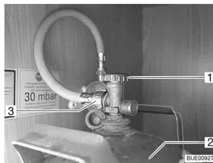
Afb. 142 Gaskast
