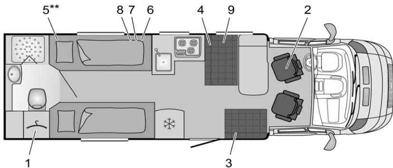
Afb. 302 Plattegrond T 720 Nexxo
