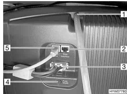
Afb. 154 Aansluitveld brandstofcel
