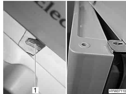
Afb. 212 Koelkastdeur in ventilatiestand (Dometic 7-serie)
