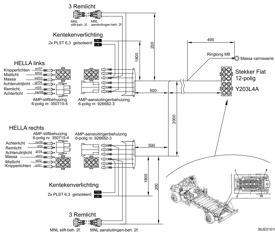
Afb. 174 Stroomschema buiten
