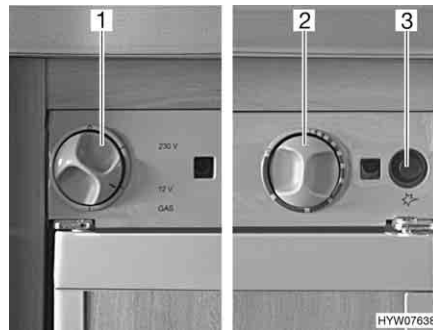
Afb. 206 Bedieningselementen voor de koelkast (Dometic 7-serie)
