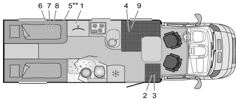
Afb. 309 Plattegrond T 729 Solano
