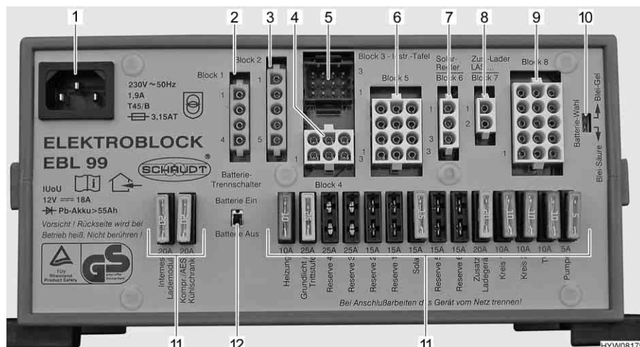
Afb. 150 Elektroblok (EBL 99)
