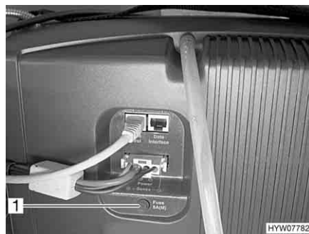
Afb. 165 Zekering van de brandstofcel
