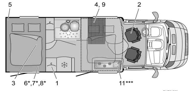
Afb. 298 Plattegrond IT 670 Ixeo Time
