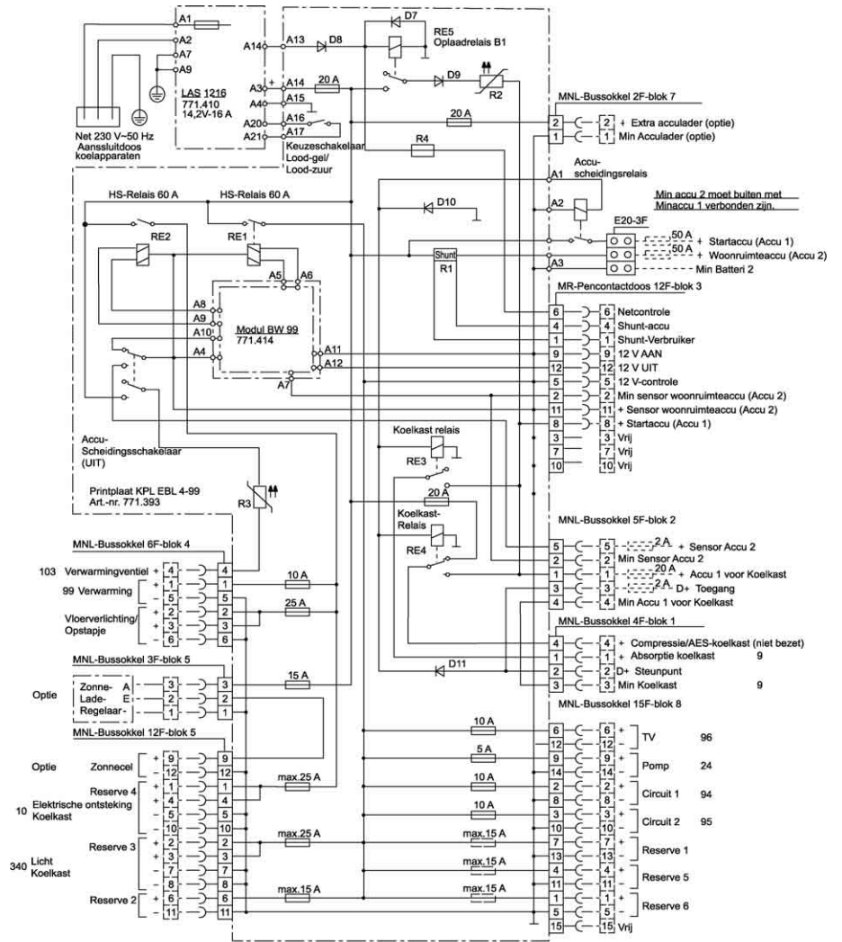
Afb. 171 Stroomschema binnen (EBL 99)
