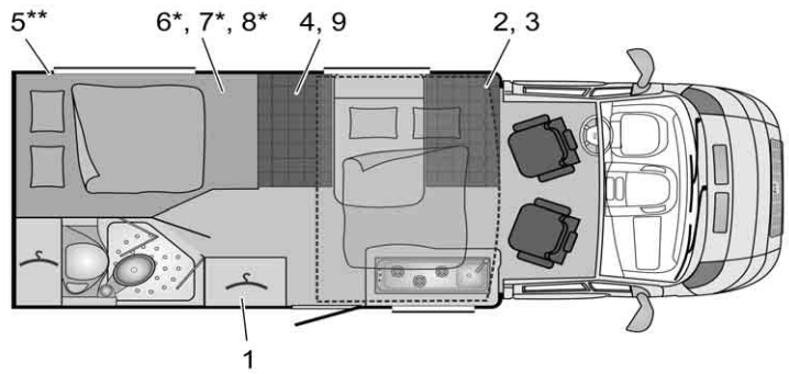
Afb. 294 Plattegrond IT 650 Ixeo Time
