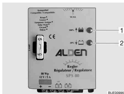
Afb. 156 Zonneregelaar
