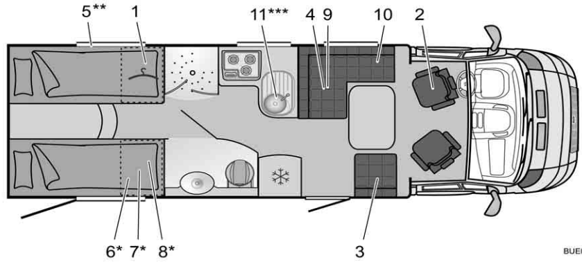
Afb. 308 Plattegrond T 728 Nexxo
