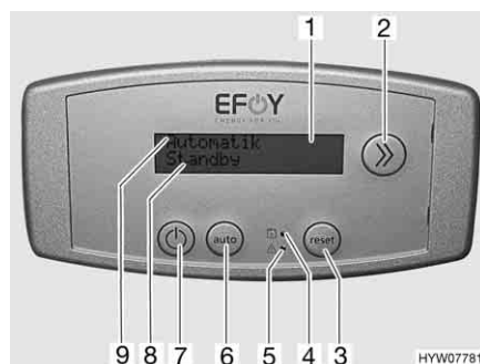
Afb. 155 Bedieningspaneel brandstofcel
