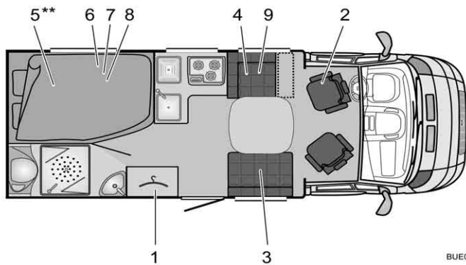
Afb. 288 Plattegrond T 580 Nexxo
