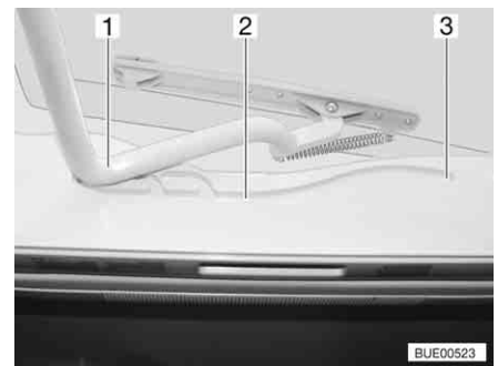
Afb. 68 Heki-dakluik, geleiding
