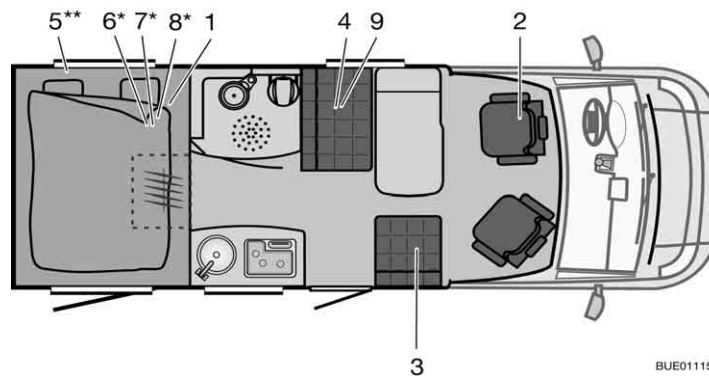
Afb. 287 Plattegrond T 571 Travel Van
