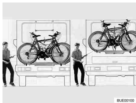
Afb. 2 Fietsenrek, neerlaatbaar
