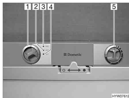
Afb. 207 Bedieningselementen voor de koelkast (Dometic 7-serie)
