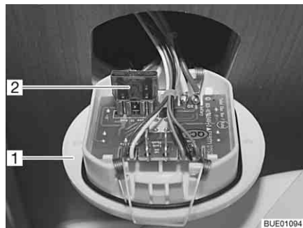
Afb. 164 Zekering van het toilet
