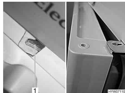
Afb. 214 Koelkastdeur/vriesvakdeur in ventilatiestand (Dometic 7-serie met apart vriesvak)
