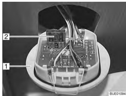
Fig. 120 Fusible des toilettes
