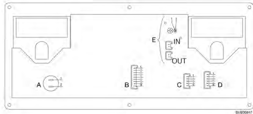
Fig. 130 Schéma fonctionnel panneau de contrôle (IT 994)
