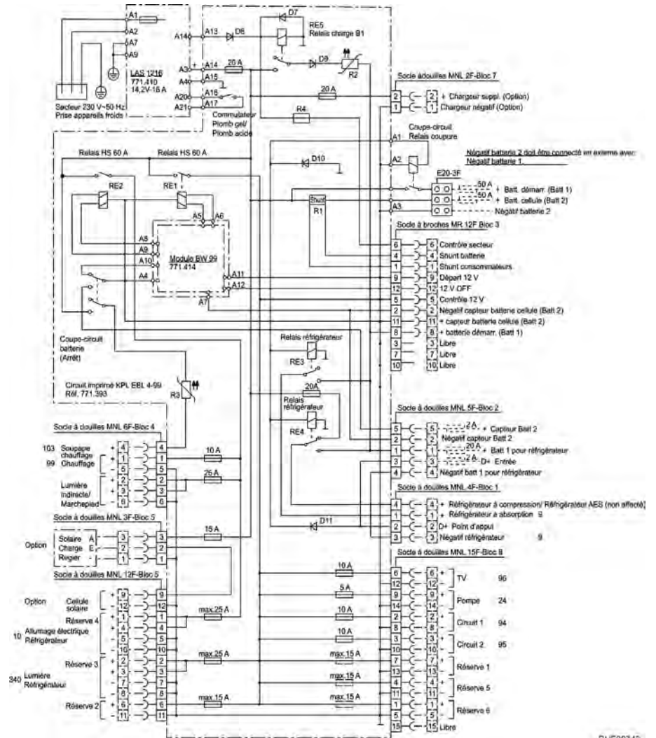
Fig. 127 Schéma électrique intérieur (EBL 99)
