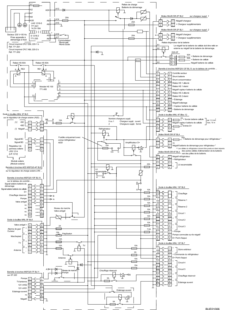
Fig. 128 Schéma électrique intérieur (EBL 220)
