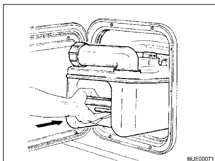
Fig. 200 Insérer la cassette Thetford
