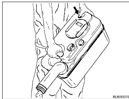
Fig. 220 Vidanger le réservoir pour matières fécales
