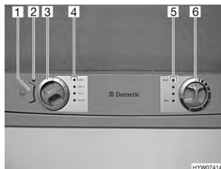
Fig. 165 Boutons de commande pour le réfrigérateur (Dometic Série 7 avec AES et CC)
