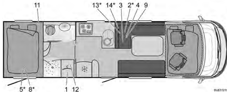
Fig. 268 Tracé I 821 Elegance
