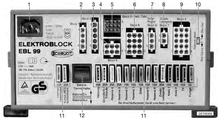
Fig. 107 Bloc électrique (EBL 99)
