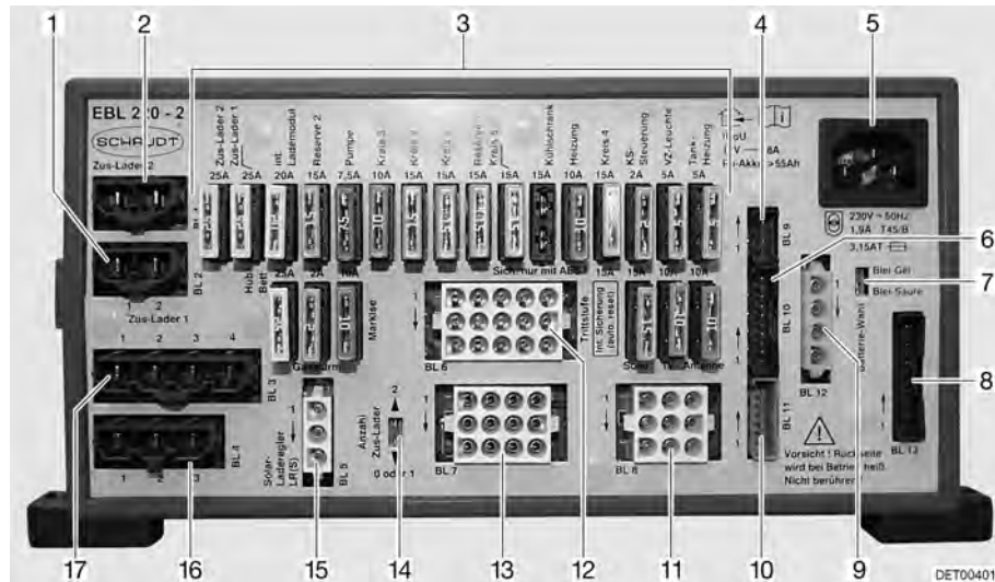
Fig. 108 Bloc électrique (EBL 220)
