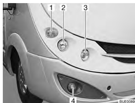
Fig. 225 Eclairage avant
