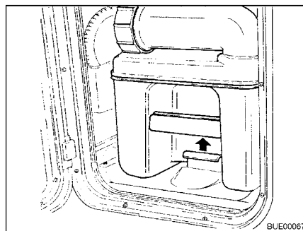
Fig. 185 Tirer l'étrier de fixation
