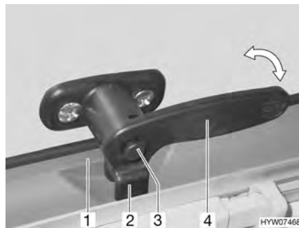
Fig. 66 Levier de verrouillage avec bouton de sécurité en position "Fermé"
