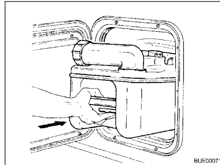
Fig. 213 Insérer la cassette Thetford
