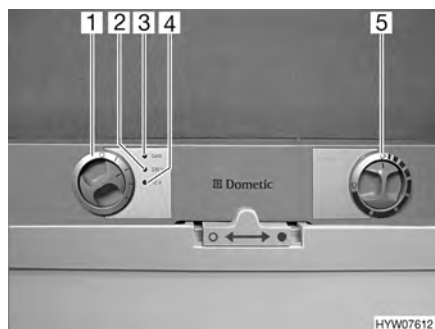
Fig. 164 Boutons de commande pour le réfrigérateur (Dometic Série 7)
