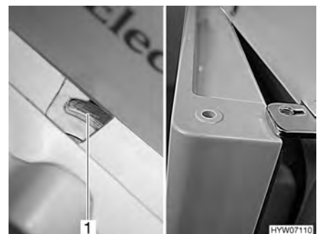
Fig. 170 Porte du réfrigérateur/du compartiment congélation en position de ventilation (Dometic Série 7 avec compartiment congélation séparé)
