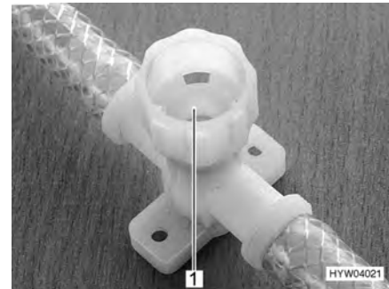
Fig. 182 Robinet de vidange (avec capuchon tournant)
