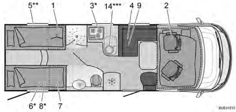
Fig. 264 Tracé I 728 Aviano
