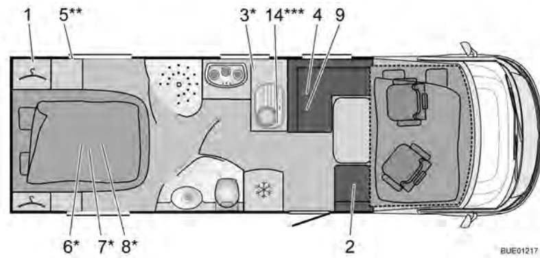
Fig. 266 Tracé I 730 Elegance
