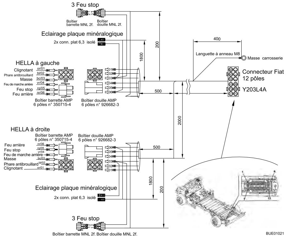
Fig. 132 Schéma électrique extérieur
