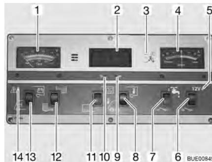
Afb. 110 Paneel IT 994
