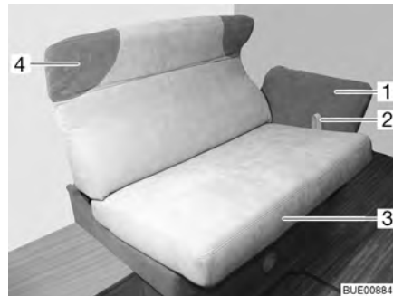
Afb. 84 Verstelling van de langszitbank
