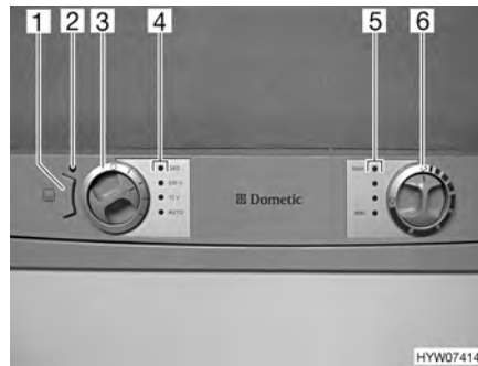
Afb. 165 Bedieningselementen voor de koelkast (Dometic 7-serie met AES en FV)
