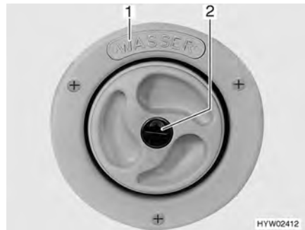
Afb. 175 Afsluitdeksel voor drinkwatervulopening
