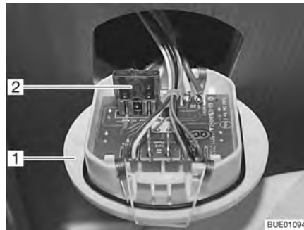
Afb. 120 Zekering van het toilet
