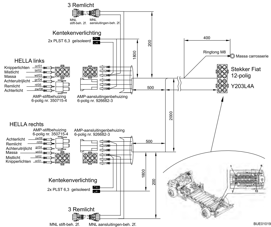
Afb. 132 Stroomschema buiten
