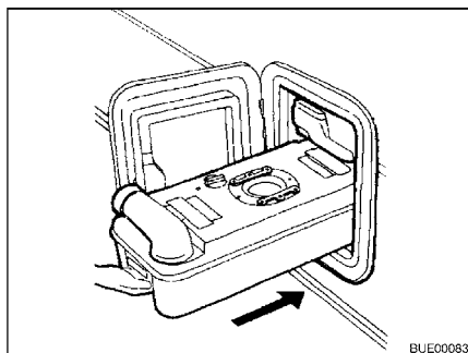
Afb. 189 Thetford-cassette inschuiven
