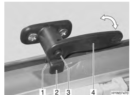
Afb. 71 Vergrendelingshendel met vergrendelingsknop in stand "continue ventilatie"
