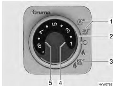
Afb. 151 Bedieningspaneel voor verwarming/boiler
