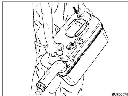
Afb. 199 Thetford-cassette leegmaken
