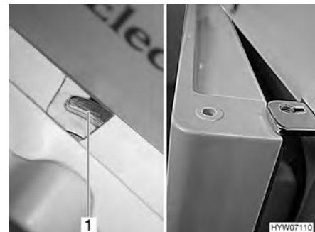
Afb. 168 Koelkastdeur in ventilatiestand (Dometic 7-serie)
