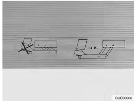
Afb. 5 Waarschuwing opstap
