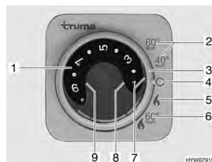
Afb. 135 Bedieningspaneel voor verwarming/boiler
