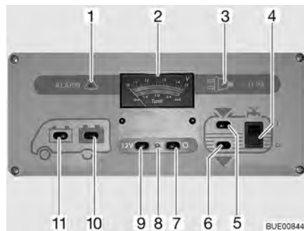
Afb. 109 Paneel IT 96-2
