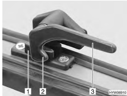
Afb. 68 Vergrendelingshendel zonder vergrendelingsknop in stand "gesloten"
