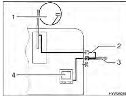
Afb. 125 TV in het voertuig
