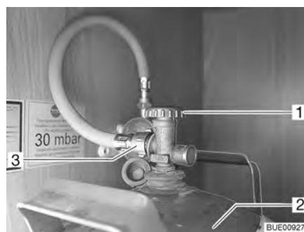
Afb. 99 Gaskast
