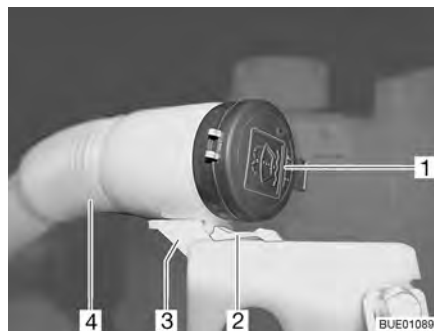
Afb. 28 Vulopening vloeistofreservoir
