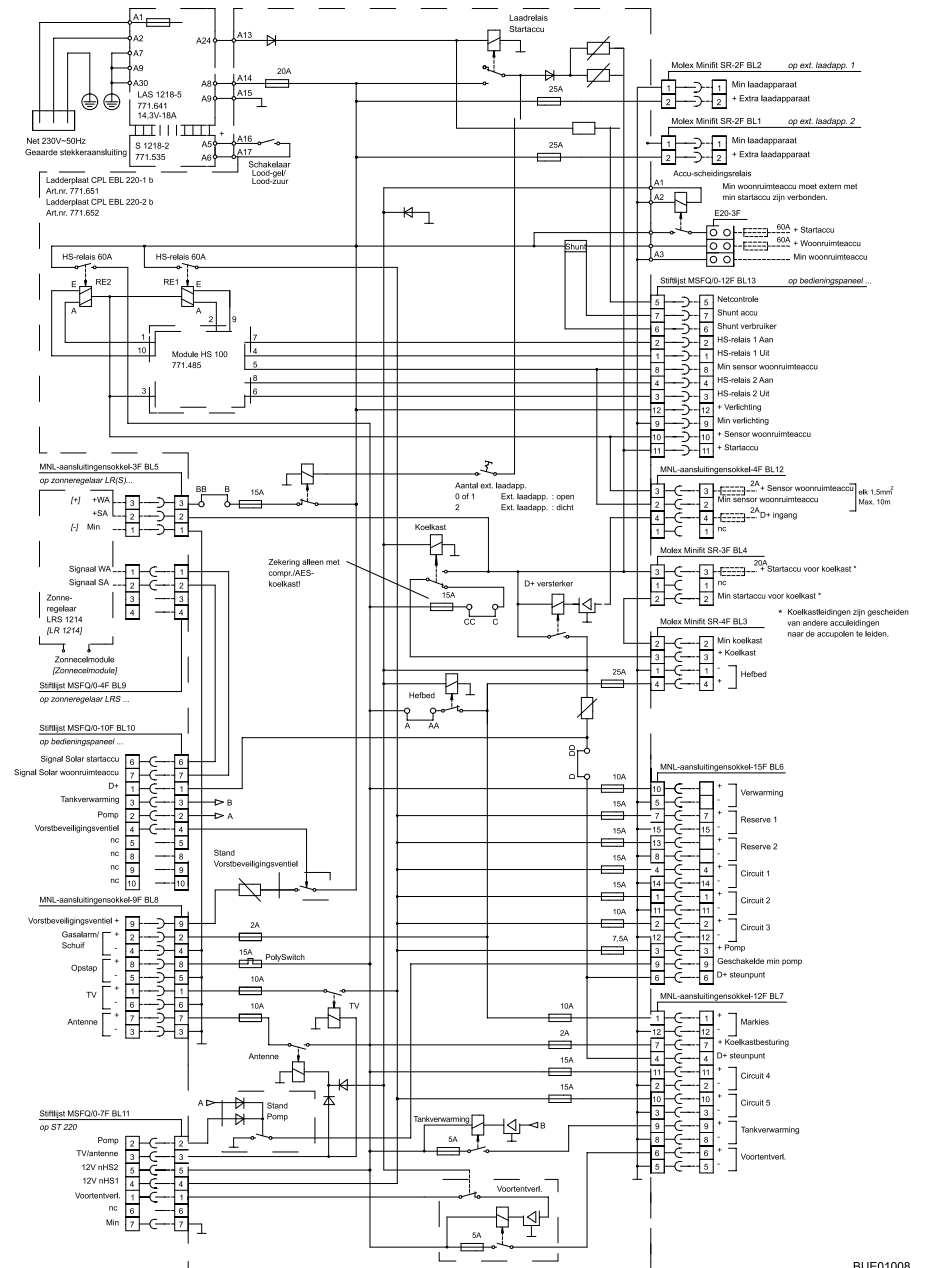
Afb. 128 Stroomschema binnen (EBL 220)
