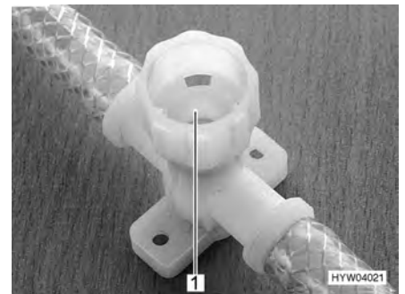
Afb. 184 Aftapkraan (met draaikap)
