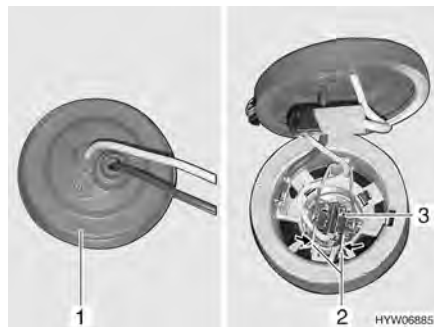
Afb. 226 Grootlicht/parkeerlicht/dimlicht
