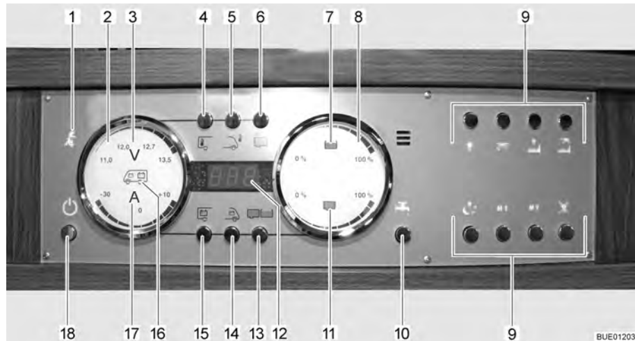
Afb. 111 Paneel LT 510
