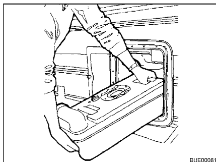
Afb. 202 Thetford-cassette uitnemen
