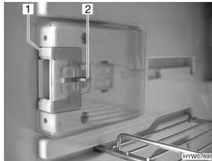
Afb. 173 Sluiting in normale stand
