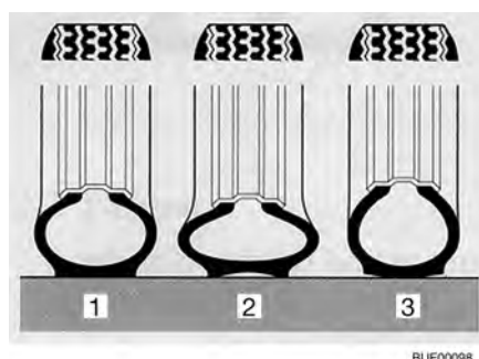
Afb. 249 Draagvlak van de band
