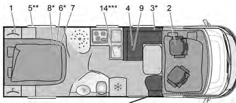
Afb. 261 Plattegrond I 726 Visco
