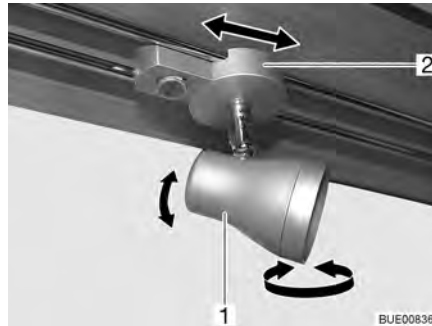
Afb. 59 Spotlight
