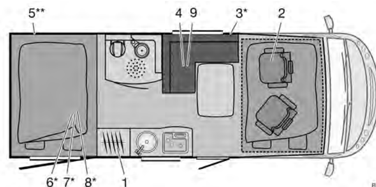
Afb. 251 Plattegrond I 620 Visero
