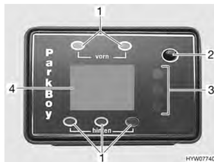
Afb. 10 Bedieningspaneel parkeerafstandscontrole
