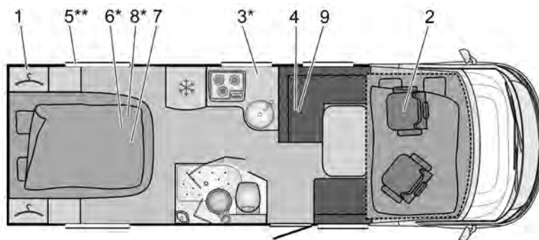
Afb. 260 Plattegrond I 725 Aviano
