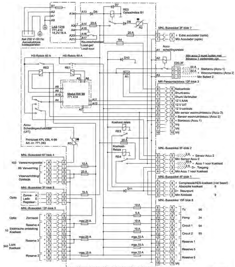
Afb. 127 Stroomschema binnen (EBL 99)
