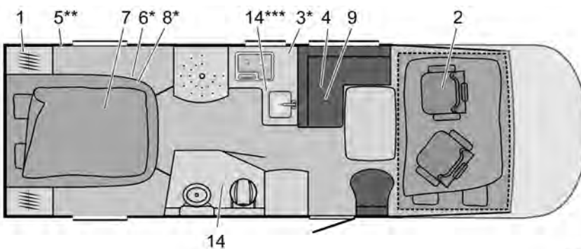
Afb. 263 Plattegrond I 727 Aviano
