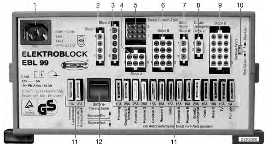
Afb. 107 Elektroblok (EBL 99)
