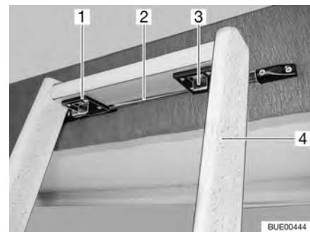
Afb. 86 Bedladder, vergrendeling
