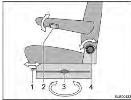
Afb. 13 Bestuurders- en passagiersstoel
