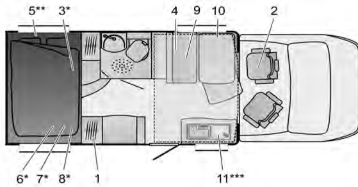
Fig. 276 Esquema IT 674 Ixeo
