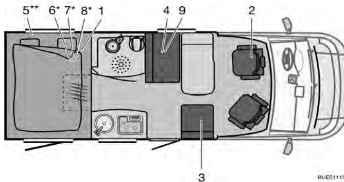
Fig. 268 Esquema T 571 Travel Van
