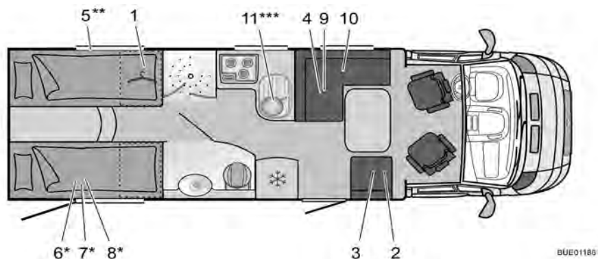
Fig. 284 Esquema T 728 Solano
