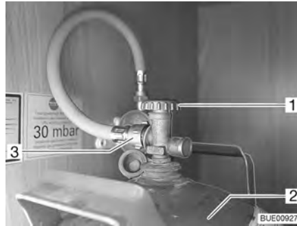
Fig. 124 Caja para bombonas de gas
