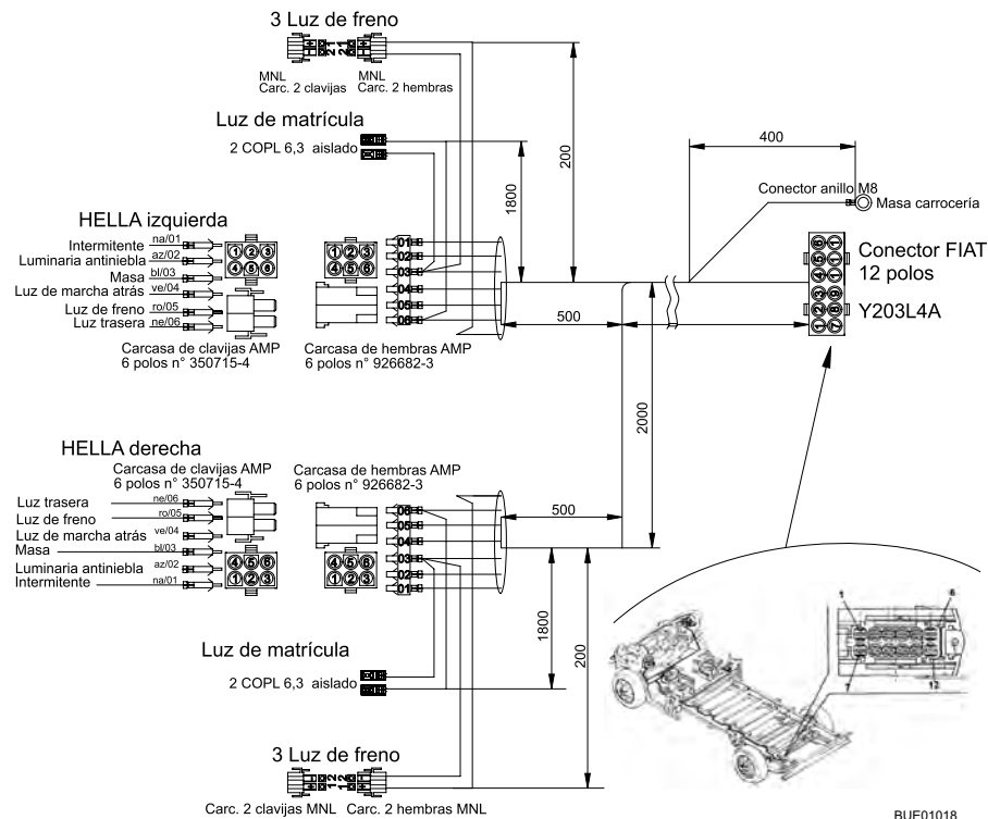
Fig. 153 Esquema de circuitos exterior
