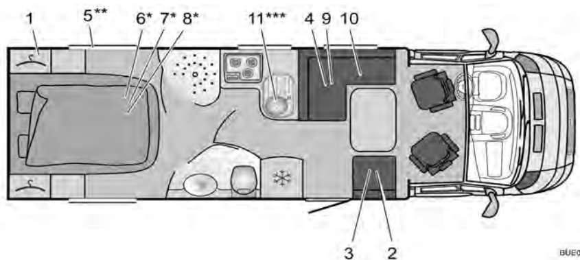
Fig. 282 Esquema T 727 Solano
