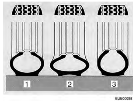
Fig. 266 Superficie de contacto del neumático
