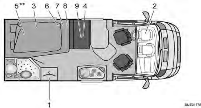
Fig. 267 Esquema T 569 Nexxo
