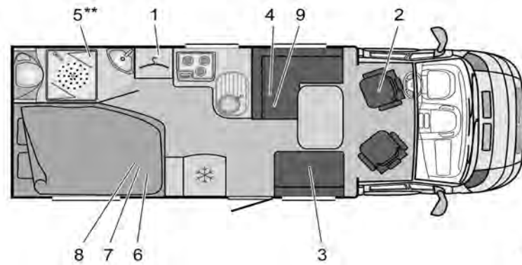
Fig. 273 Esquema T 660 Nexxo
