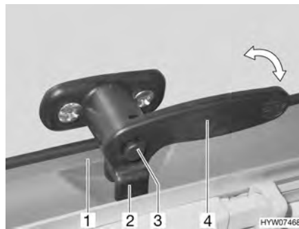
Fig. 57 La palanca de bloqueo con botón de seguridad en la posición "cerrada"
