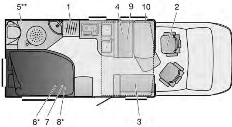
Fig. 274 Esquema IT 664 Ixeo
