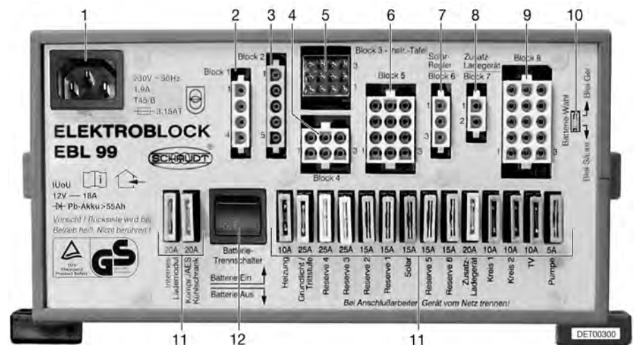
Fig. 132 Bloque eléctrico (EBL 99)
