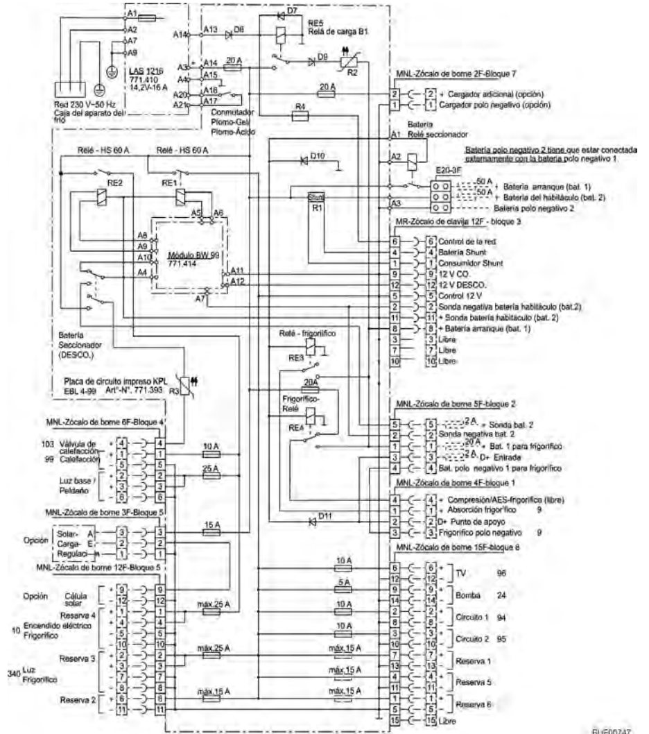
Fig. 150 Esquema de circuitos interior (EBL 99)
