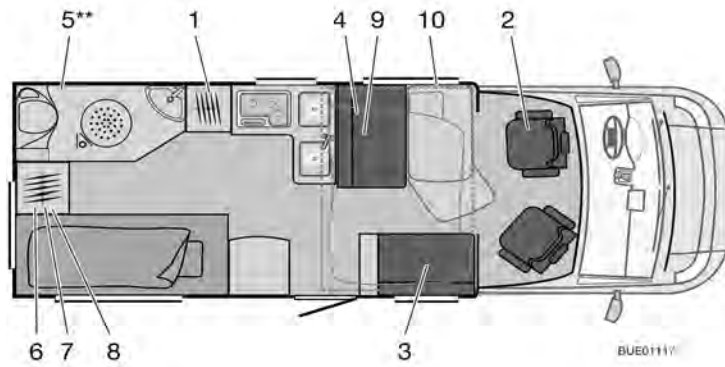
Fig. 275 Esquema IT 666 Ixeo
