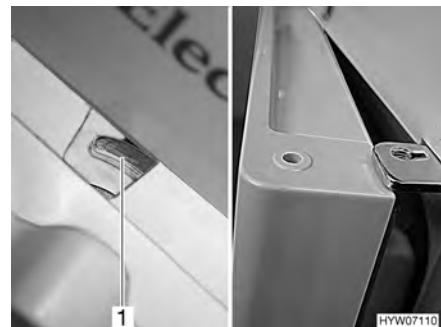
Fig. 194 Porta del frigorifero in posizione di ricircolo dell'aria (serie Dometic 7)
