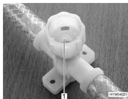
Fig. 209 Rubinetto di scarico (con tappo a vite)
