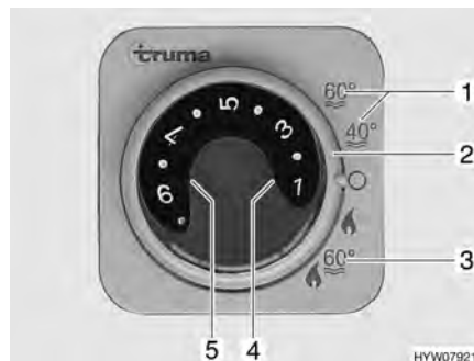
Fig. 173 Centralina di controllo per riscaldamento/boiler
