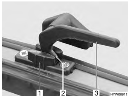
Fig. 61 Leva di serraggio senza bottone di sicurezza in posizione "Aerazione continua"
