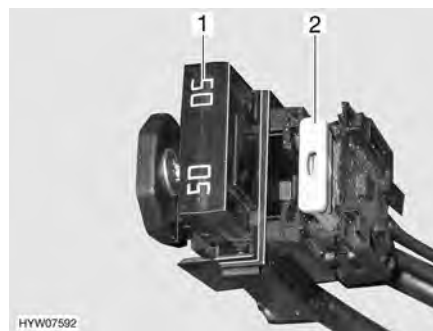
Fig. 140 Fusibili nella batteria dell'abitacolo
