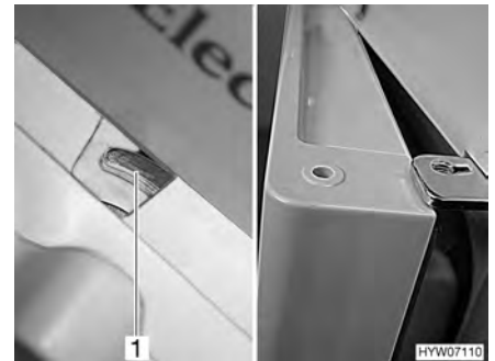
Fig. 196 Porta del frigorifero/del vano congelatore in posizione di ricircolo d'aria (serie Dometic 7 con vano congelatore separato)
