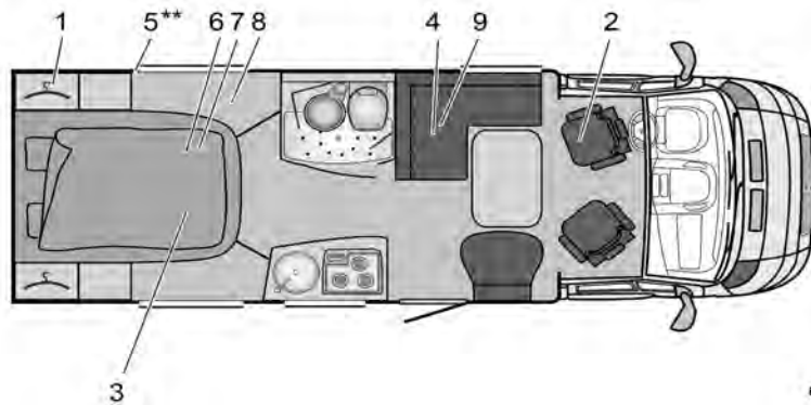
Fig. 277 Pianta T 687 Nexxo
