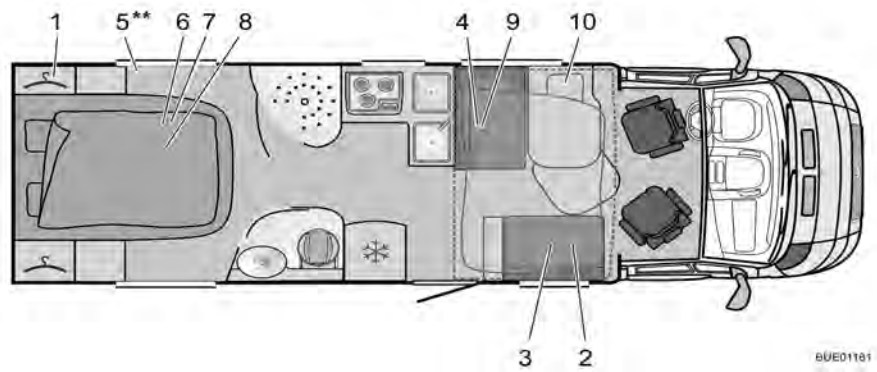
Fig. 279 Pianta IT 724 Ixeo
