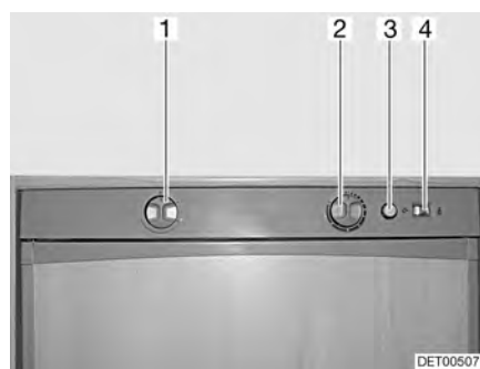
Fig. 188 Elementi di comando per il frigorifero (serie Dometic 7 con accensione manuale)
