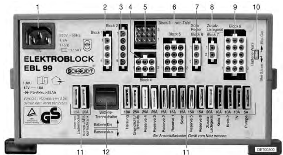
Fig. 132 Centralina elettrica (EBL 99)
