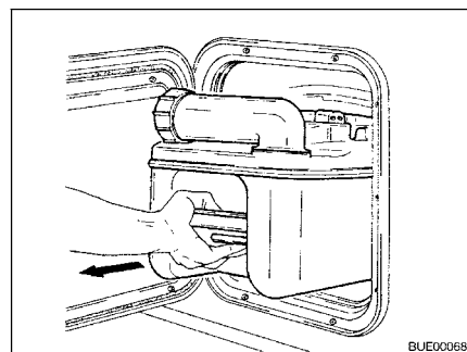
Fig. 235 Cassetta Thetford, rimozione
