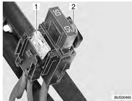
Fig. 139 Fusibili nella batteria di avviamento
