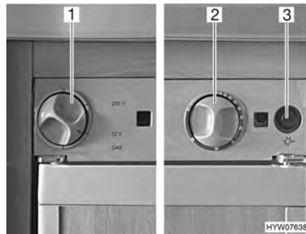
Fig. 187 Elementi di comando per il frigorifero (serie Dometic 7)
