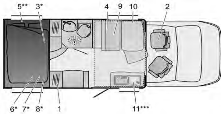
Fig. 276 Pianta IT 674 Ixeo
