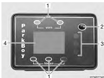
Fig. 16 Centralina di controllo del sensore di controllo distanza durante il parcheggio
