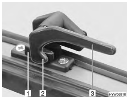
Fig. 59 Leva di serraggio senza bottone di sicurezza in posizione "Chiuso"
