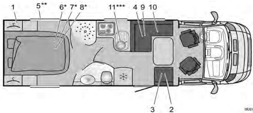
Fig. 282 Pianta T 727 Solano
