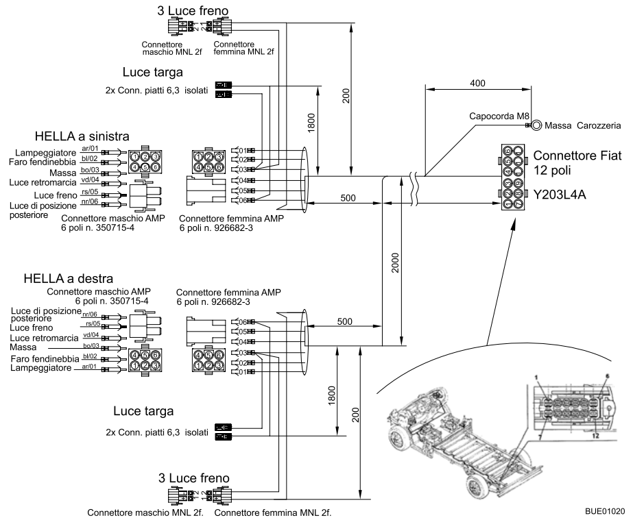
Fig. 153 Schema elettrico esterno
