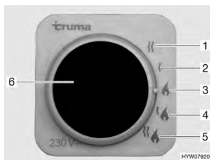
Fig. 175 Selettore di energia per riscaldamento/boiler
