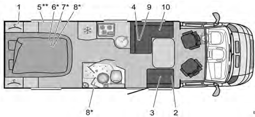
Fig. 280 Pianta T 725 Solano
