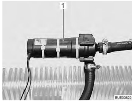
Fig. 163 Pompa di circolazione aggiuntiva
