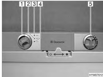
Fig. 189 Elementi di comando per il frigorifero (serie Dometic 7)
