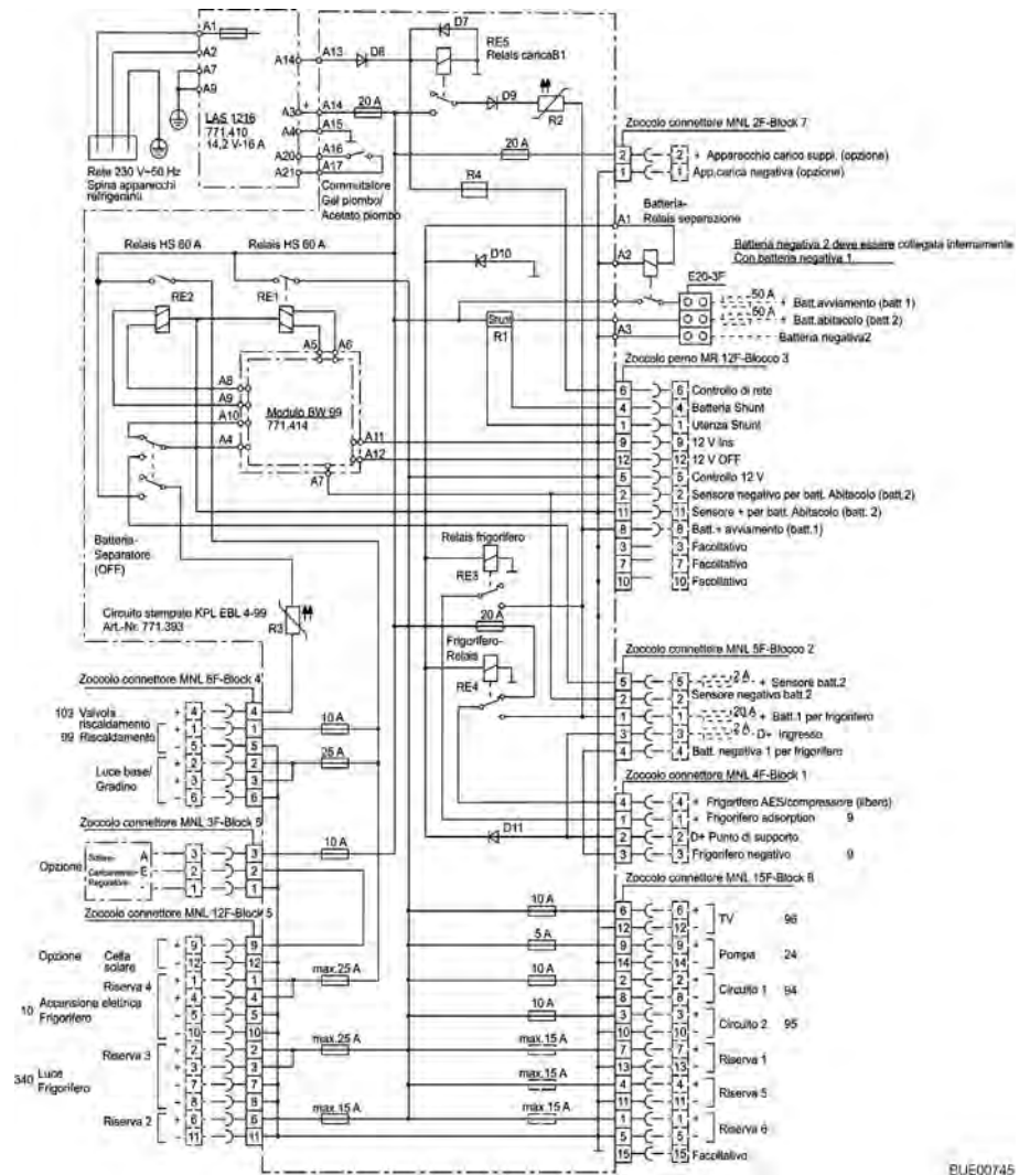
Fig. 150 Schema elettrico interno (EBL 99)
