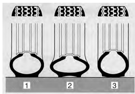
Fig. 266 Base di appoggio dei pneumatici
