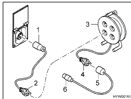
Fig. 136 Possibilità di collegamento per il collegamento a 230 V
