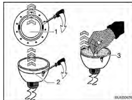
Afb. 254 De halogeengloeilamp verwisselen
