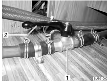
Afb. 161 3-wegventiel
