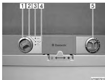
Afb. 189 Bedieningselementen voor de koelkast (Dometic 7-serie)
