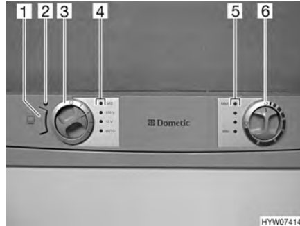
Afb. 190 Bedieningselementen voor de koelkast (Dometic 7-serie met AES en FV)
