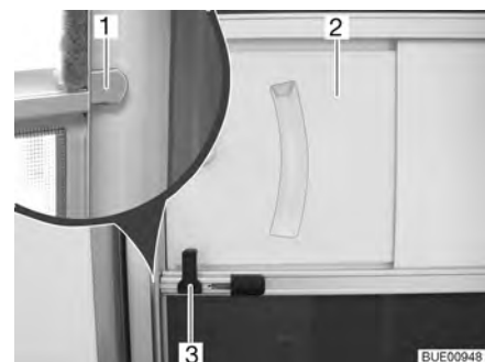
Afb. 34 Vergrendeling op frame
