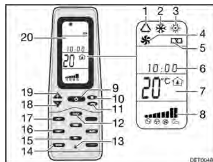
Afb. 169 Afstandsbediening
