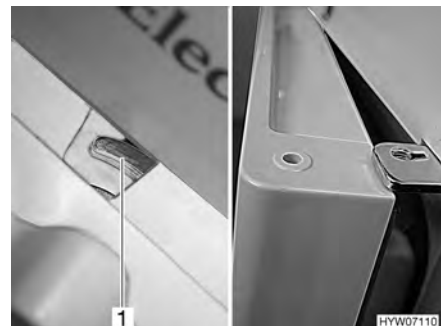
Afb. 196 Koelkastdeur/vriesvakdeur in ventilatiestand (Dometic 7-serie met apart vriesvak)
