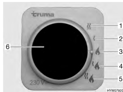
Afb. 175 Energiekeuzeschakelaar voor verwarming/boiler
