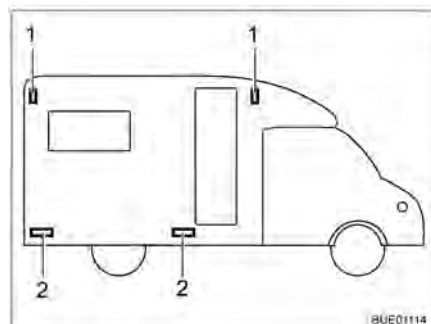
Afb. 252 Verlichting zijkant
