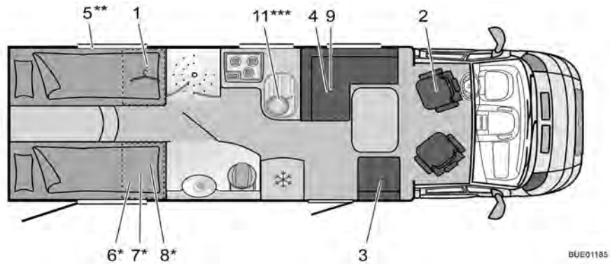
Afb. 283 Plattegrond T 728 Nexxo
