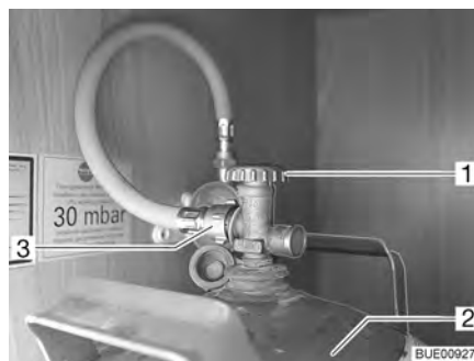
Afb. 124 Gaskast
