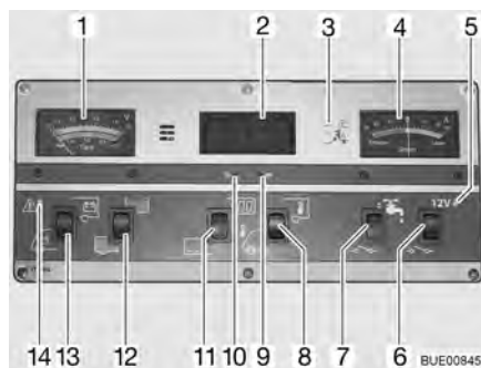
Afb. 134 Paneel IT 994
