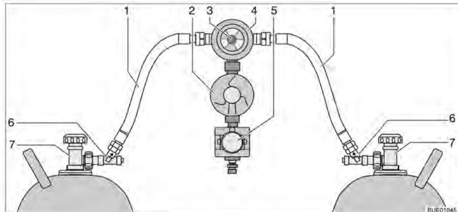
Afb. 127 Omschakelinstallatie Crash-Protection-Unit
