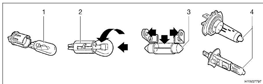
Afb. 249 Gloeilamptypen
