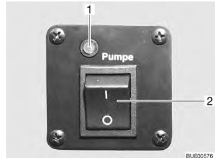
Afb. 164 Bedieningsschakelaar extra circulatiepomp
