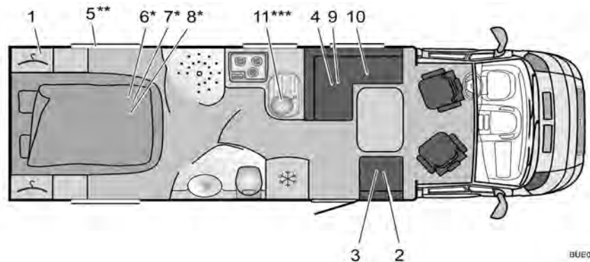
Afb. 282 Plattegrond T 727 Solano
