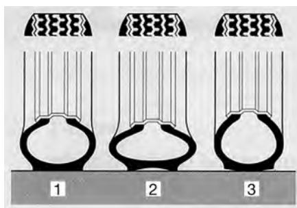
Afb. 266 Draagvlak van de band
