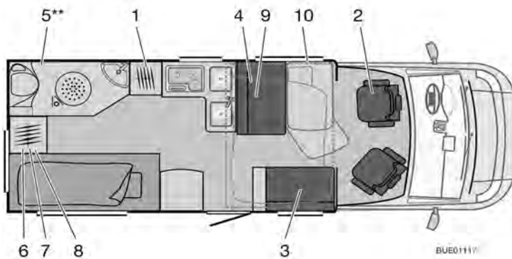
Afb. 275 Plattegrond IT 666 Ixeo
