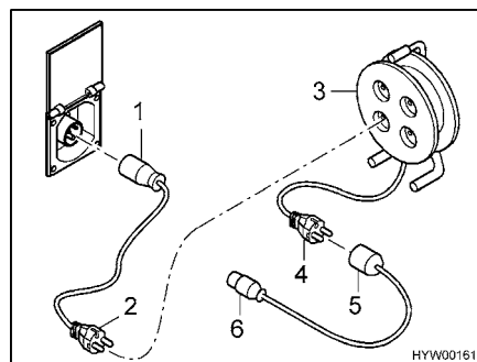
Afb. 136 Aansluitmogelijkheden 230-V-aansluiting
