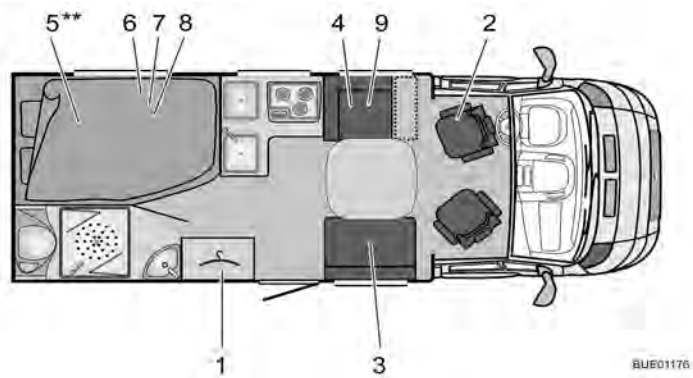
Afb. 269 Plattegrond T 580 Nexxo
