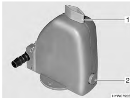
Afb. 177 Veiligheids-/aftapventiel van de boiler
