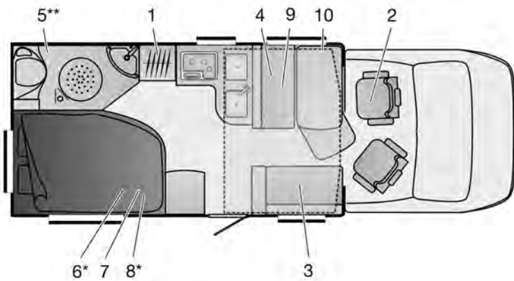
Afb. 274 Plattegrond IT 664 Ixeo
