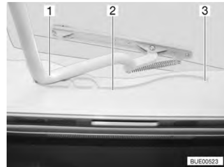
Afb. 74 Heki-dakluik, geleiding
