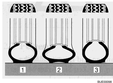
Afb. 48 Draagvlak van de band
