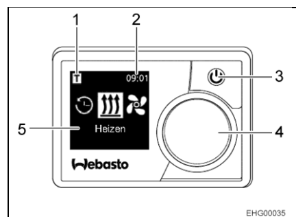
Afb. 38 Bedieningspaneel
