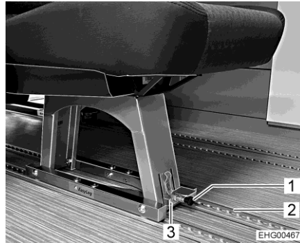
Afb. 3 Aparte zitting (vergrendeld)
