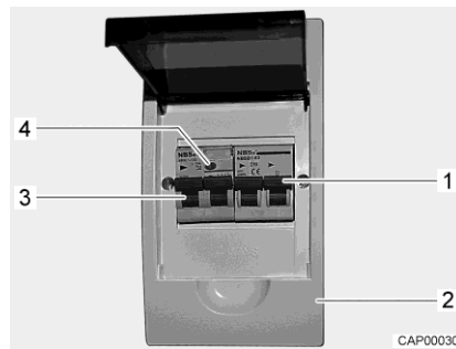
Afb. 32 Beveiligingsautomaat en FI-schakelaar (230-V-zekeringenkast)
