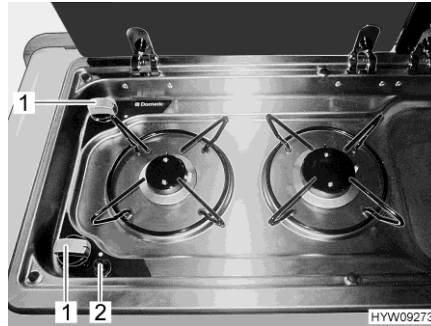
Afb. 39 Gaskooktoestel
