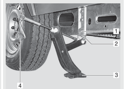
Afb. 224: Wagenkrik, AL-KO
