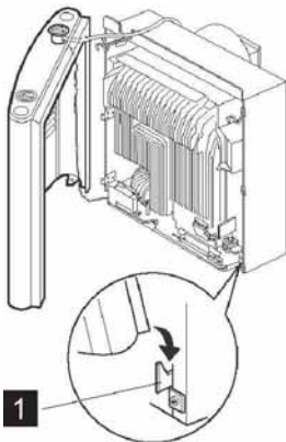
Afb. 134: bekleding van verwarming opengedraaid
