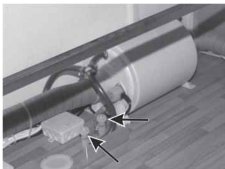
Afb. 99: TRUMA-therme en wateraftapkranen
