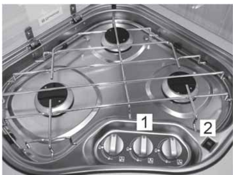
Afb. 206: Gaskomfoor
