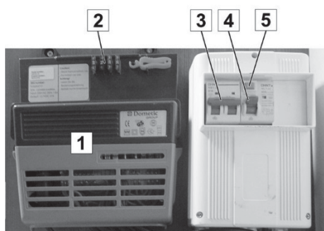
Afb. 61: Omvormer (netvoeding) (1) en zekeringautomaten
