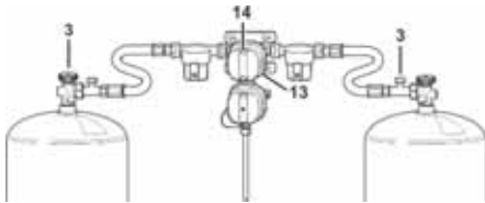
Afb. 120: Gasdrukregelset
