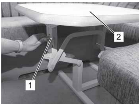
Afb. 181: tafel met heftafeldraagconstructie
