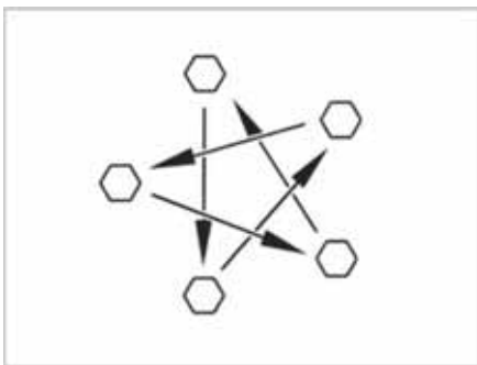
Afb. 220: Wielmoeren of wielschroeven kruisgewijs aandraaien
