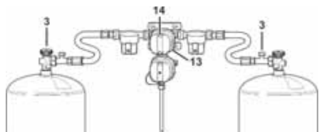
Afb. 117: Gasdrukregelset
