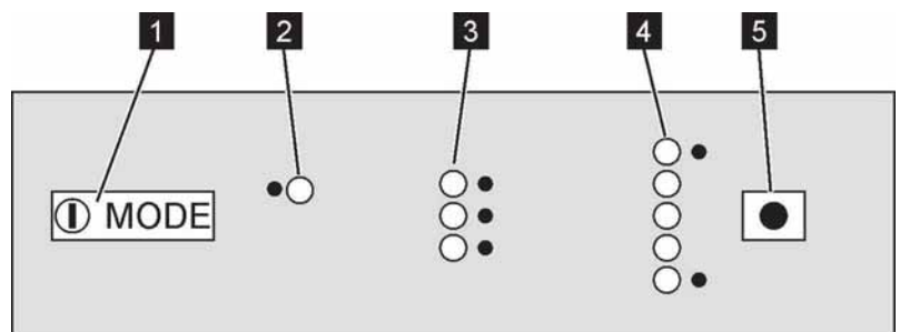
Afb. 217: Besturingselementen op de koelkast met automatische ontsteking
