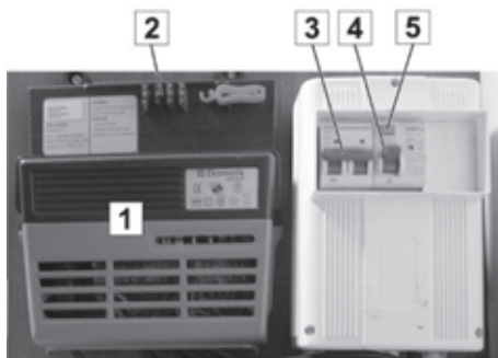
Fig. 58: Convertidor (equipo de red) (1) y fusibles automáticos
