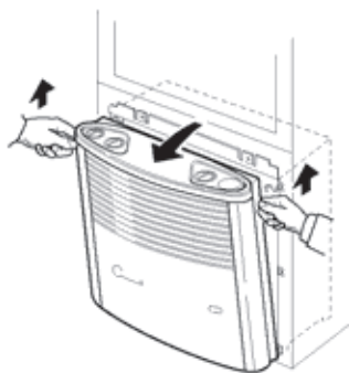
Fig. 115: Levantar el revestimiento de la calefacción
