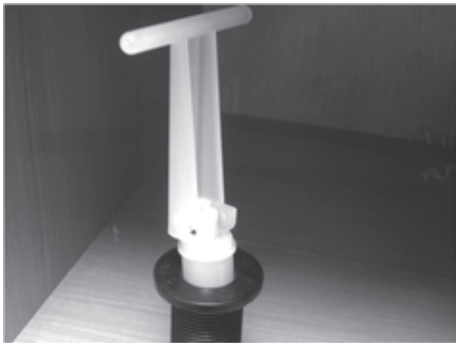
Fig. 92: Tapón de cierre en el depósito de agua limpia, abierto (palanca basculante en posición vertical)
