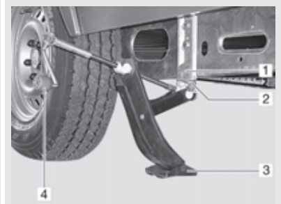
Fig. 150: Gato elevador AL-KO
