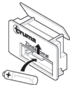
Fig. 117: Cambio de la pila
