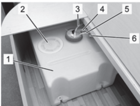
Fig. 81: Depósito de agua limpia, ejemplo
