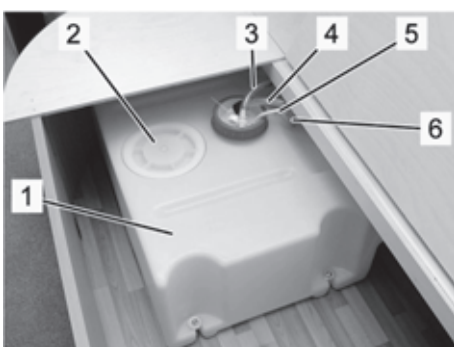
Abb. 81: Frischwassertank, Beispiel
