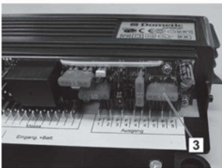
Abb. 60: 12 V-Komplettversorgung
