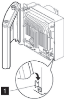
Abb. 116: Heizverkleidung aufgeschwenkt
