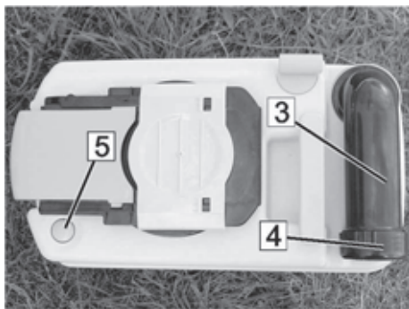
Abb. 134: Fäkalientank entleeren
