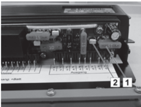
Abb. 59: 12 V-Notbeleuchtung
