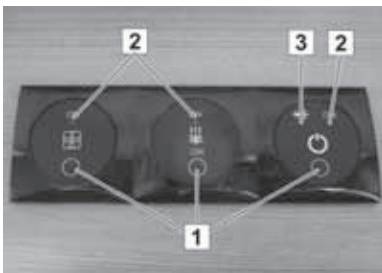
Abb. 62: Anzeigepanel Ladegerät
