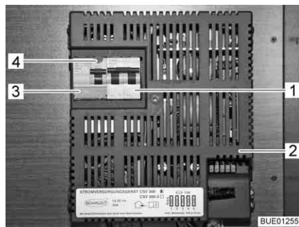
Fig. 125 Scatola dei fusibili a 230 V con interruttore di sicurezza e interruttore automatico FI
