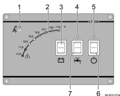
Fig. 122 Pannello di controllo LT 408
