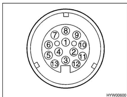
Fig. 132 Figura del contatto della spina a 13 poli
