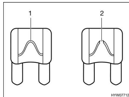
Fig. 127 Fusibile a 12 V
