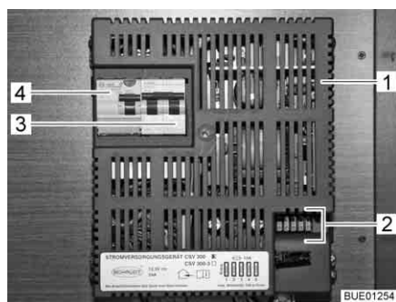
Fig. 120 Apparecchio per l'alimentazione elettrica CSV 300
