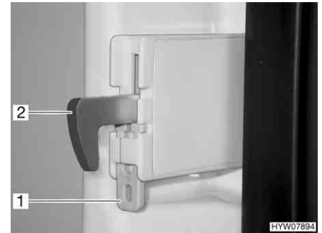
Fig. 174 Fissaggio del gancio di bloccaggio
