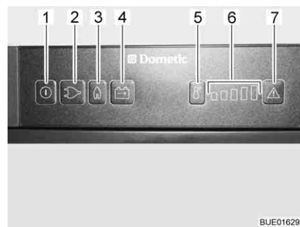
Fig. 171 Elementi di comando per il frigorifero (serie Dometic 8 con SMSE)
