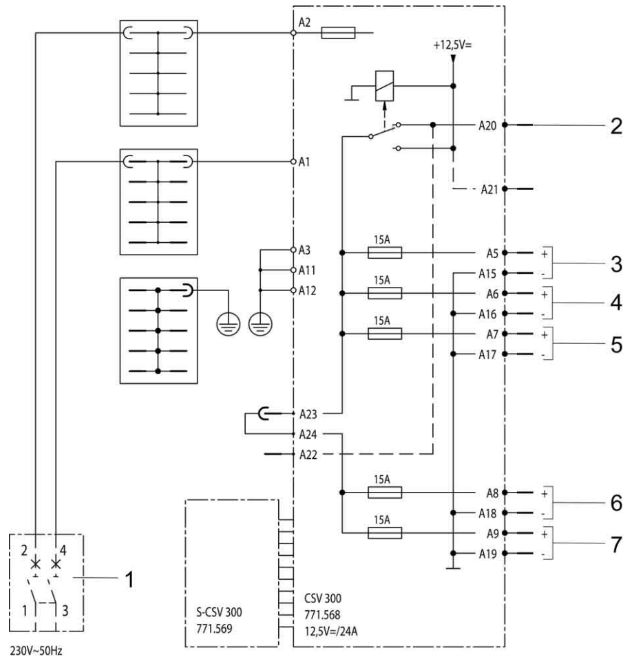
Fig. 136 Schema elettrico interno (CSV 300)
