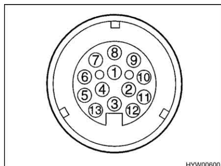
Bild 132 Kontaktbild des dreizehnpoligen Steckers
