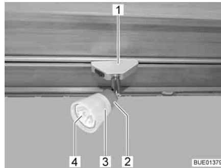
Bild 217 Halogenspotleuchte (verschiebbar)
