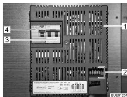
Bild 120 Stromversorgungsgerät CSV 300
