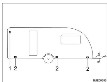
Bild 208 Beleuchtung Seite
