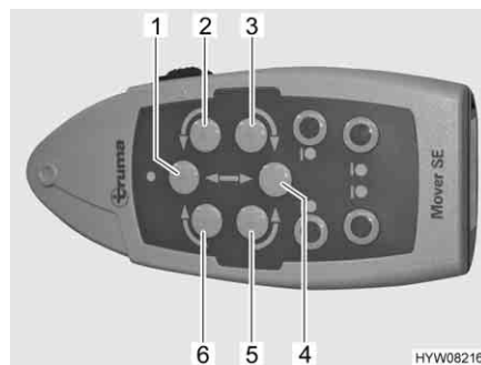
Bild 6 Richtungstasten
