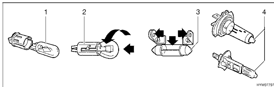
Bild 205 Glühlampen-Typen
