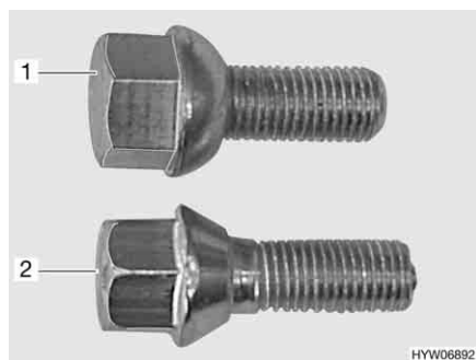
Bild 222 Radschrauben
