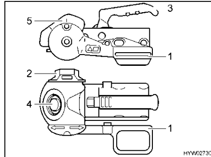
Bild 2 Sicherheitskupplung AKS 1300
