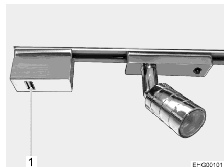
Afb. 188 USB-aansluiting op railsysteem
