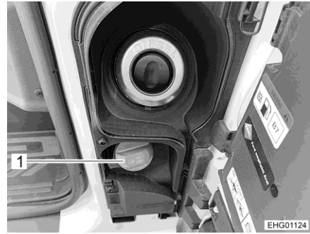
Afb. 45 Vulopening voor AdBlue® (Ford)
