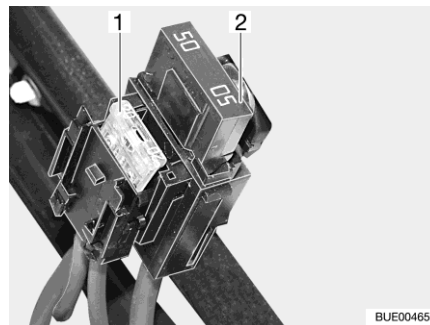
Afb. 197 Zekeringen op de startaccu
