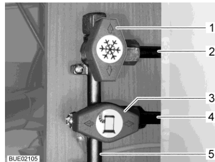
Afb. 180 Stand gasafsluitkranen (voorbeeld)
