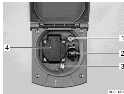
Afb. 204 Buitencontactdoos
