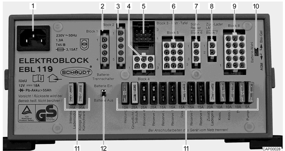
Afb. 190 Elektroblok (EBL 119, voorbeeld)
