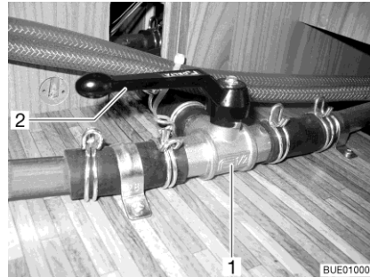
Afb. 217 3-wegventiel
