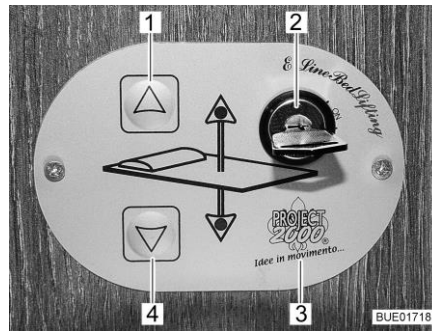
Afb. 143 Bedieningspaneel
