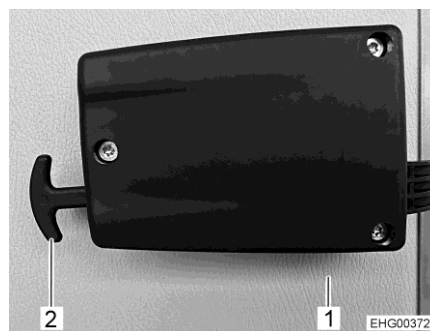
Afb. 61 Noodontgrendeling garage- luik
