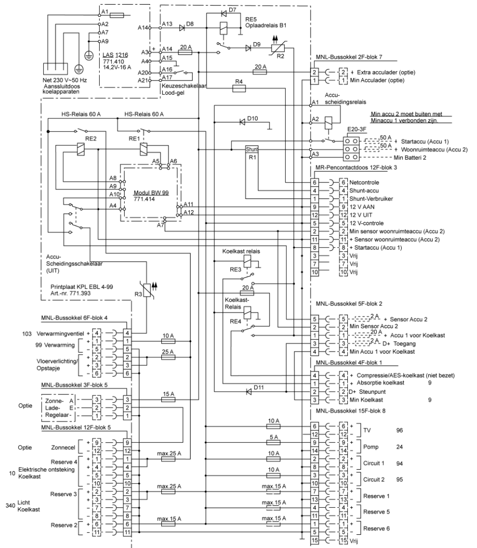
Afb. 207 Stroomschema binnen (EBL 119/EBL 99)
