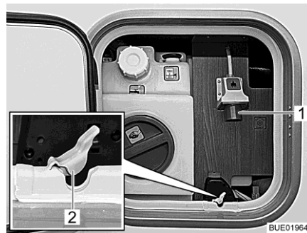
Afb. 194 230-V-aansluiting op het voertuig (met service-unit)
