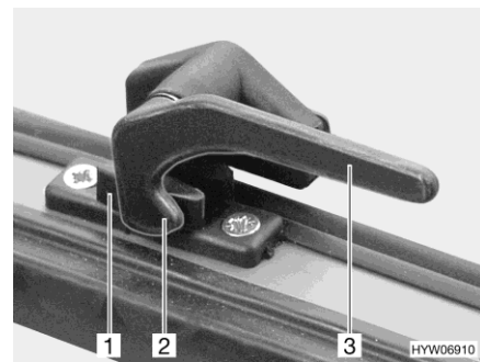
Afb. 119 Vergrendelingshendel in stand "gesloten"
