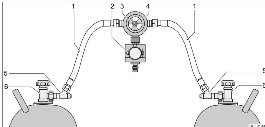
Afb. 20 Gasdrukregelaar met CPU en slangbreukbeveiliging
