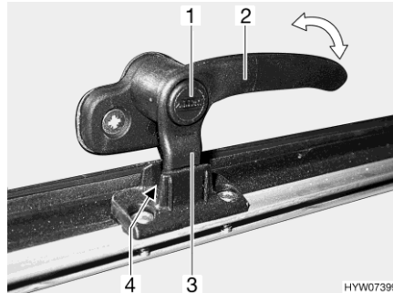
Afb. 121 Vergrendelingshendel met vergrendelingsknop in stand "continue ventilatie"
