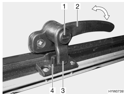
Afb. 118 Vergrendelingshendel met vergrendelingsknop in stand "gesloten"
