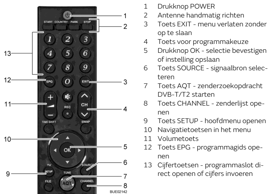
Afb. 50 Afstandsbediening
