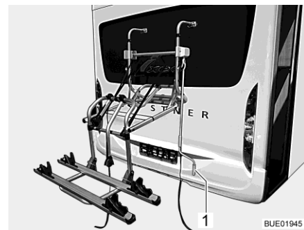
Afb. 5 Fietsenrek, neergelaten
