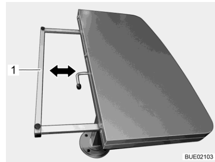
Afb. 130 Tafelblad verkleinen
