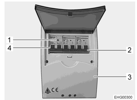
Afb. 193 230-V-zekeringenkast (variant)
