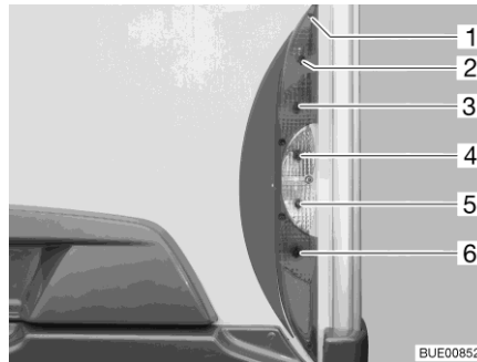
Afb. 289 Verlichting achter
