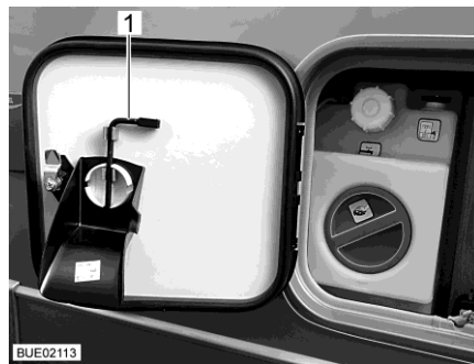
Afb. 263 Serviceluik met vierkantsleutel
