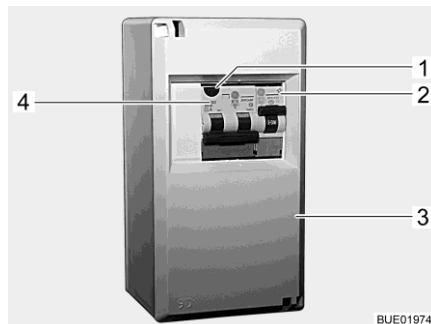
Afb. 202 230-V-zekeringenkast
