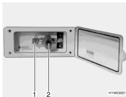
Afb. 181 Externe gasaansluiting (gasafsluitkraan gesloten)
