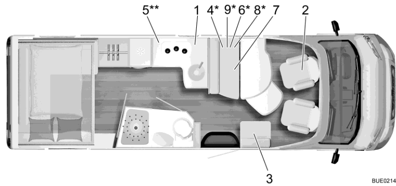
Afb. 321 Plattegrond IT 744
