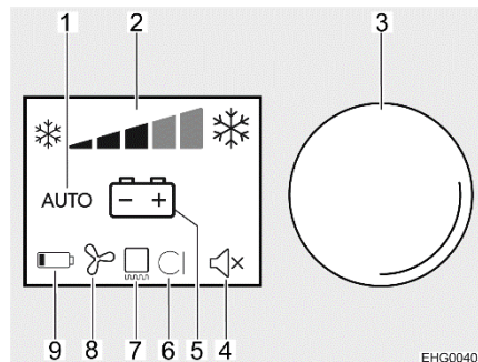
Afb. 240 TFT-display
