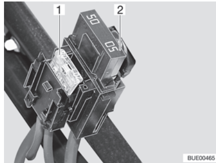
Fig. 124 Fusibles en la batería del motor de arranque
