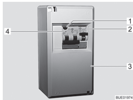
Fig. 121 Caja de fusibles de 230 V con interruptor de protección de línea e interruptor FI
