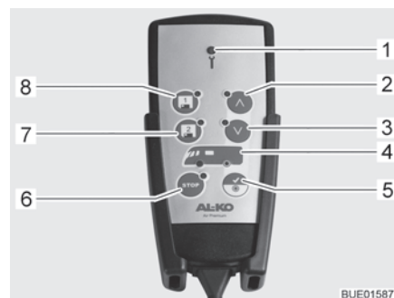
Fig. 15 Mando a distancia
