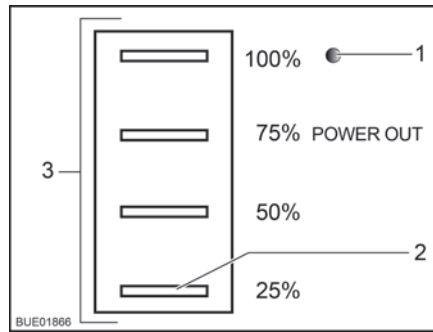
Fig. 120 Indicador de estado del regulador de carga solar
