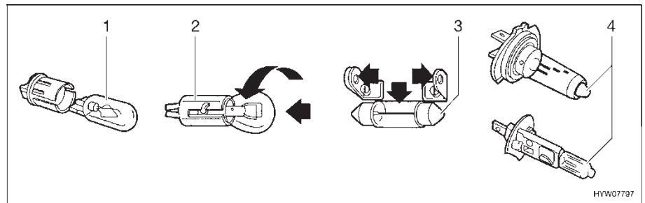
Fig. 186 Tipos de bombilla
