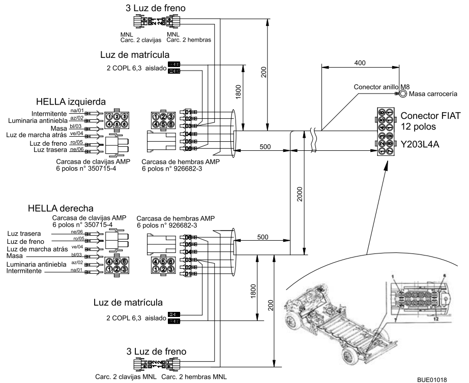
Fig. 133 Esquema de circuitos exterior
