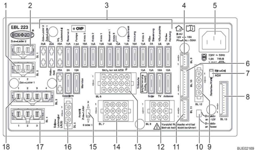
Fig. 118 Bloque eléctrico (EBL 223)
