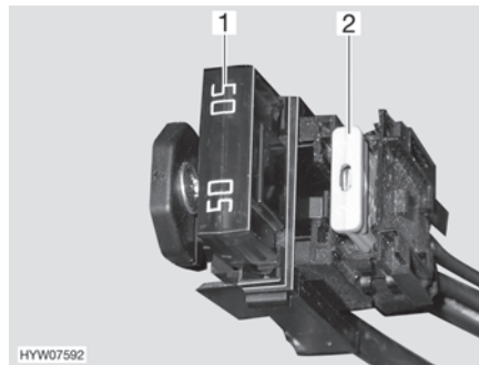
Fig. 125 Fusibles en la batería del habitáculo
