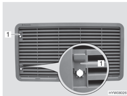
Fig. 155 Rejilla de ventilación del frigorífico (con corredera)
