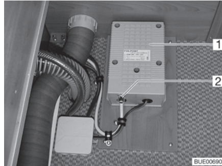
Fig. 145 Transformador para calentamiento eléctrico del piso
