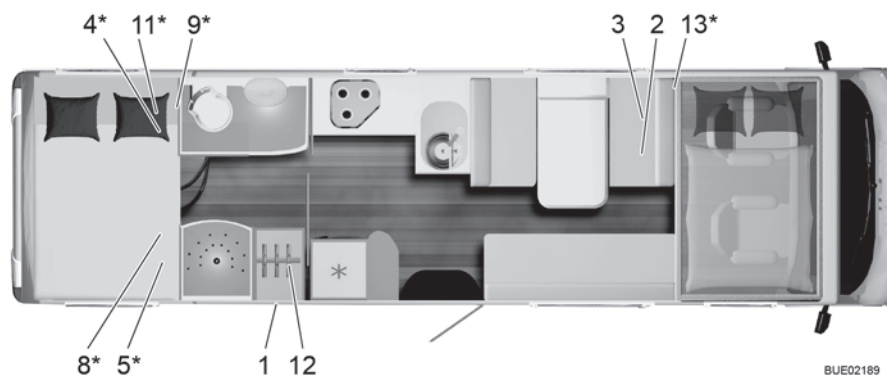
Fig. 202 Esquema A 747-2 G
