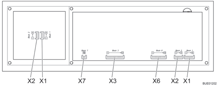
Fig. 132 Diagrama de bloques del panel (LT 511)
