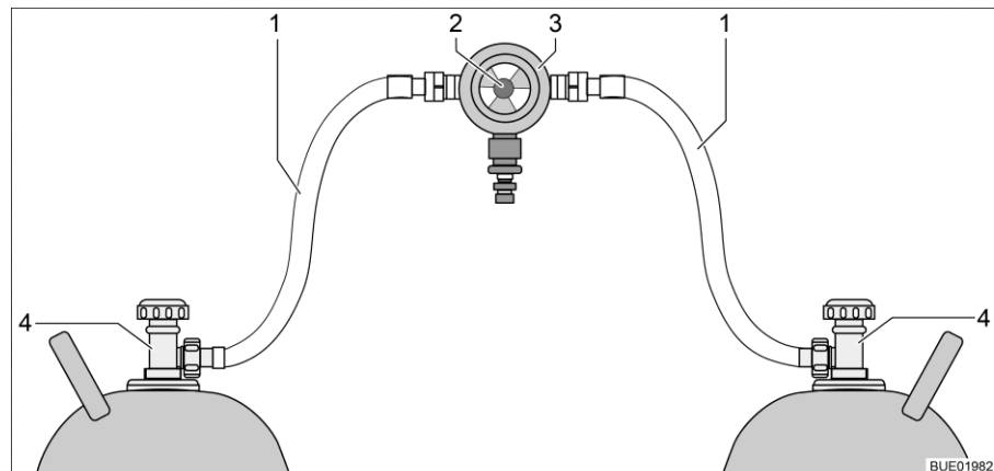
Afb. 173 Omschakelinstallatie voor gasflessen
