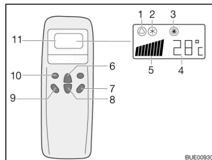
Afb. 231 Afstandsbediening
