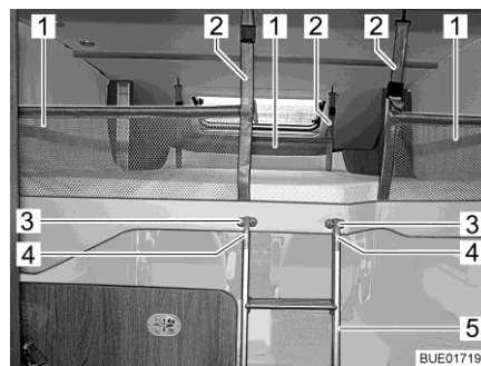
Afb. 138 Hefbed met gespannen veiligheidsnet
