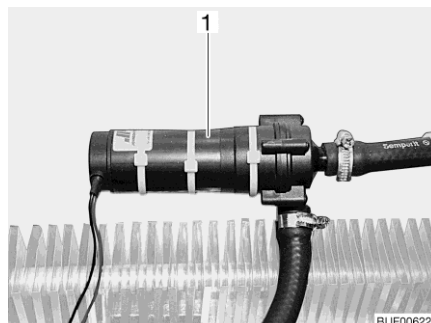
Afb. 221 Extra circulatiepomp
