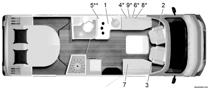
Afb. 320 Plattegrond Lyseo TD 736
