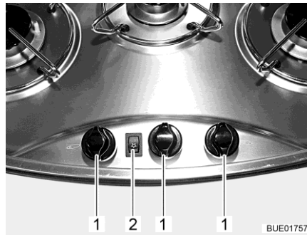
Afb. 234 Bedieningselementen voor gaskooktoestel
