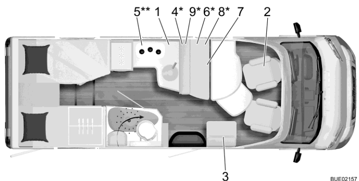
Afb. 314 Plattegrond Lyseo TD 690
