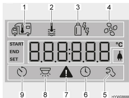
Afb. 213 Display (bedieningspaneel)
