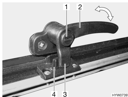
Afb. 113 Vergrendelingshendel met vergrendelingsknop in stand "gesloten"
