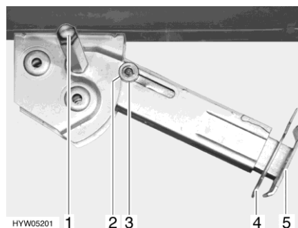
Afb. 41 Hefsteun
