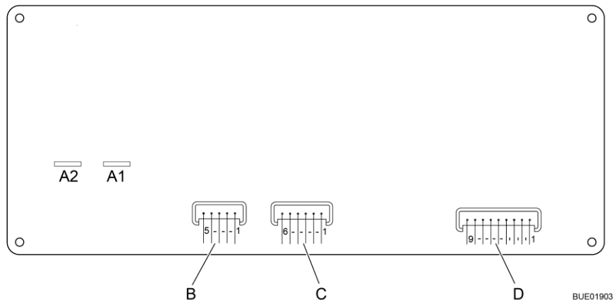
Afb. 206 Aansluitschema, paneel (LT 96)
