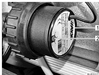
Afb. 218 Toerentalverlaging
