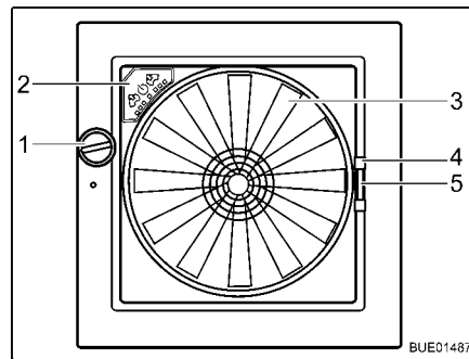
Afb. 111 Dakluik Omni-Vent
