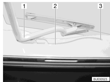
Afb. 108 Geleiding (Heki-dakluik)
