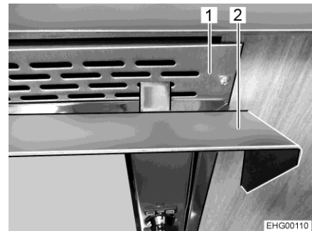
Afb. 237 Hitteschermin (ingehangen)
