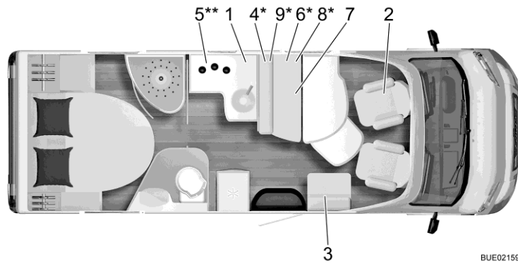
Afb. 315 Plattegrond Lyseo TD 700
