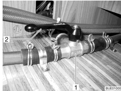
Afb. 219 3-wegventiel
