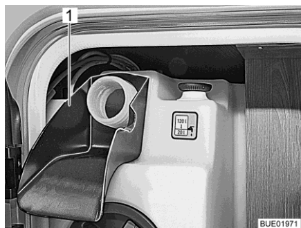
Afb. 264 Vulhulp
