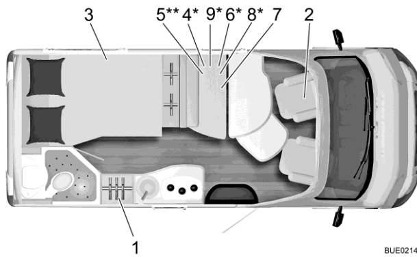
Afb. 325 Plattegrond Nexxo Time T 569
