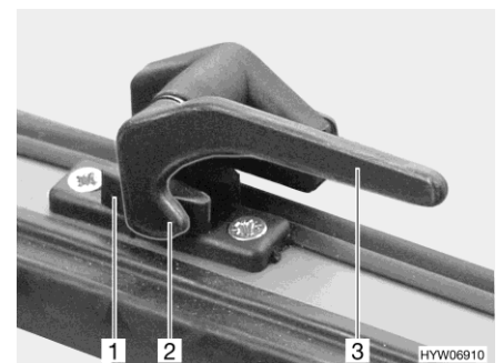
Afb. 114 Vergrendelingshendel in stand "gesloten"
