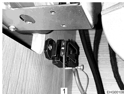
Afb. 199 Zekering hefbed (Ixeo T)
