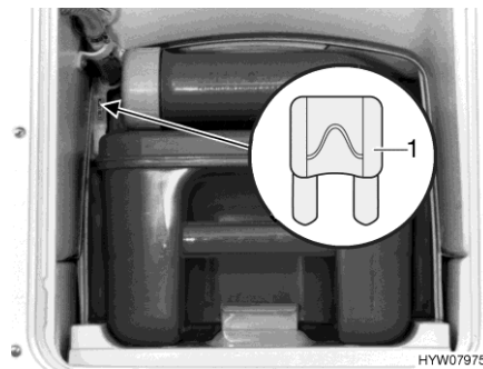
Afb. 192 Zekering van het Thetford-toilet
