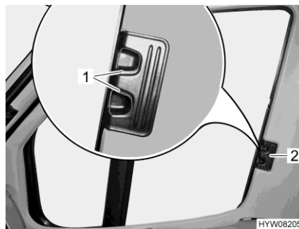
Afb. 102 Vouwverduistering (bestuurders-/passagiersraam)
