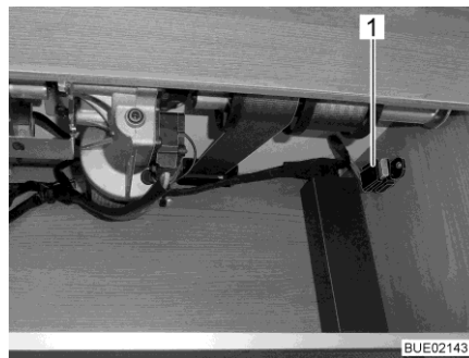
Afb. 149 Zekering
