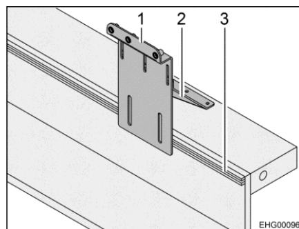
Afb. 1 Reservewielhouder (aan sjoornail)
