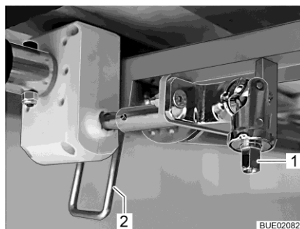
Afb. 132 Hoogte-verstelling
