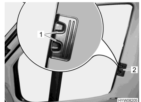
Afb. 38 Vouwverduistering voor bestuurders-/passagiersraam
