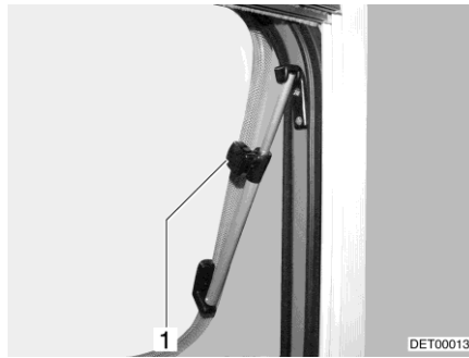
Afb. 115 Dakluik met draaibare uitzetters, geopend
