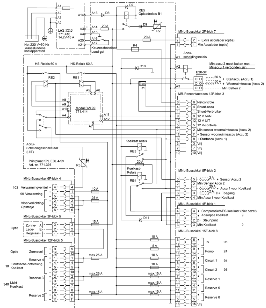
Afb. 204 Stroomschema binnen (EBL 119)
