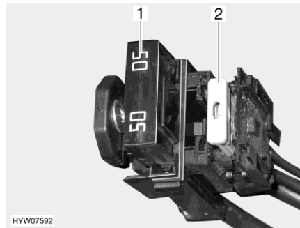
Afb. 191 Zekeringen (woonruimteaccu)
