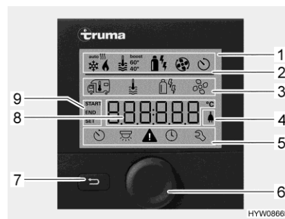
Afb. 212 Bedieningspaneel met aanduidingen
