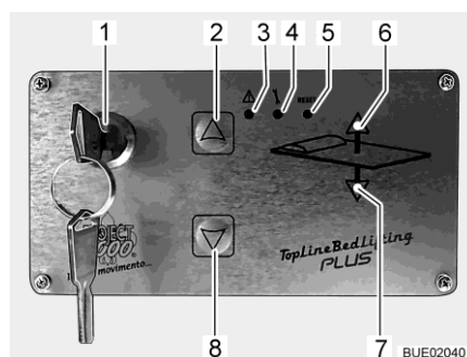
Afb. 134 Bedieningsgedeelte
