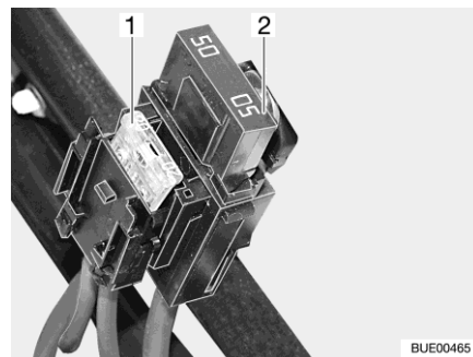
Afb. 190 Zekeringen aan de startaccu
