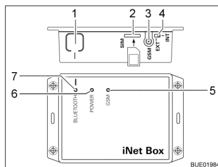
Afb. 233 Truma iNet-Box
