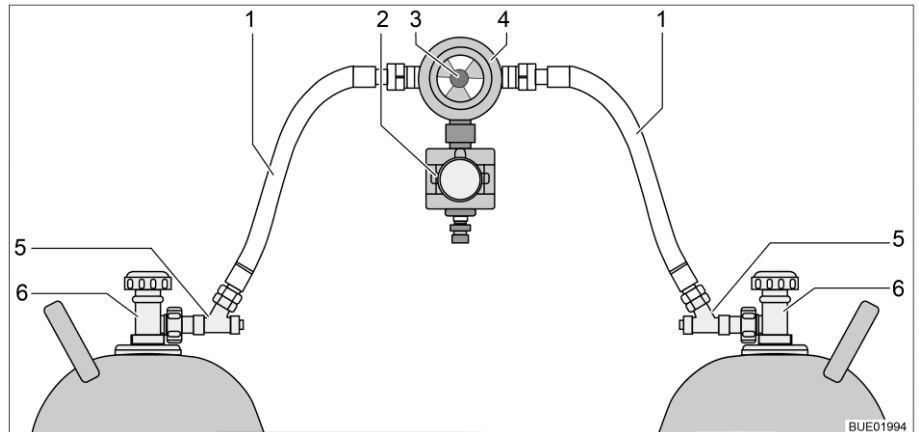
Afb. 20 Gasdrukregelaar met CPU en slangbreukbeveiliging
