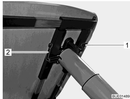
Afb. 124 Verstelling heftafel
