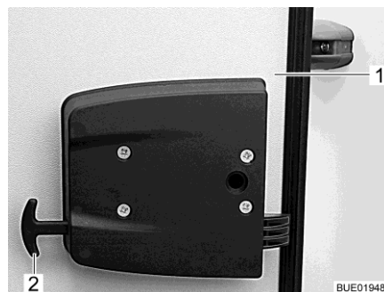
Afb. 55 Noodontgrendeling garage- luik
