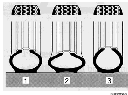
Afb. 311 Draagvlak van de band
