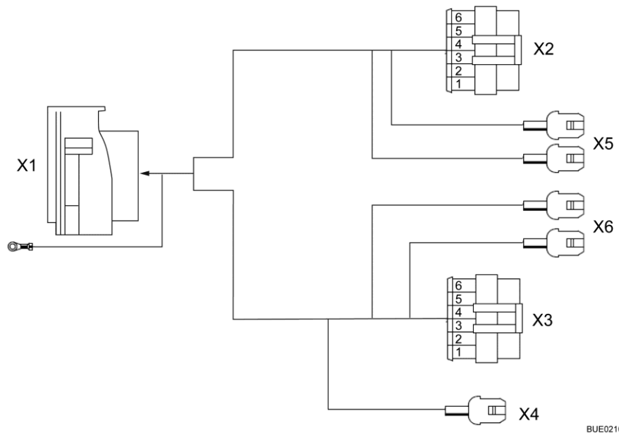
Afb. 208 Stroomschema buiten
