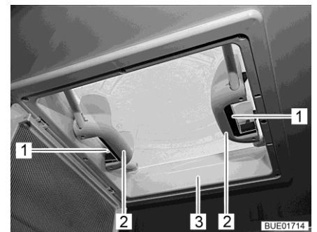
Afb. 105 Grepen met kliksluitingen
