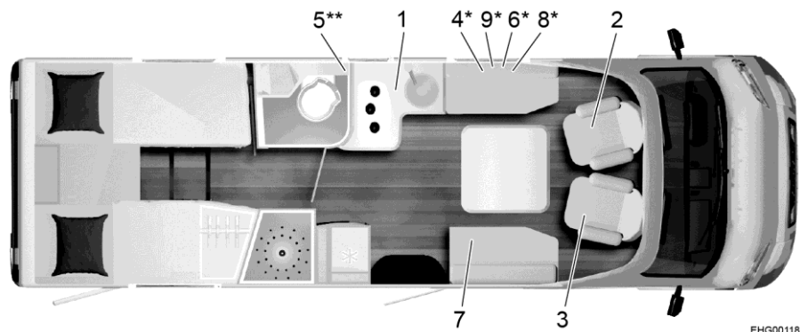
Afb. 317 Plattegrond Lyseo TD 727
