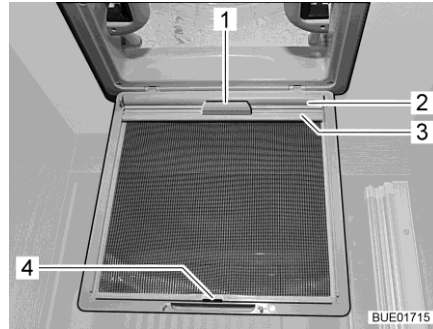
Afb. 106 Verduisteringsrollo (dakluik)
